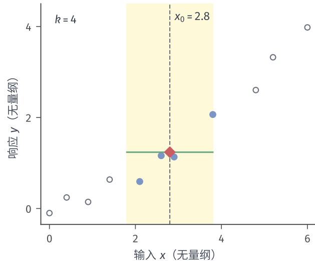
(a) k -NN: 邻域平均
