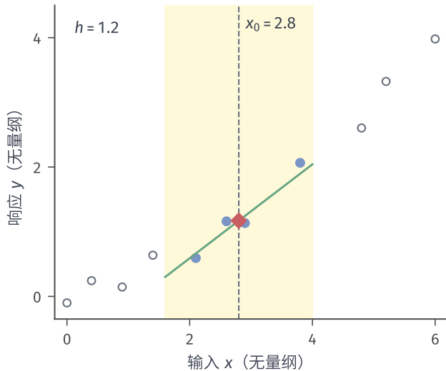
(b) LOESS: 局部直线
