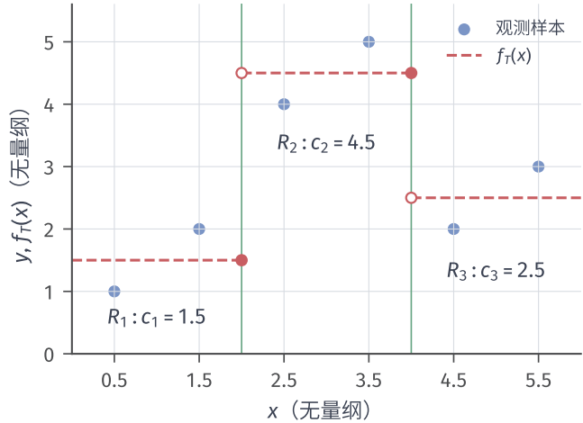
(b) 分段常数预测
