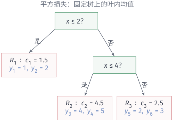
(a) 给定阈值树
