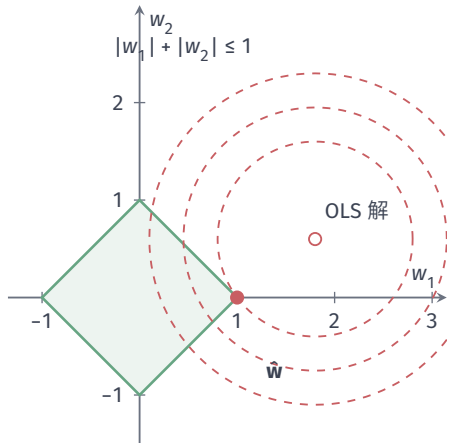
(b) Lasso：菱形约束
