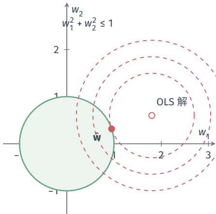
(a) 岭：圆形约束
