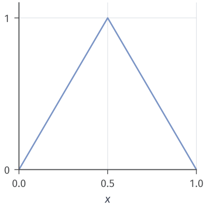
T_1(x) · 2 个线性区间
