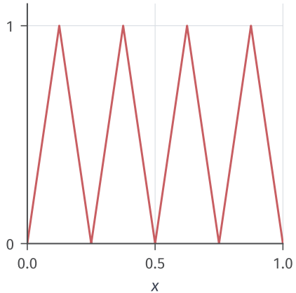
T_3(x) · 8 个线性区间
