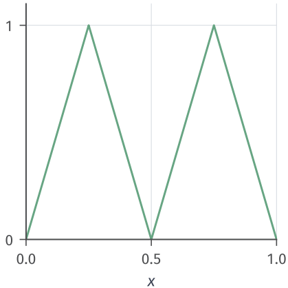
T_2(x) · 4 个线性区间
