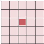
5 \times 5 感受野
