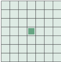
7 \times 7 感受野
