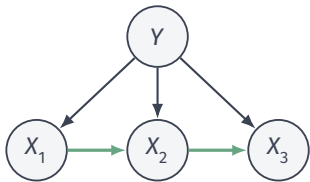
树增强朴素贝叶斯
