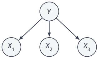
朴素贝叶斯
