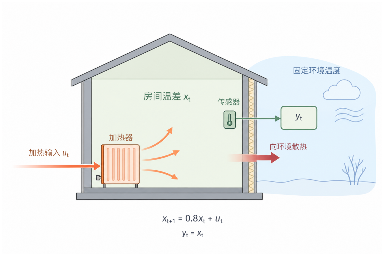
图 13.1 温度模型中的状态、输入与输出。环境温度固定时， x_t 表示房间相对环境的温差， u_t 表示给定加热输入，传感器在时刻 t 读取 y_t = x_t 。随后按 x_{t+1} = 0.8x_t + u_t 形成下一时刻温差；系数 0.8 表示未加热时保留下来的温差比例。图中没有根据读数选择输入的控制。
