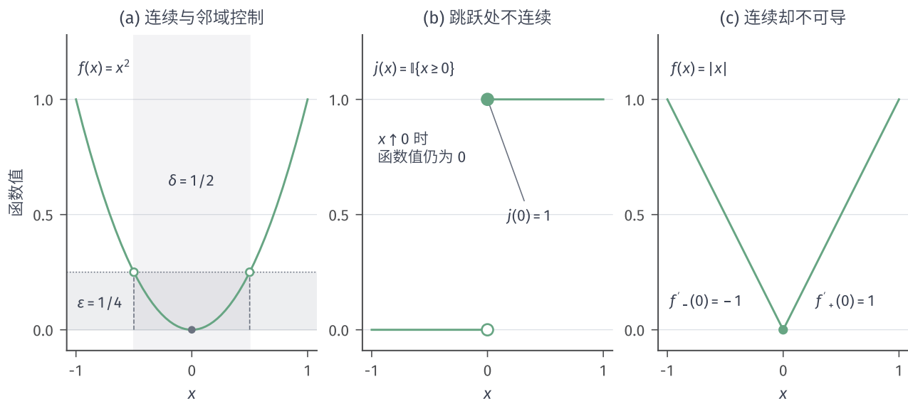
图 3.3 三个不同的局部性质。(a) f(x) = x^2 在 0 处可用 \delta = 1/2 控制 \epsilon = 1/4 : 严格位于输入邻域内的点, 其函数值严格落在输出邻域内。(b) 阶跃函数在 0 的左极限为 0, 取值却为 1, 空心点和实心点区分两者。(c) |x| 在 0 处连续, 但左右导数分别为 -1 和 1 , 不存在共同的双侧导数。图中曲线均为解析教学示例。
