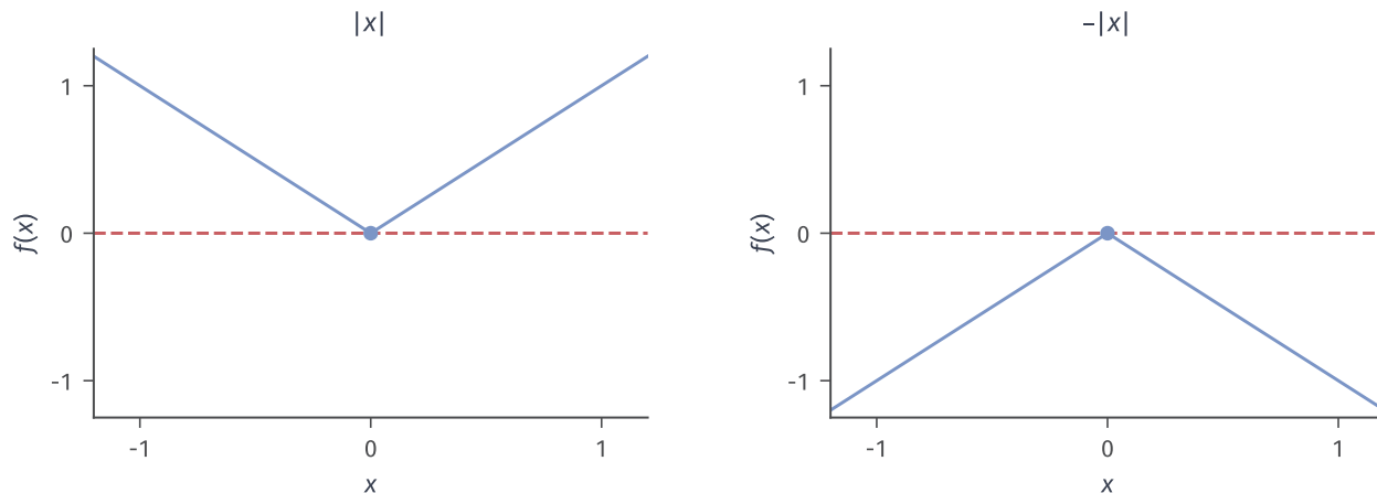
图 3.5 同一广义驻点条件的不同含义。蓝线分别为 |x| 与 -|x| ，红虚线为原点处候选斜率 g = 0 对应的直线。两图在原点的 Clarke 广义梯度均为 [-1, 1] ，却分别形成局部最小点与局部最大点；只有左图红线是全局仿射下界。两图共用坐标尺度，由解析式生成。
