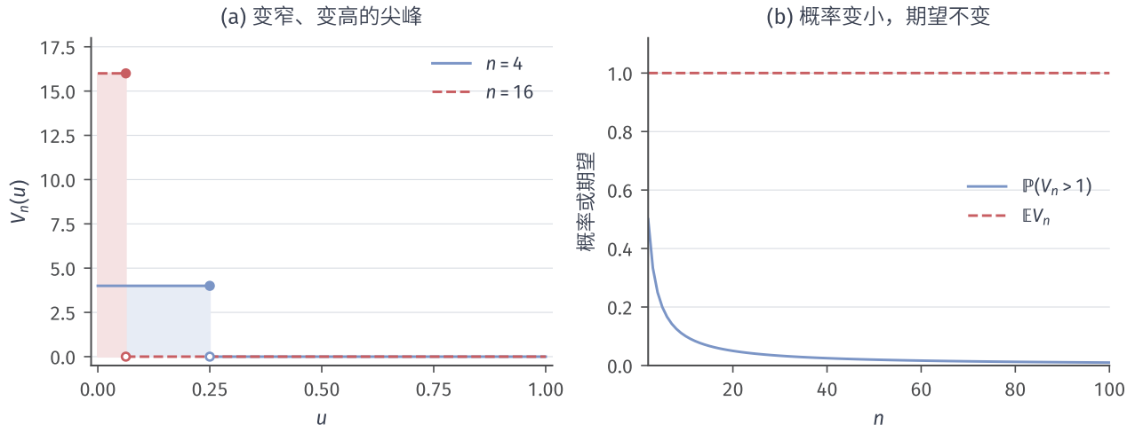
图 10.5 小概率尖峰与期望质量 (解析式教学图)。左图为 V_n(u) = n\mathbb{I}\{u \leq 1/n\} 在 n = 4, 16 时的取值, 均以面积 1 贡献期望; 右图对 n \geq 2 显示 P(V_n > 1) = 1/n 趋于零, 而 \mathbb{E}V_n = 1 不变。基础变量为 U \sim \text{Unif}(0, 1) 。
