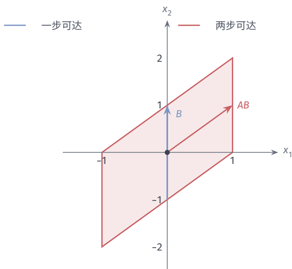
图 14.1 教学系统 \mathbf{A} = \begin{bmatrix} 1 & 1 \\ 0 & 1 \end{bmatrix} 、 \mathbf{B} = (0, 1)^\top 从零出发。蓝色线段为 |u_0| \leq 1 的一步可达集合，红色区域为 |u_0|, |u_1| \leq 1 的两步可达集合；箭头为 \mathbf{B} 与 \mathbf{AB} 。幅值限制用于显示可达区域，不属于无约束可控性秩判据的假设。
