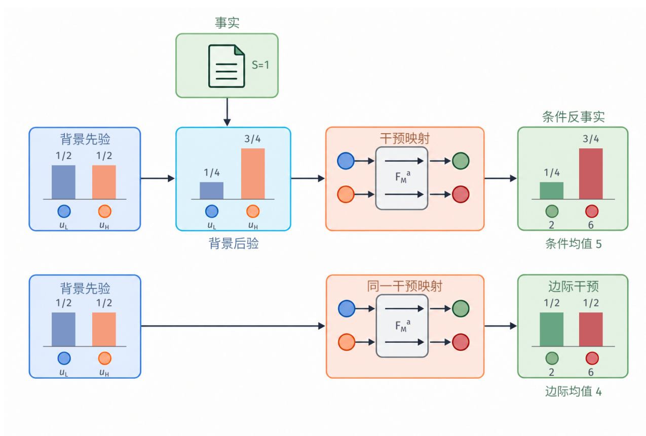
图 12.1 同一行动映射下的条件反事实与总体干预。背景 u_L, u_H 的先验概率各为 1/2 ，事实 S=1 将两者的后验概率更新为 1/4, 3/4 ；行动映射分别给出结果 2, 6。保留后验得到条件均值 5，沿用先验得到总体干预均值 4。概率柱使用共同的零基线与比例尺；溯因是给定的模型内的条件化，不证明结构假设本身有效。
