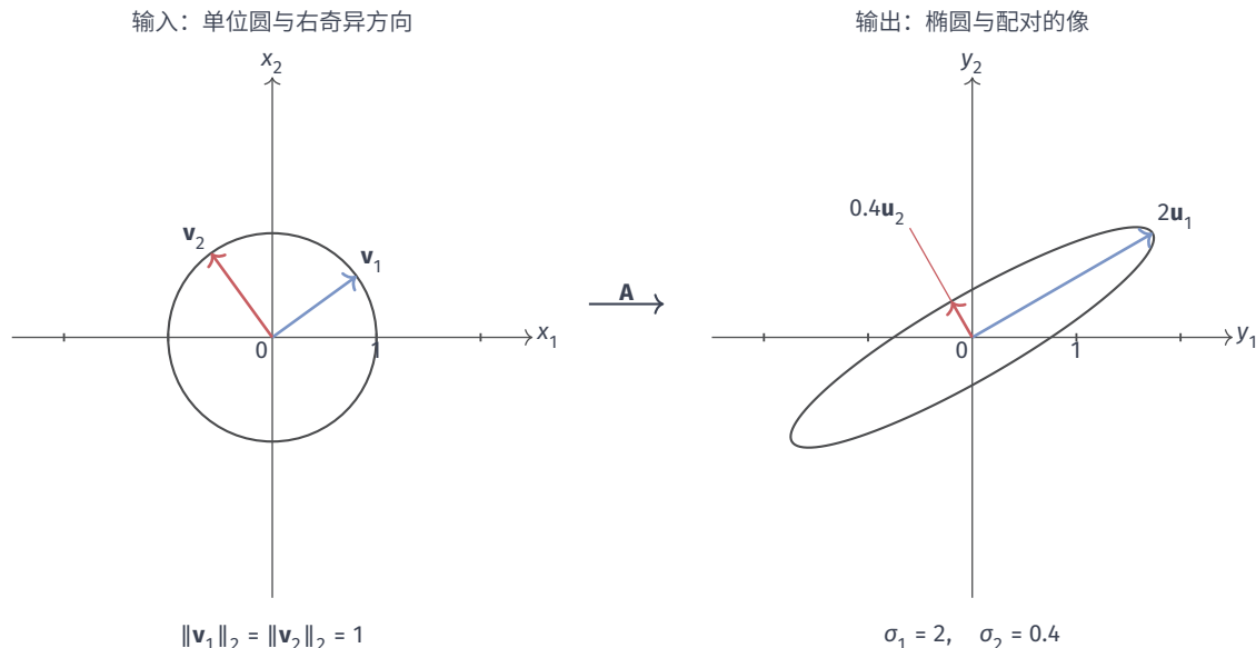
图 6.6 矩阵 A = R(\pi/6) \text{diag}(2, 0.4) R(\pi/5)^T 将单位圆变为椭圆。蓝、红箭头分别标出右奇异方向 v_i 及其像 \sigma_i u_i ；两侧坐标比例相同。奇异值决定长度变化，左右方向可以不同，因而这不是沿特征方向的空间缩放。图为教学构造。
