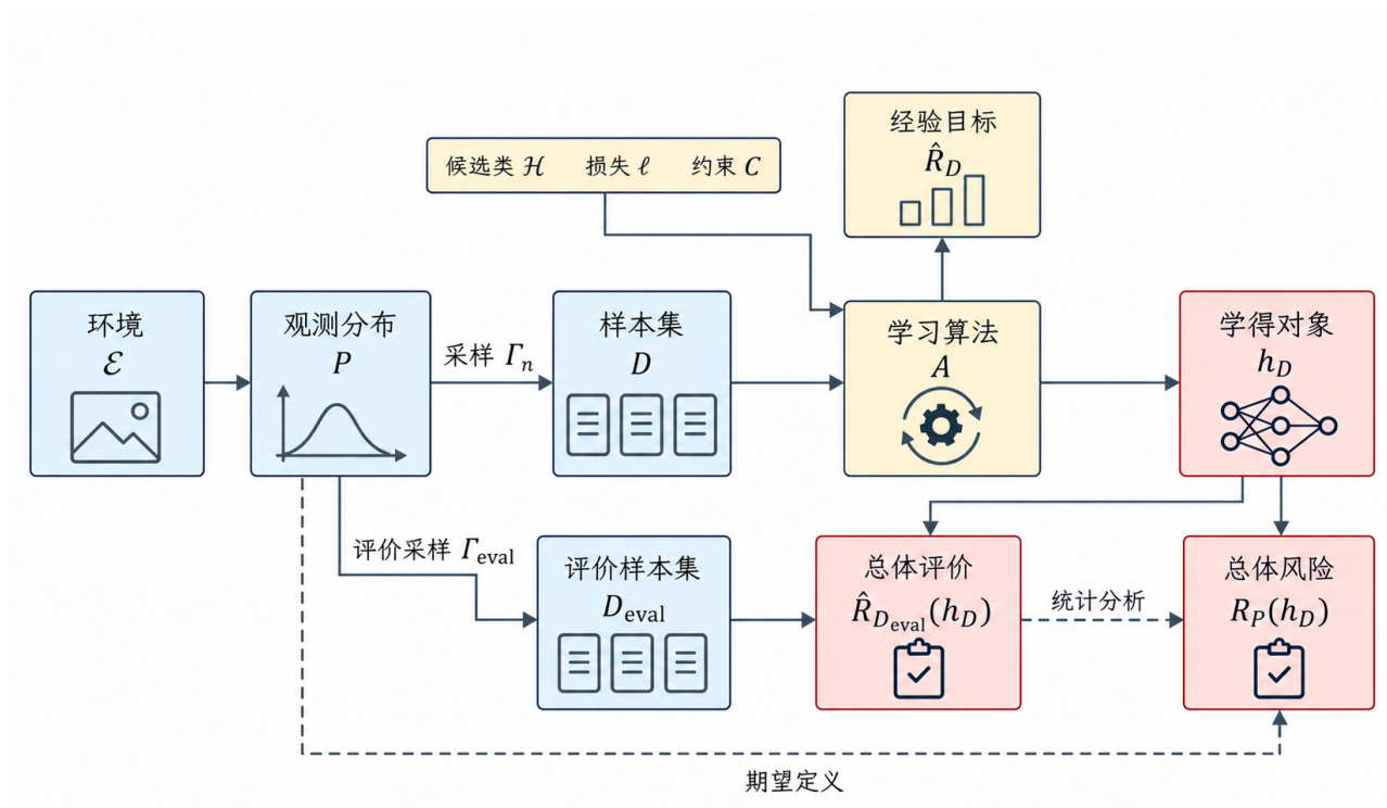
图 17.1 静态学习的共同流程。学习算法接收样本集和候选类、损失、约束，产出经验目标与学得对象。独立评价样本与学得对象共同形成样本上的总体评价，再通过统计分析联系真正的总体风险；分布到风险的虚线表示期望定义。
