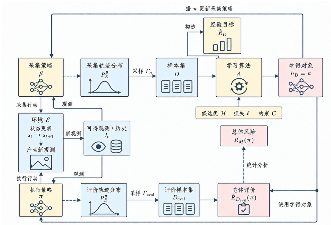
图 17.2 交互学习保留静态流程的采样、学习与评价环节。上方用 \beta 采集并学习，下方部署学得策略 \pi 并采样评价。中间只有一个共享环境：行动更新内部状态，新观测进入 I_t ，两种策略都从可得信息选择行动。它们表示不同运行阶段，不同时控制同一次行动。总体评价是有限轨迹样本的估计，总体风险是它所联系的理论目标；在线更新时可据 \pi 构造下一轮 \beta 。
