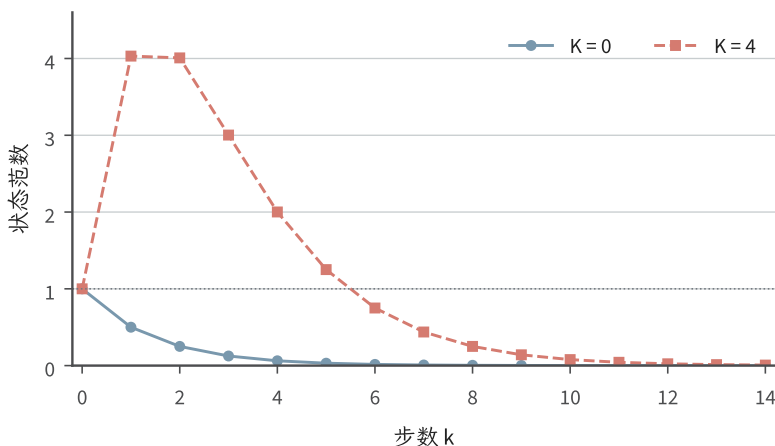
图 13.2 同谱系统的不同瞬态. 初值均为 (0, 1)^T , 蓝色圆点取 K = 0 , 红色方点取 K = 4 , 谱半径均为 1/2 . 后者前两步范数约为 4.03、4.01, 随后才趋零; 灰线为初始范数 1. 长期衰减不等于每一步都收缩.
