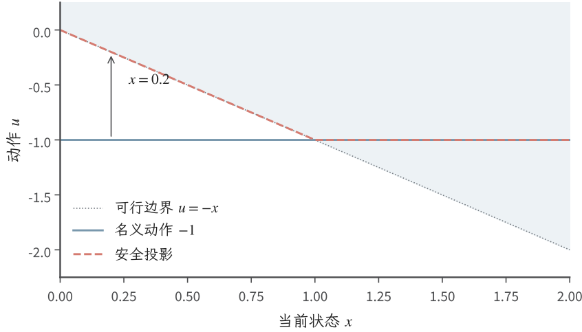
图 14.4 教学积分器 \dot{x}_t = u_t 、安全集合 x \geq 0 及 \alpha(h) = h 。灰色虚线 u = -x 上方为允许动作；蓝色实线为名义动作 u = -1 ，红色虚线为投影 u^* = \max\{-1, -x\} 。 x \geq 1 处无需修正， x = 0.2 处修正为 -0.2 。图中没有额外执行器限制，不能据此判断有限输入范围下的联合可行性。
