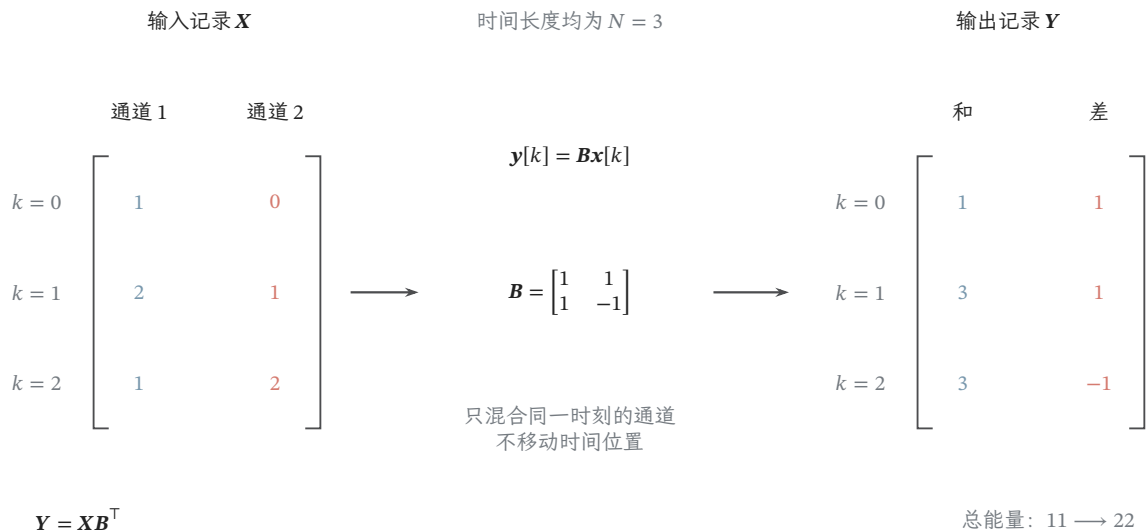
图 8.5 同一双通道三时刻记录的轴与混合。左侧行标记时间、列标记通道；中间矩阵 \mathbf{B} 对每一行对应的同时读数取和与差，右侧时间轴长度仍为 3。通道混合不是时间平移，也不意味着两个输入通道独立；这里只使用当前时刻的值。
