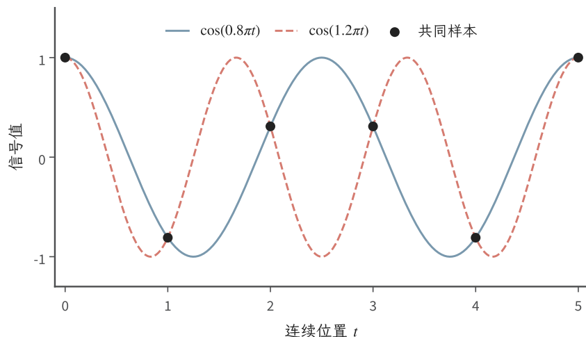
图 8.6 教学构造 f_1(t) = \cos(0.8\pi t) 与 f_2(t) = \cos(1.2\pi t) 。蓝色实线和红色虚线在整数时刻具有共同样本，深灰圆点标出这些观测。图只展示 [0, 5] ，样本相同对所有整数成立；两条纯余弦是功率信号，不属于后文定理中的整轴平方可积信号类。
