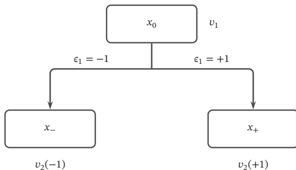
图 5.6 深度为 2 的固定查询树。根查询 x_0 , 左右分支对应 \epsilon_1 = -1 与 +1 ; 各节点旁的 v_1, v_2(\pm 1) 是一棵覆盖中心预先指定的值, 表示近似值而非真实反馈。固定两点输入只观察其中一条路径。
