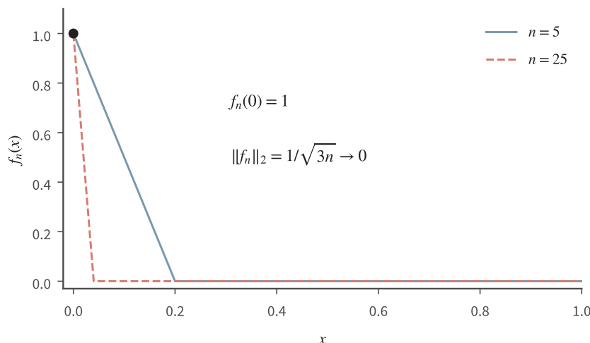
图 5.1 连续尖峰 f_n(x) = \max\{1 - nx, 0\} 在 L^2 范数下趋于零，原点函数值却始终为 1。峰宽分别为 1/5 和 1/25 ；蓝、红线均由解析式生成。整体能量控制不等于稳定的点值控制。
