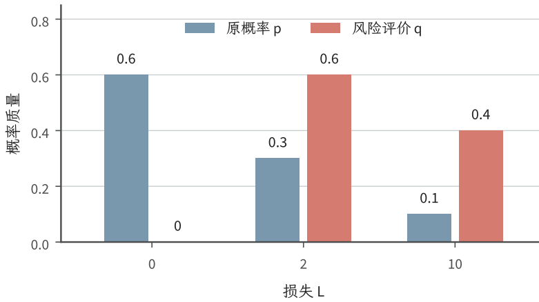
图 15.2 损失 0, 2, 10 的名义概率为 (0.6, 0.3, 0.1) , \text{CVaR}_{0.75} 的约束为 q_i \leq 4p_i 和 \sum_i q_i = 1 。最优重加权 (0, 0.6, 0.4) 的期望为 5.2。蓝色为名义质量, 红色为对偶最优质量; 真实发生概率并未因评价重加权而改变。
