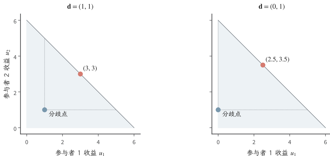
图 16.3 两方协商的教学可行域 u_1, u_2 \geq 0, u_1 + u_2 \leq 6 , 两图坐标一致。蓝点为分歧收益, 红点为相对该分歧点的 Nash 乘积最优解。左图 d = (1, 1) 得到 (3, 3) , 右图 d = (0, 1) 得到 (2.5, 3.5) ; 灰色虚线给出个体可接受的下界。可行总收益没有变化, 变化的是退出时可得到的收益。
