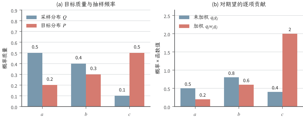
图 10.4 三结果换测度的有限构造。左图比较采样分布 Q 与目标分布 P ，右图比较 q_j g_j 与 q_j w_j g_j = p_j g_j 。各柱从零起画；右图柱高之和分别为 1.7 和 2.8，并非单点概率。
