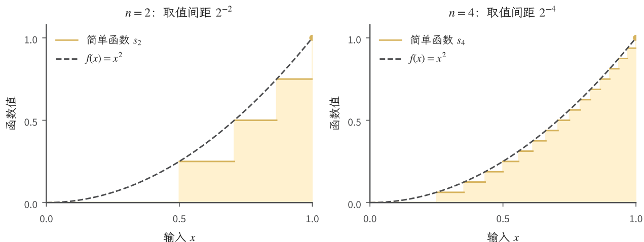
图 3.6 按取值分层的简单函数逼近。两图都使用式 (3.33) 的构造，分别取 n = 2 和 n = 4 ；本例中高度截断不起作用。黄色阶梯下的面积是有限加权和，目标曲线下的面积为 1/3 。两图共用坐标尺度。
