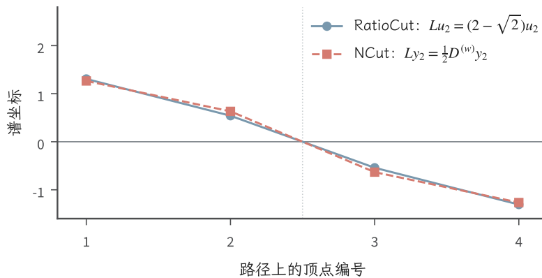
图 9.11 单位权四顶点路径的两种谱方向。蓝实线为组合拉普拉斯第二特征向量，红虚线为度加权广义特征向量，点形也作区分。显示时均按欧氏范数 2 缩放，不替代 NCut 的度加权范数。横轴为四个离散顶点，连线仅引导阅读；竖虚线标出零阈值分割，两种方向虽同号分组，相对幅度并不相同。
