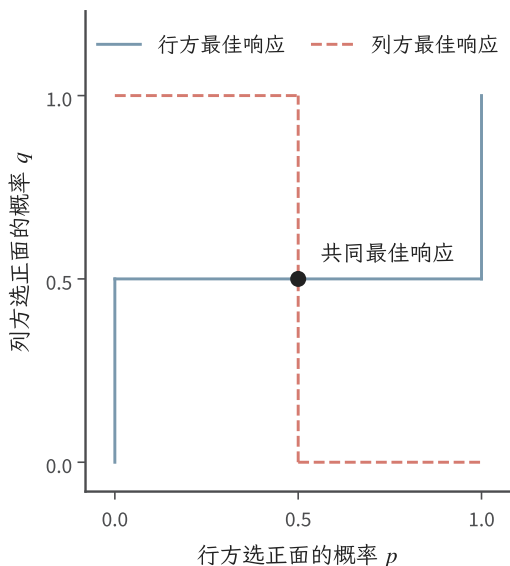
图 16.1 匹配硬币的最佳响应集合。横轴 p 、纵轴 q 分别是两方选 H 的概率。蓝色实线为行方响应，红色虚线为列方响应；在 q = 1/2 处行方允许全部 p ，在 p = 1/2 处列方允许全部 q ，唯一共同点为 (1/2, 1/2) 。这些线段描述允许的响应，不是实际运行的学习轨迹。
