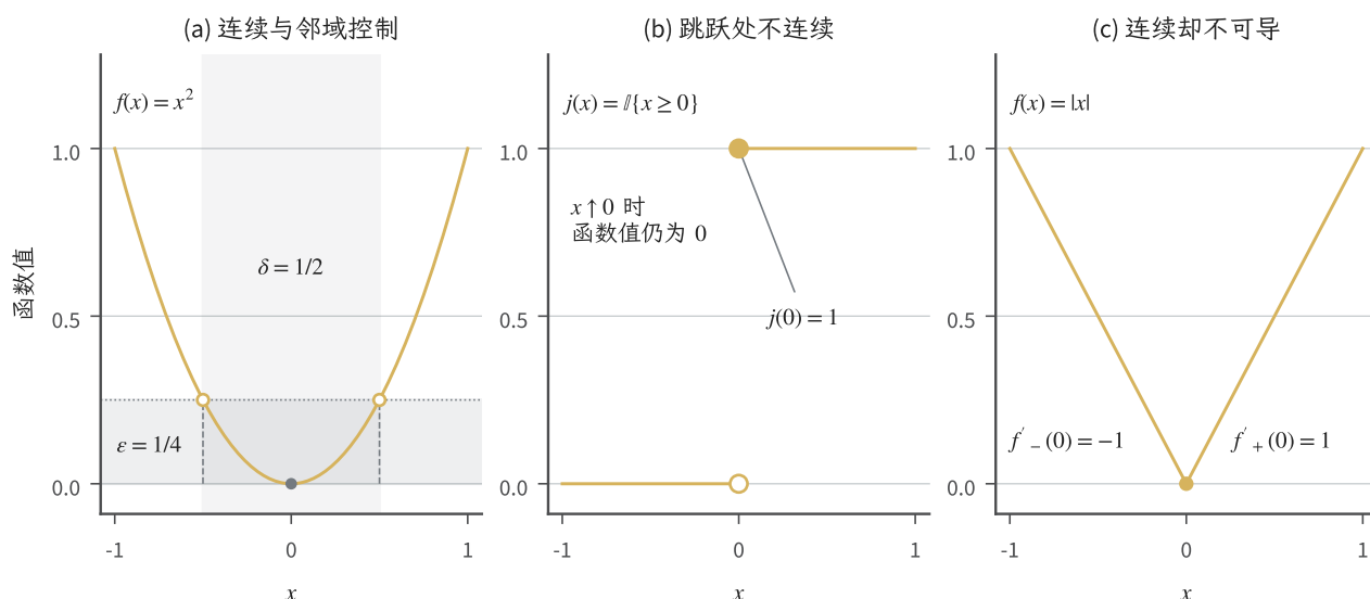
图 3.3 三个不同的局部性质。(a) f(x) = x^2 在 0 处可用 \delta = 1/2 控制 \epsilon = 1/4 : 严格位于输入邻域内的点, 其函数值严格落在输出邻域内。(b) 阶跃函数在 0 的左极限为 0, 取值却为 1, 空心点和实心点区分两者。(c) |x| 在 0 处连续, 但左右导数分别为 -1 和 1 , 不存在共同的双侧导数。图中曲线均为解析教学示例。
