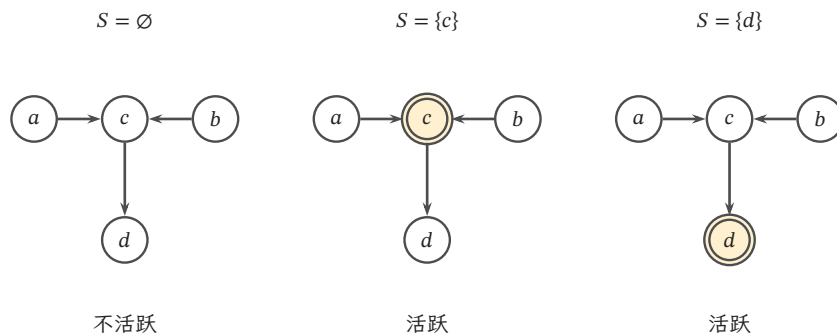
图 9.3 同一底层路径 a - c - b 在三个条件集下的活跃性。箭头及顶点没有改变；空条件集未打开碰撞点，给定碰撞点 c 或其后代 d 都会打开它。双圈表示被给定的顶点，底部文字给出判定。活跃性不是沿箭头从 a 走到 b 的可达性，也不是简单删除条件顶点后的连通性。
