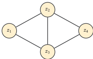
图9.1 由四变量约束的作用域导出的关系图。边表示两个变量共同出现在至少一个约束中；共享顶点集合 \{2, 3\} 连接左右两侧。图没有记录约束的具体真值表，也没有预先指定边长、容量或相似度。
