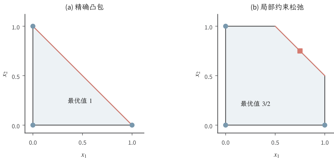
图 4.6 最大化 x_1 + x_2 的两种放宽。左图精确凸包满足 x_1 + x_2 \leq 1 ; 右图局部松弛满足 0 \leq x_i \leq 1 与 x_1 + x_2 \leq 3/2 。实心圆为整数可行点, 方形为右图的分数最优点 (3/4, 3/4) , 粗边标出各自最优面。两图采用相同坐标尺度。
