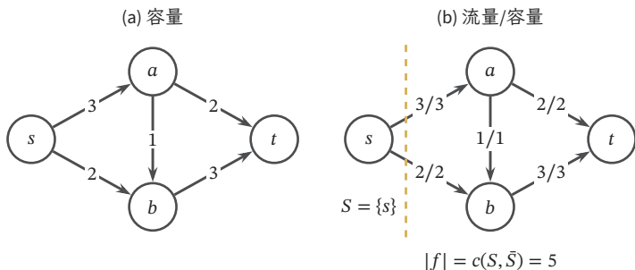
图 9.8 同值流与割构成最优性证书。左图标容量，右图标流量/容量；内部顶点均满足流守恒。黄虚线划出 S = \{s\} ，跨出它的容量为 3 + 2 = 5 ，等于已实现流值。图中画的是原网络弧，未画残量反向弧。
