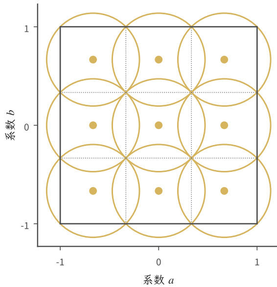
图 5.5 仿射函数族的有限覆盖。方形表示 a, b \in [-1, 1] ，九个实心点是类内代表，圆的半径为 \sqrt{2}/3 。每个小方格都被对应格心的闭球覆盖；圆的重叠与越出方形的部分均不影响覆盖要求。
