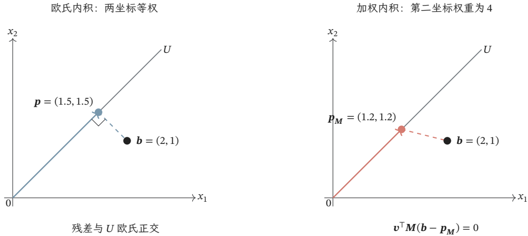
图 6.2 同一目标在同一直线上的欧氏投影与加权投影。实箭头是投影向量，虚线是残差；右图画在普通坐标中，残差不必形成欧氏直角。正交性必须用所选内积判断。
