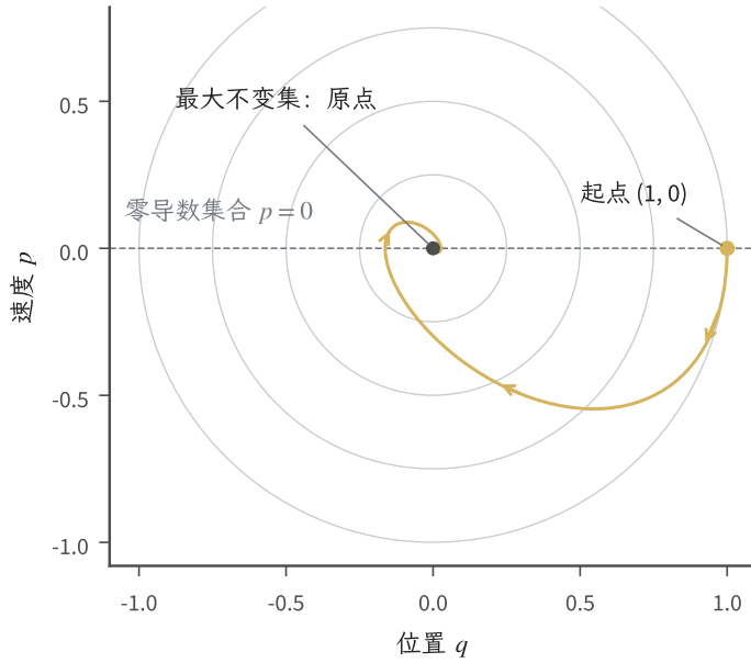
图 13.3 阻尼振子 \dot{q} = p, \dot{p} = -q - p 从 (1,0) 出发的精确轨迹。黄色轨迹覆盖 t = 0 至 12，箭头指示时间；灰色虚线为 \dot{V} = 0 的直线 p = 0 ，浅灰圆为能量参考等值线。起点虽在零导数集合上，初始速度 (0, -1) 却将它带离该集合；能一直留在其中的完整轨迹只有原点。
