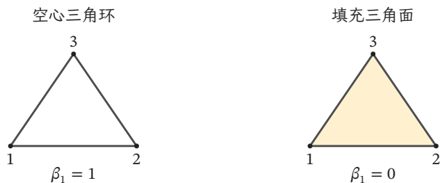
图 7.2 一圈边是否已填充，取决于高阶面而非边图。左侧闭链 c = [1, 2] + [2, 3] - [1, 3] 不是边界；右侧加入 [1, 2, 3] 后有 c = \partial_2[1, 2, 3] 。两者 \beta_0 = 1 ， \beta_1 分别为 1 与 0。图为组合教学示例，不代表某个观测点云的真实拓扑。
