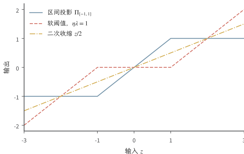
图 4.3 同一输入 z 的三种邻近映射。投影采用 C = [-1, 1] ；软阈值与二次收缩均取 \eta\lambda = 1 ，分别输出 \text{sign}(z)(|z| - 1)_+ 和 z/2 。横轴刻度标出阈值位置，曲线由完整分段解析式生成。
