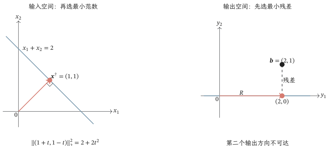
图 6.4 伪逆的两次选择。右图先在可达输出中选择离 \mathbf{b} = (2, 1)^\top 最近的 (2, 0)^\top ；左图再在整条原像直线 x_1 + x_2 = 2 上选择最靠近原点的 (1, 1)^\top 。两图属于不同空间，各自等比例绘制。
