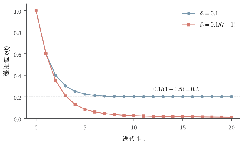
图 3.1 相同初值与收缩系数下的两种递推。蓝线使用持续扰动，红线使用衰减扰动；每个点都是整数步上的精确递推值，图中 e(t) 对应正文的 e^{(t)} ，灰虚线是持续扰动留下的极限 0.2。图为教学构造。
