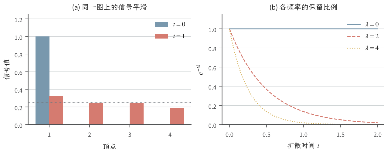
图 9.13 贯穿四顶点图的解析式扩散。左图比较 \mathbf{f}(0) = (1, 0, 0, 0)^\top 与 \mathbf{f}(1) = e^{-L}\mathbf{f}(0) ，灰虚线是最终均值 1/4；右图绘制特征值 0, 2, 4 的保留比例，4 的重数为 2。柱和曲线直接由该图的拉普拉斯计算，不表示实验均值或误差条。
