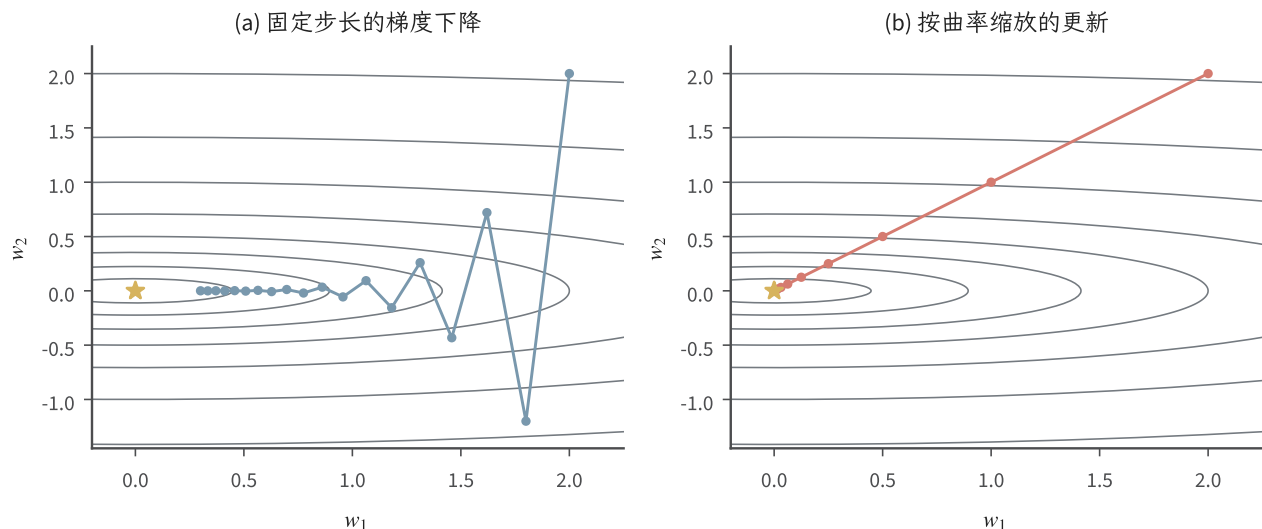
图 4.2 例 4.11 中的精确更新路径。灰线是同一二次目标的等值线，蓝、红圆点分别表示普通更新与预条件更新，黄色星号是最小点。预条件使用了已知曲率，获得和应用这一矩阵的成本仍属于算法代价。
