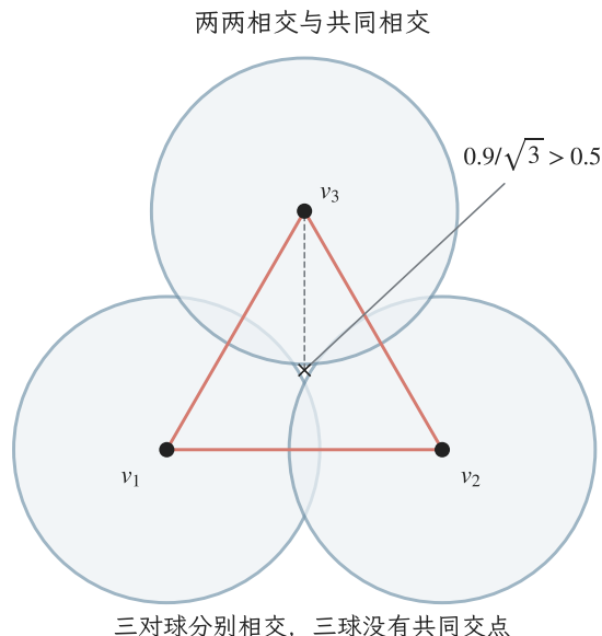
图 7.1 固定同组三点比较共同交集与成对条件。正三角形边长 0.9, \varepsilon = 1 , 蓝色开球半径 0.5; 红色边满足两种构造的连边条件。三球无共同交点, Čech 不含二维面, Rips 含二维面。中心到各顶点的距离为 0.9/\sqrt{3} > 0.5 。圆周只标开球边界, 图为解析教学构造。
