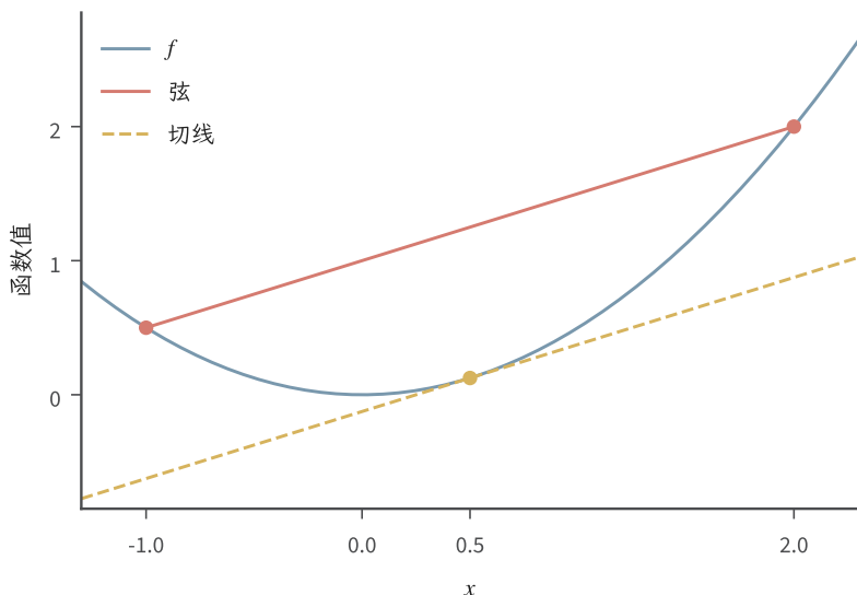
图 4.1 f(x) = x^2/2 的弦与切线。蓝线为函数，红线连接 u = -1 与 v = 2 的函数值，在这两个输入之间给出弦上界；黄虚线是在 x_0 = 1/2 处的一阶仿射下界，适用于整个实线。红线的上界只在其端点之间使用，切线下界来自凸性。图为解析教学示例。
