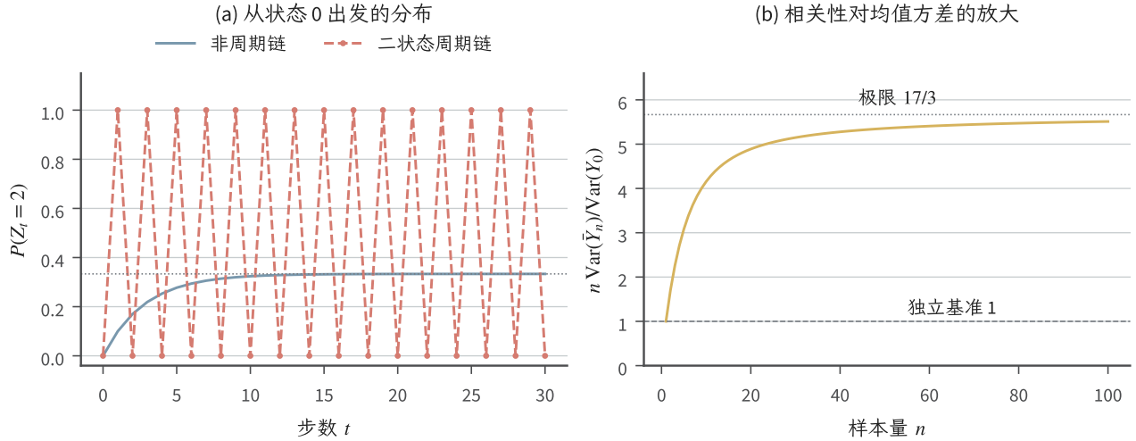
图 10.7 两状态链的解析式教学图。左图蓝线使用例 10.81 的转移矩阵，从 Z_0 = 0 出发绘制 \mathbb{P}(Z_t = 2) = (1 - 0.7^t)/3 ；红线使用确定交替的转移矩阵。右图使用平稳初态和 \rho_k = 0.7^k ，绘制 1 + 2 \sum_{k=1}^{n-1} (1 - k/n) \rho_k ，其极限为 17/3 ，独立观测基准为 1。
