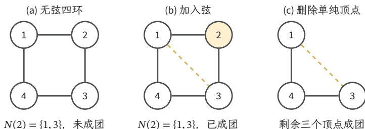
图 9.7 四环补入弦 1-3 后, 顶点 2 的两个邻居已经相邻。删除 2 不需填充, 余图 \{1, 3, 4\} 是团, 因此 (2, 1, 3, 4) 是补弦图的完美消元序。补边改变了原图的路径与分离关系, 不能把右图当作左图所有查询的等价表示。
