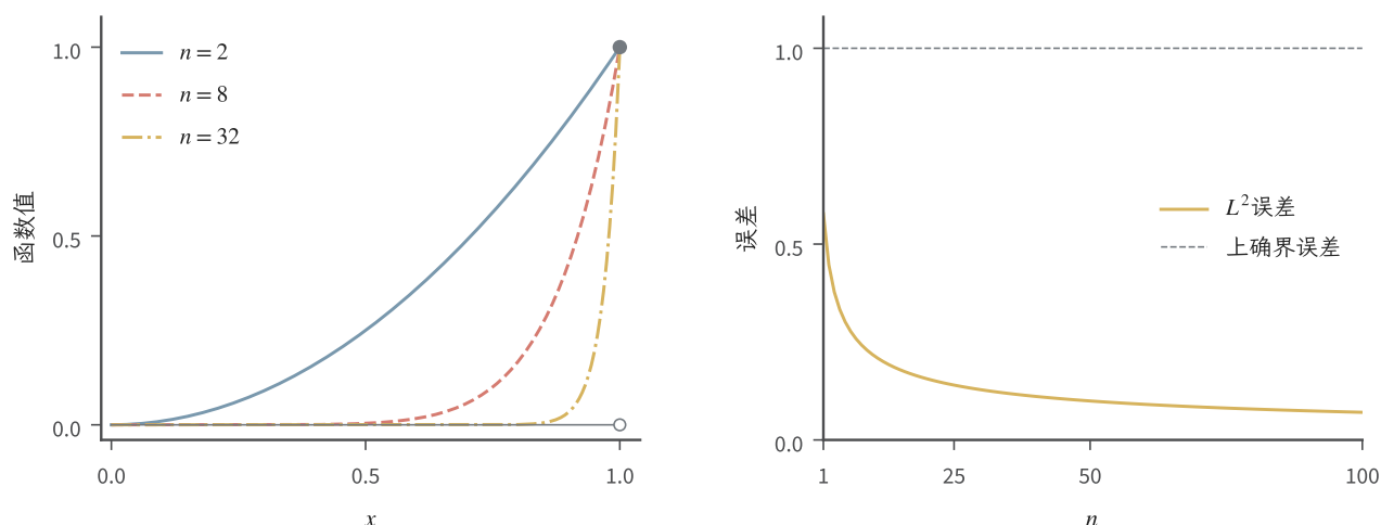
图 3.7 x^n 在 [0, 1] 上的两种整体尺度。左图蓝、红、黄线分别取 n = 2, 8, 32 ；灰线与端点标记表示逐点极限，它在 x < 1 处为零、在 x = 1 处为 1。右图黄色曲线为精确的 L^2 误差 (2n+1)^{-1/2} ，灰虚线为始终等于 1 的普通上确界误差；单点 x = 1 的修改不影响积分。图解析教学示例。
