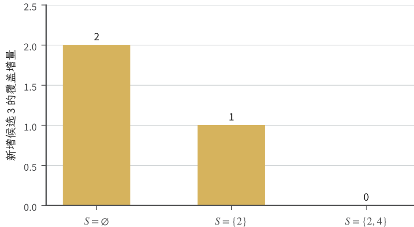
图 2.10 覆盖函数的有限教学构造。使用式 (2.19) 中的 Q_2, Q_3, Q_4 ，向 \emptyset \subset \{2\} \subset \{2, 4\} 分别加入候选 3，覆盖增量为 2, 1, 0。柱高从零基线起画；图中只展示一个具体递减链，完整次模性仍由集合差证明。
