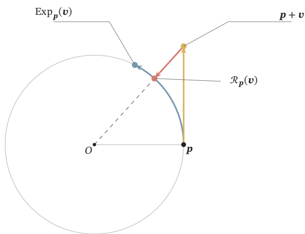
图 7.6 单位圆截面中的切向步、指数映射与归一化回缩。取 \mathbf{p} = (1, 0)^\top 、 \mathbf{v} = (0, 1.1)^\top 。黄色箭头为切向步，终点 \mathbf{p} + \mathbf{v} 位于圆外；红色径向箭头将该点归一化为 \mathcal{R}_p(\mathbf{v}) 。从起点方向计，蓝色指数更新转过 1.1 弧度，归一化回缩转过 \arctan(1.1) \approx 0.833 弧度。两种更新关于步长的曲线在零步长处有相同初速度，但有限步位置不同。图为解析教学示例。
