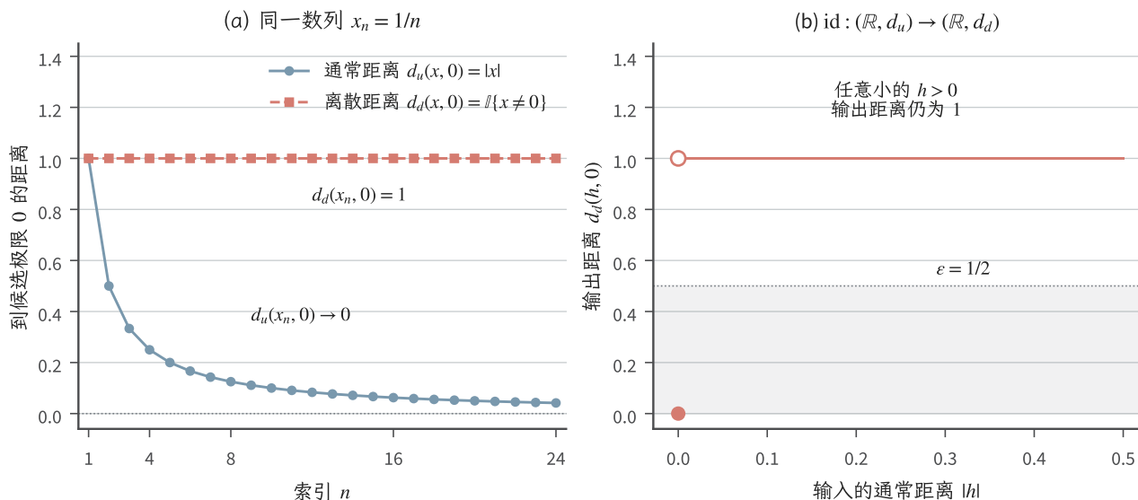
图 3.2 数值相同，距离不同。图中 d_u, d_d 分别对应正文的通常距离 d_1 与离散距离 d_2 。(a) 数列 x_n = 1/n 到 0 的通常距离趋于零，离散距离却恒为 1，所以收敛要连同度量说明。(b) 恒等映射从通常度量空间映入离散度量空间时，任意非零且很小的输入位移仍对应输出距离 1，不能进入 \varepsilon = 1/2 的输出邻域，故它在 0 处不连续。图为解析教学示例。
