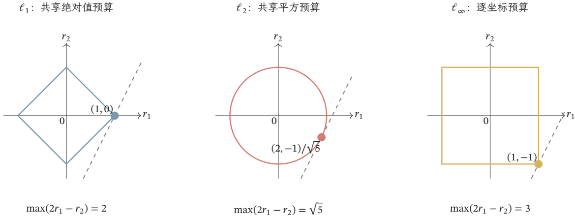
图 6.1 同一线性读取 2r_1 - r_2 在 \ell_1 、 \ell_2 、 \ell_\infty 单位球上的最大值依次为 2、 \sqrt{5} 、3。虚线为最后接触可行集的支撑直线，点为最大化方向。三图坐标尺度相同，均为解析教学例；改变允许误差的形状会改变误差常数。
