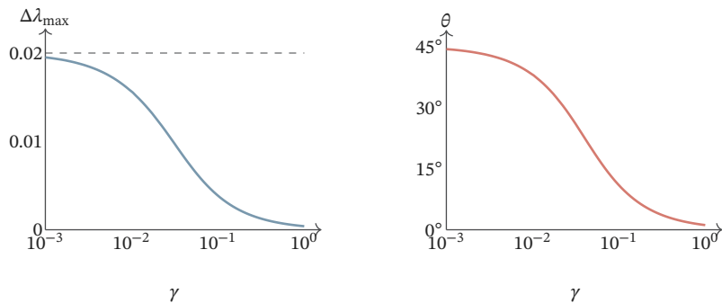
图 6.9 同一对称扰动下，谱值稳定不等于方向稳定，固定 \epsilon = 0.02 。左图为最大特征值增量 \Delta\lambda_{\max} = \sqrt{(\gamma/2)^2 + 0.02^2} - \gamma/2 ，灰虚线为扰动范数 0.02；右图为最大特征方向转角 \theta = \frac{1}{2} \arctan(0.04/\gamma) ，角度用度表示。两图横轴均为原始谱隙 \gamma ，采用相同的对数刻度。所有数值均来自二阶特征方程的解析解。
