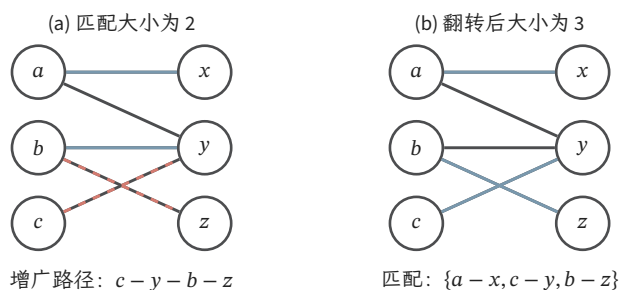
图 9.9 沿交替路径重新安排匹配。两组顶点为 U = \{a, b, c\} 、 W = \{x, y, z\} 。蓝实线是已选边，左图红虚线是增广路径的未选边，灰线是其余候选边。翻转 c-y-b-z 后保留 a-x ，得到三条互不共享端点的边。线条表达候选配对，不表达因果方向。
