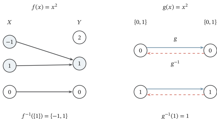
图 1.1 原像与逆映射回答不同问题。左侧 f : \{-1, 0, 1\} \rightarrow \{0, 1, 2\} 按平方取值，标出的 1 有两个原输入，2 没有原输入；原像 f^{-1}(\{1\}) = \{-1, 1\} 仍有定义。右侧将定义域与陪域都限制为 \{0, 1\} 得到双射 g ，实线表示正向求值，虚线表示逆映射，因而 g^{-1}(1) = 1 是一个元素。两侧均为精确的有限映射。
