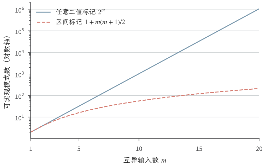
图 2.3 有限输入上的二值模式数（精确计数教学图）。蓝实线为不受限制的 2^m ，红虚线为实数轴区间分类器的 1 + m(m+1)/2 。纵轴使用对数刻度，红线是该具体类的精确计数；它也恰等于至多两个正类点的集合族计数，但两类实现的模式可以不同。
