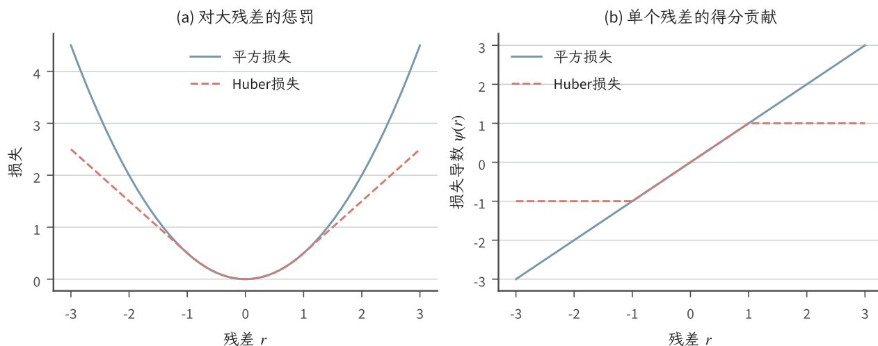
图 10.10 平方损失与阈值 c = 1 的 Huber 损失 (解析式教学图)。左图比较惩罚值, 右图比较对残差的导数; Huber 得分在 [-1, 1] 内截断。横轴是构造残差, 不代表实测异常值分布。
