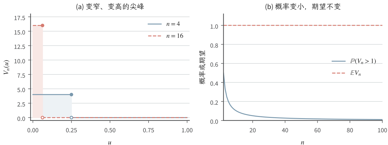
图 10.5 小概率尖峰与期望质量 (解析式教学图)。左图为 V_n(u) = n\mathbb{I}\{u \leq 1/n\} 在 n = 4, 16 时的取值, 均以面积 1 贡献期望; 右图对 n \geq 2 显示 \mathbb{P}(V_n > 1) = 1/n 趋于零, 而 \mathbb{E}V_n = 1 不变。基础变量为 U \sim \text{Unif}(0, 1) 。
