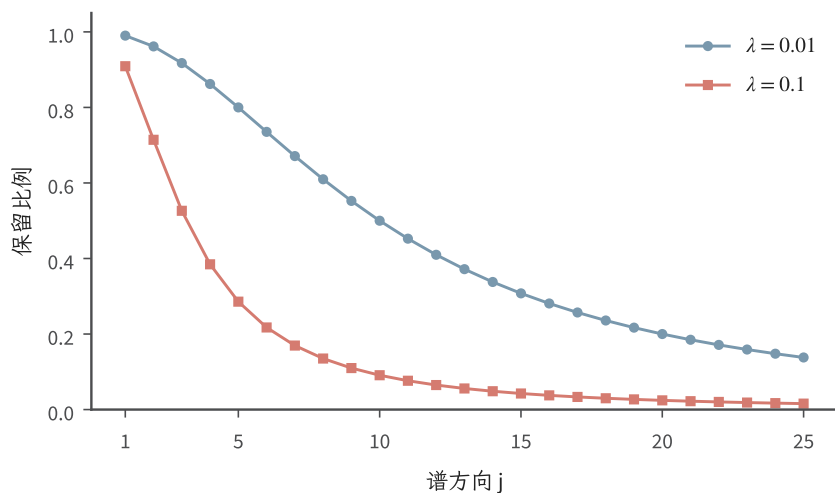
图 5.8 教学谱 \mu_j = j^{-2} 上的收缩比例 \mu_j / (\mu_j + \lambda) 。蓝、红线使用 \lambda = 0.01 和 0.1 ，点标出前 25 个方向；增大正则化后更多方向被抑制。有效维度的定义仍对全部谱方向求和。
