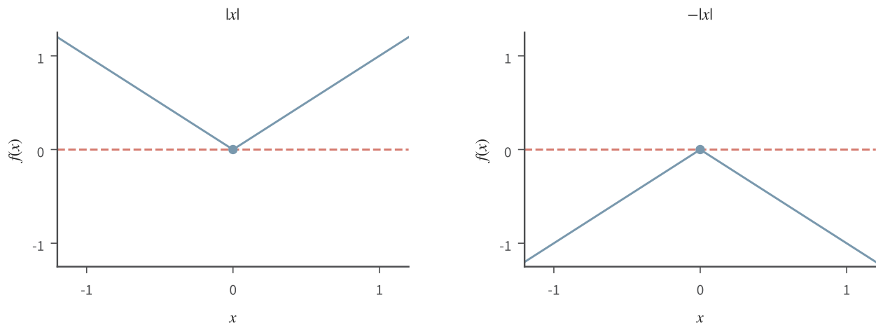
图 3.5 同一广义驻点条件的不同含义。蓝线分别为 |x| 与 -|x| ，红虚线为原点处候选斜率 g = 0 对应的直线。两图在原点的 Clarke 广义梯度均为 [-1, 1] ，却分别形成局部最小点与局部最大点；只有左图红线是全局仿射下界。两图共用坐标尺度，由解析式生成。
