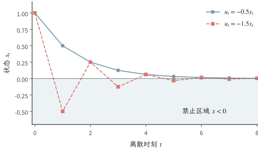
图 14.3 教学系统 x_{t+1} = x_t + u_t 从 x_0 = 1 出发。蓝色圆点采用 u_t = -0.5x_t , 保持 x_t \geq 0 ; 红色方点采用 u_t = -1.5x_t , 第一步进入禁止的负半轴后交替衰减。两者都渐近稳定, 只有前者保持安全集合。灰色区域表示禁止状态。
