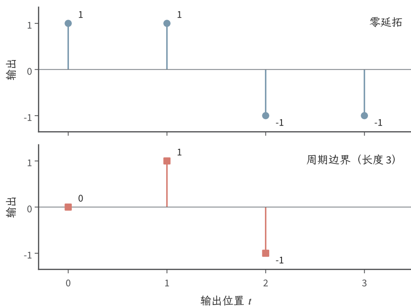
图 8.4 输入 (1, 2, 1) 与核 (1, -1) 的边界比较。蓝色圆点采用零延拓，给出四项线性卷积；红色方点采用长度 3 的循环边界，末项 -1 回到首项并与 1 抵消。连线只指示离散数值的顺序，不定义整数之间的信号值。
