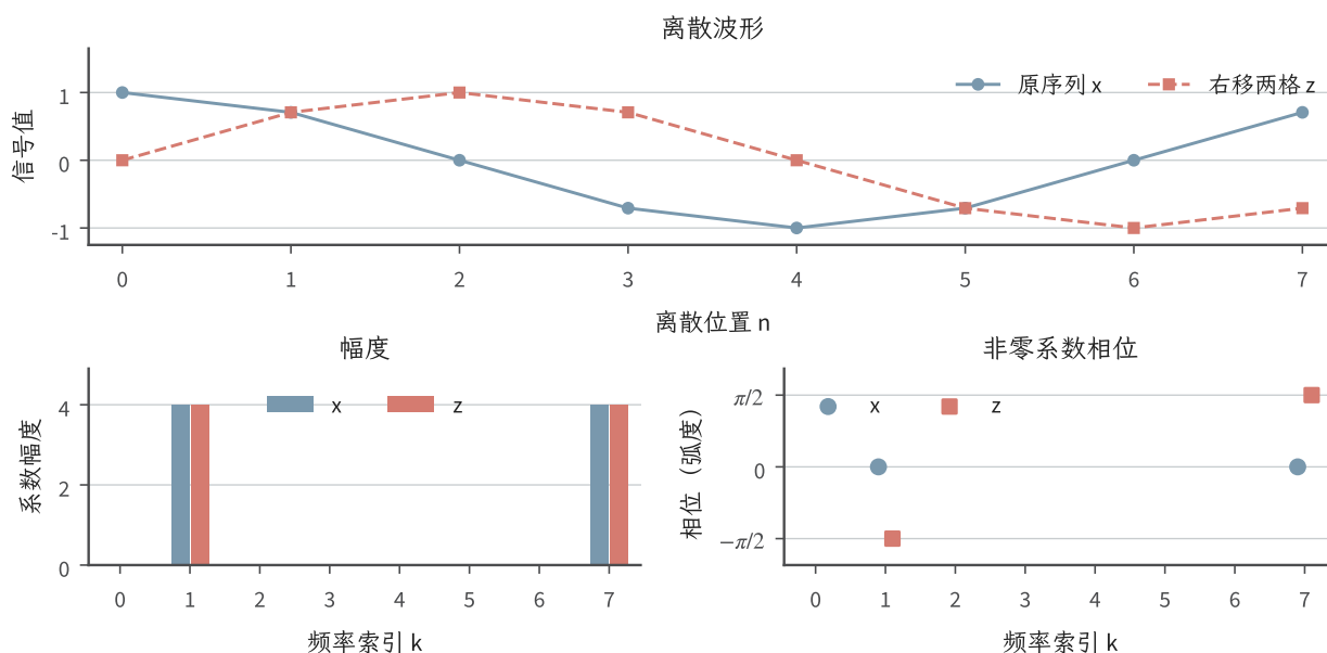
图 8.1 长度 8 的教学信号 x[n] = \cos(2\pi n/8) 及其循环延迟两格的结果。上方波形的峰值位置不同，下方在 k=1,7 的幅度均为 4，相位却改变。相位图只画非零系数；波形连线只帮助观察顺序，不表示已选择连续时间插值。
