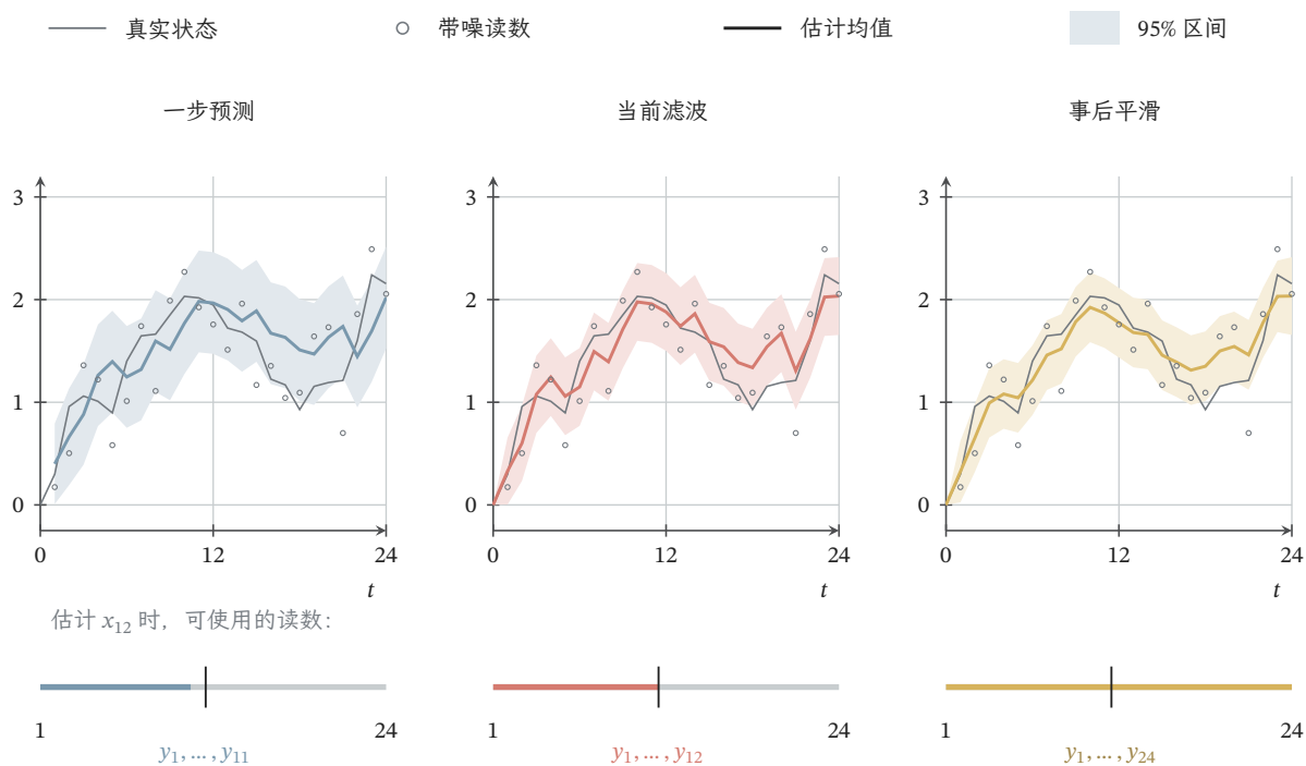
图 13.8 与图 13.4 完全相同的温度轨迹及读数。三栏分别画一步预测、滤波与固定终点 T = 24 的平滑均值和逐时刻 95% 高斯区间，灰线为实际状态，圆点为读数；区间不是整条路径同时覆盖的置信带。下方以 t = 12 为例标出可用观测范围。已知 x_0 = 0 ，给定 u_t = 0.4 ，过程、观测方差仍为 0.04, 0.09。平滑的信息优势不是额外的在线能力。
