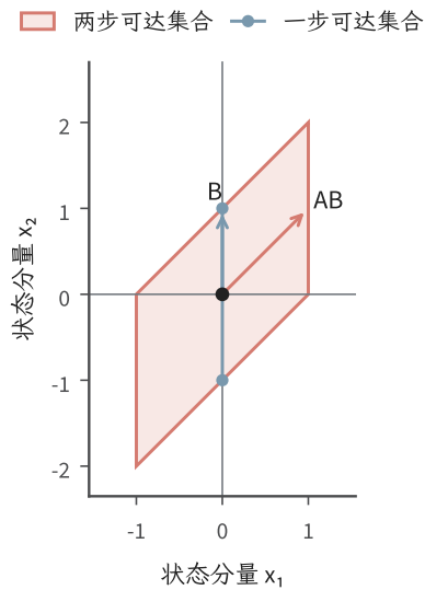
图 14.1 教学系统 \mathbf{A} = \begin{bmatrix} 1 & 1 \\ 0 & 1 \end{bmatrix} 、 \mathbf{B} = (0, 1)^\top 从零出发。蓝色线段为 |u_0| \leq 1 的一步可达集合，红色区域为 |u_0|, |u_1| \leq 1 的两步可达集合；箭头为 \mathbf{B} 与 \mathbf{AB} 。幅值限制用于显示可达区域，不属于无约束可控性秩判据的假设。
