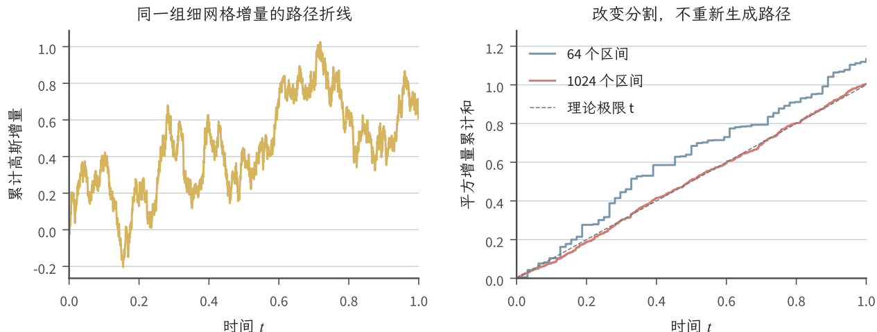
图 10.9 以固定随机种子构造的高斯增量教学例。左图由 4096 个独立增量 \Delta W_i \sim \mathcal{N}(0, 1/4096) 累计成路径折线；右图将同一组增量分别合并为 64 和 1024 个时间区间，再累计各区间增量的平方。蓝、红阶梯线使用不同分割，灰色参考线为理论二次变差 t 。这里只绘制有限网格，不把某一条折线作为连续布朗路径或收敛证明。
