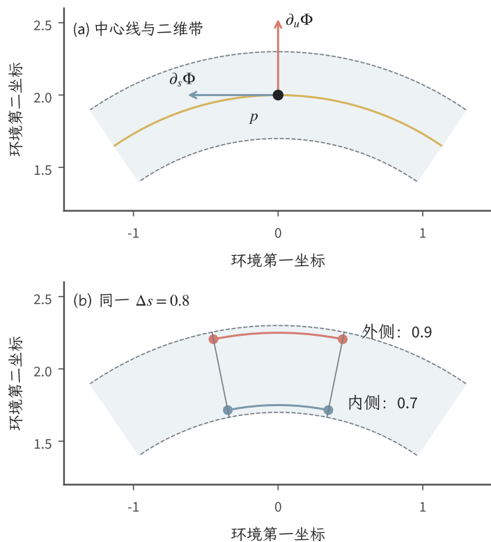
图 7.3 开带与中心线的局部方向不同。取 R = 2 、 w = 0.3 。上图的两个参数方向属于二维开带，仅以中心线为对象时，径向方向不属于其切空间；箭头平移到 \mathbf{p} 只是画法。下图取 u = -0.25, 0.25 ，同一 \Delta s = 0.8 对应圆弧长度 0.7, 0.9。灰虚线为不纳入开带的边界，两图等比例绘制，均为解析教学示例。
