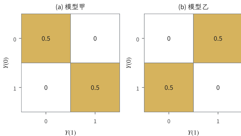
图 12.1 相同干预边缘的两种跨世界配对。行对应 Y(0) ，列对应 Y(1) ，格内数字为联合概率；每张表的行和、列和均为 1/2。甲的个体效应恒为零，乙的个体效应等概率取 1, -1，两者 ATE 均为零。这是相容机制的教学构造，不是随机试验直接观察到的潜在结果联合表。
