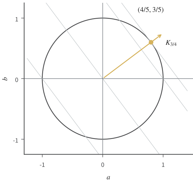
图 5.7 仿射 RKHS 中读取 f(3/4) = a + 3b/4 。灰圆表示 a^2 + b^2 \leq 1 ，黄箭头是核截面 K_{3/4} 对应的系数 (1, 3/4) ；灰平行线为相同点值。黄圆点 (4/5, 3/5) 达到单位范数球上的最大点值 5/4 。这里坐标是函数系数，不是输入位置。图为解析教学示例。
