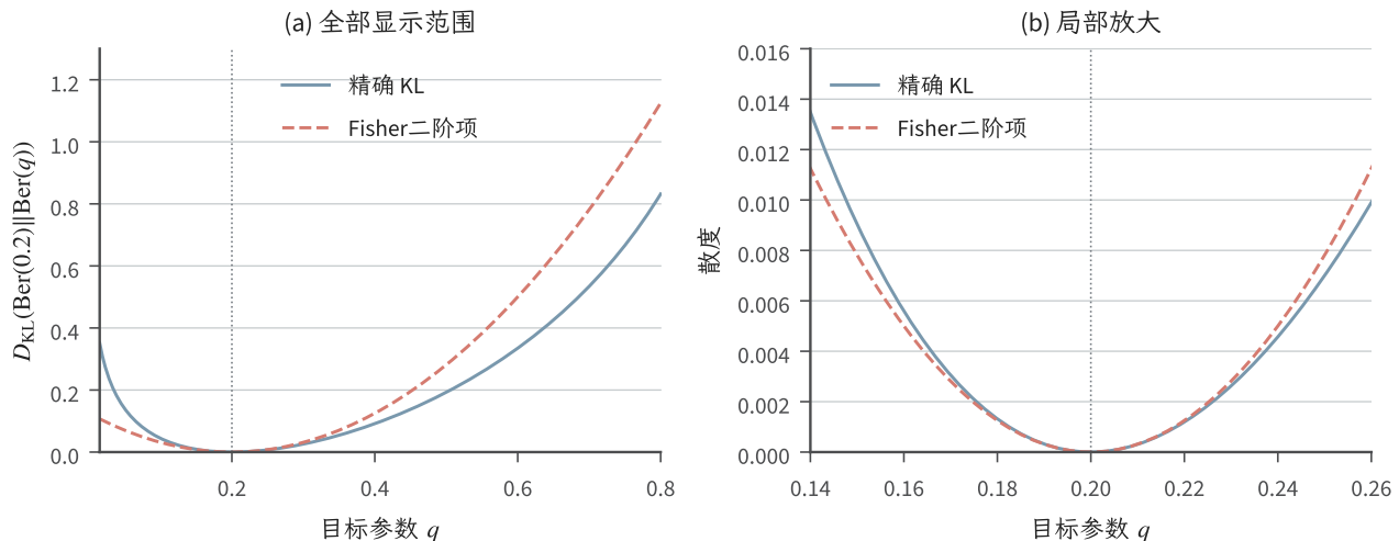
图 11.6 Bernoulli 族在 p = 0.2 处的 Fisher 局部近似（解析式教学图）。蓝实线为 D_{\text{KL}}(P_{0.2} \parallel P_q) ，红虚线为 (q - 0.2)^2 / [2(0.2)(0.8)] ；右图放大邻域。图中 0 < q < 1 ，二阶式只描述足够小的参数扰动。
