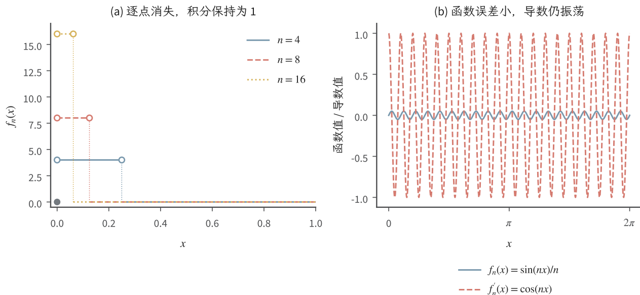
图 3.8 两种交换运算的障碍。左图的尖峰支撑不断收缩，但高度同步增长，每条曲线的积分仍为 1；开圆点标出不取的上端点，竖虚线仅提示跳跃。右图取 n = 20 ， \sin(nx)/n 的函数幅度很小，导数 \cos(nx) 仍有单位幅度。两图均为按给定函数公式构造的教学示例。
