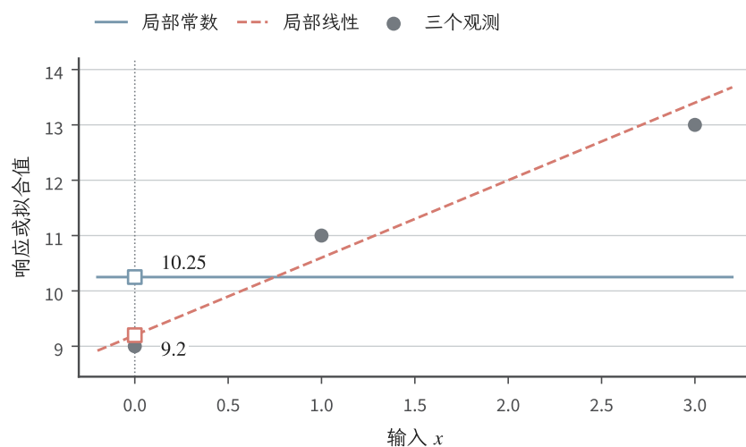
图 10.11 边界处的局部常数与局部线性拟合（教学数据图）。观测为 (0, 9), (1, 11), (3, 13) ，权重为 1, 0.75, 0.25 。蓝实线为加权常数 10.25，红虚线为 9.2 + 1.4x ，边界 x_0 = 0 处分别预测 10.25 和 9.2。
