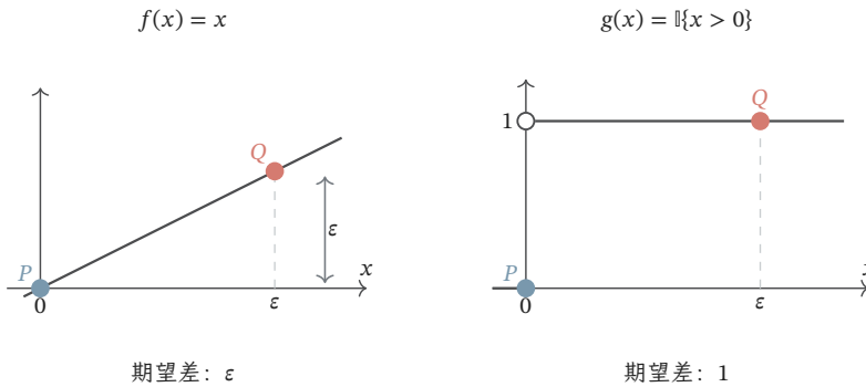
图 11.4 同一小位移对两种固定评价的影响。取 P = \delta_0 、 Q = \delta_\varepsilon 、 \varepsilon > 0 ，底层距离为绝对值。左图的 1-Lipschitz 函数 f(x) = x 变化 \varepsilon ；右图的事件函数 \mathbb{I}\{x > 0\} 变化 1。横向位置仅作示意，结论对任意正的 \varepsilon 成立。
