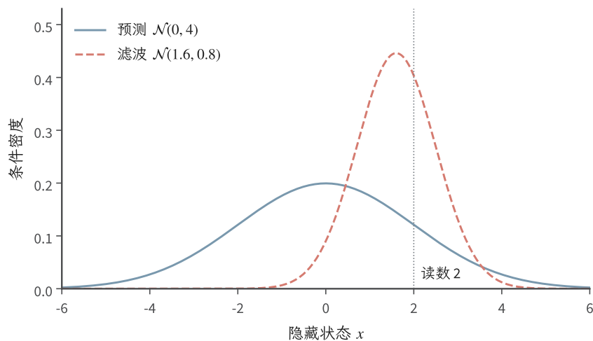
图 13.7 独立标量教学例的预测 \mathcal{N}(0, 4) 与后验 \mathcal{N}(1.6, 0.8) , 实际读数 y = 2 、观测噪声方差 1。第二个高斯参数是方差; 本图不是贯穿温度模型的参数设定。
