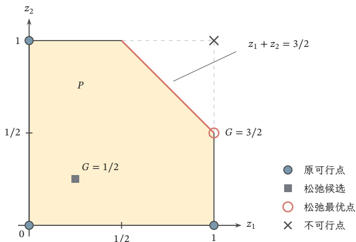
图 2.11 式 (2.27) 的精确可行域。浅黄多边形为松弛范围 P ，蓝色实心圆点为原零一可行点，灰色方点的目标值仅为 1/2 ，红色空心圆点达到松弛最优值 3/2 ；右上角叉号为取整后不可行的 (1, 1) 。红色线段满足 z_1 + z_2 = 3/2 ，整个 P 都在该线的低值一侧。
