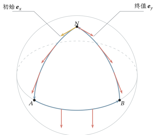
图 7.5 单位球面上沿 N \rightarrow A \rightarrow B \rightarrow N 的平行移动。蓝色为给定的三条大圆弧，红箭头为例 7.24 中逐段计算的切向量。沿路协变导数为零，返回 N 后的方向却由黄色初始箭头 e_x 变为红色终值箭头 e_y 。箭头在三维中等长，投影到纸面后的长度可以不同。图解析教学示例。
