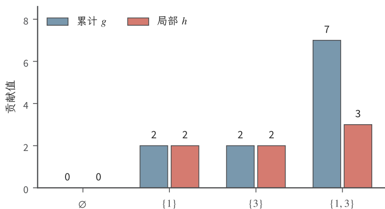
图 2.1 同一四元素教学构造在 \{1, 3\} 的子集上的累计值与局部贡献。蓝柱为 g , 红柱为 h ; 单项贡献各为 2, 二元累计值 7 包含额外交互 3。图中四个子集的数据由正文解析式精确计算, 没有省略影响这个二元交互的子集。
