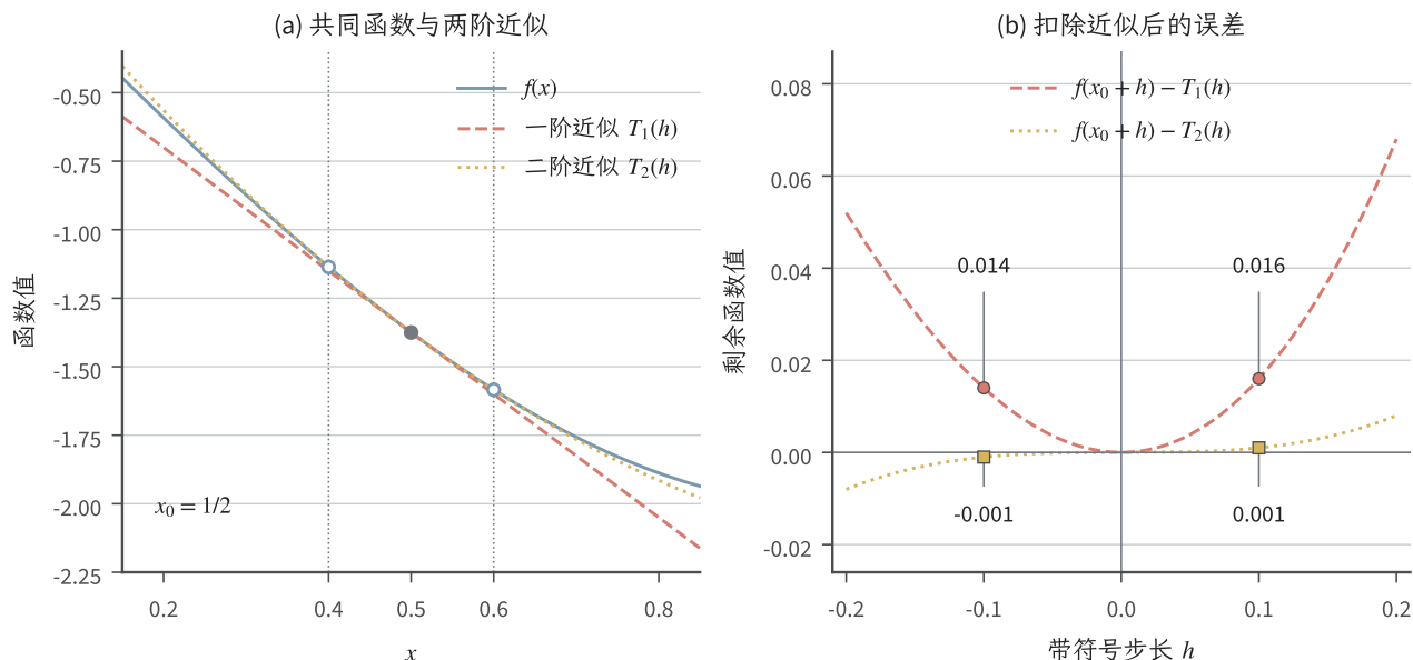
图 3.4 统一函数 f(x) = x^3 - 3x 在 x_0 = 1/2 处的两阶近似, 记 h = x - x_0 。(a) 蓝线为真函数, 红虚线为切线近似 T_1 = f(x_0) + f'(x_0)h , 黄点线加入二次项 f''(x_0)h^2/2 , 得到 T_2 。(b) 扣除各近似后的带符号余项分别为 3h^2/2 + h^3 与 h^3 , 标出 h = \pm 0.1 的精确结果。一阶导数确定切线, 二阶导数补充局部曲率; 余项的正负表示真值位于近似值的哪一侧。图为解析教学示例。
