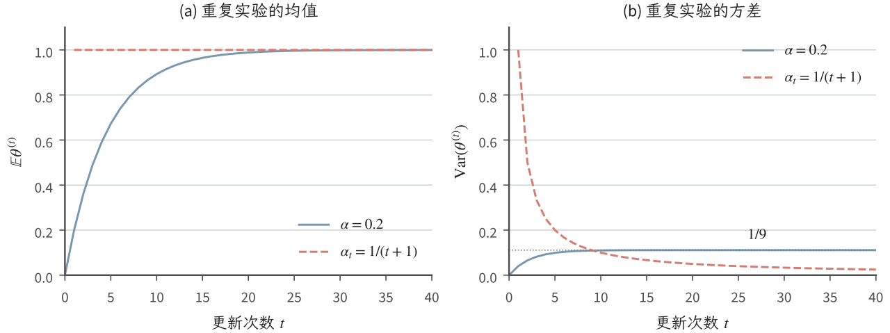
图 13.5 同一均值问题的重复实验均值与方差。取 \theta^{(0)} = 0, \mu = 1, \sigma^2 = 1 , 观测独立同分布; 蓝实线为固定 \alpha = 0.2 , 红虚线为 \alpha_t = 1/(t+1) 。固定步长方差趋于 1/9 , 样本平均方差为 1/t 。曲线由解析式得到, 不是一条样本轨迹。
