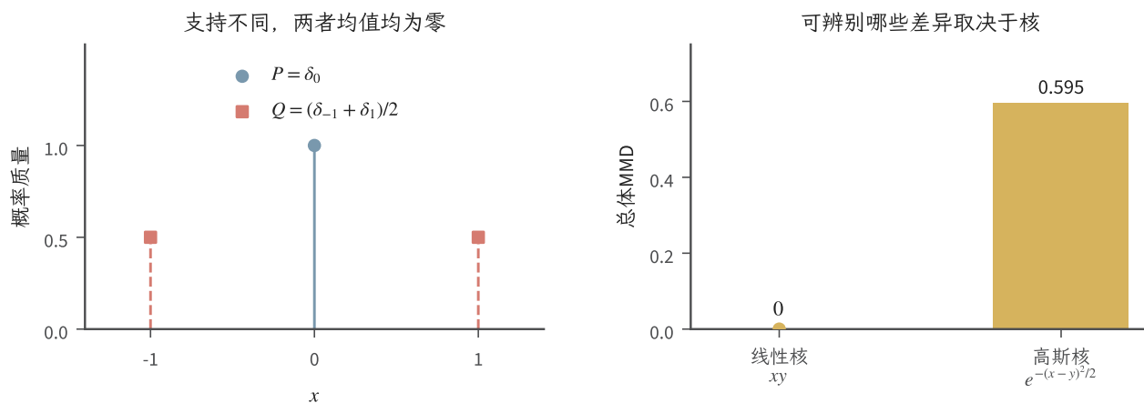
图 11.2 同均值分布在不同核下的 MMD (解析式教学图)。左图为 P = \delta_0 与 Q = (\delta_{-1} + \delta_1)/2 , 右图按精确总体期望计算: 线性核给出零, 高斯核给出约 0.595。没有使用有限样本估计; 差别来自测试函数类。
