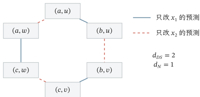
图 2.7 六模式族 \mathcal{V} 的逐坐标邻接。每个顶点是一种两输入预测; 蓝实线只改变第一坐标, 红虚线只改变第二坐标。每个顶点在两个方向上都有邻居, 所以它构成二维伪立方体; 图中没有固定两标签对形成的四角矩形, 故其 DS 维为 2 而 Natarajan 维为 1。
