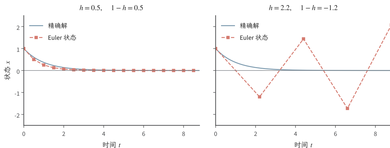
图 13.1 教学方程 \dot{x} = -x 、 x(0) = 1 的精确解与 Euler 近似。蓝色实线为精确解, 红色方点为数值状态; 左图 h = 0.5 衰减, 右图 h = 2.2 交替增长。两图采用相同坐标范围, 连线只连接相邻数值状态。右图的发散来自步长, 并非原连续系统不稳定。
