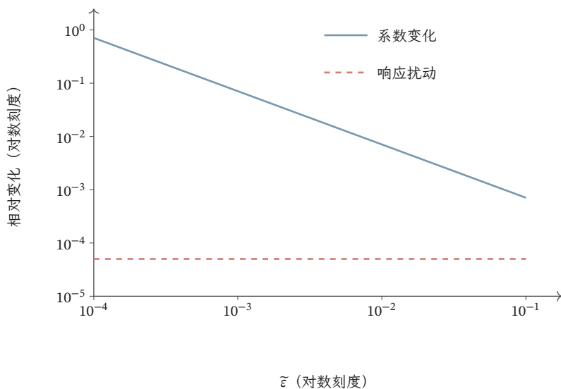
图 6.8 近共线矩阵的精确敏感性。固定 \mathbf{y}_0 = (2, 0)^\top , 扰动为 (0, 10^{-4})^\top ; 红线是响应相对扰动 5 \times 10^{-5} , 蓝线是系数相对变化 10^{-4}/(\sqrt{2}\epsilon) 。双对数坐标显示列越接近, 反求系数越敏感; 图中没有数值求解误差。
