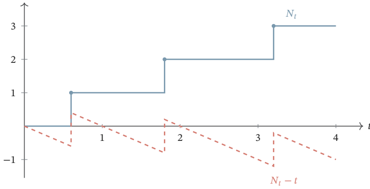
跳跃量同为 1；补偿只加入斜率 -1 的连续漂移
