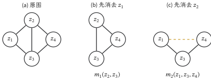
图 9.6 两个初步消元产生不同接口。删去 z_1 后，新表索引 (z_2, z_3) ；删去 z_2 后，通常须索引 (z_1, z_3, z_4) ，黄虚线为填充边 1-4 。二值稠密接口表分别有 4 和 8 项，虽然两张余图都只剩三个顶点。特殊函数可能还能分解；图给出的是通用作用域范围。
