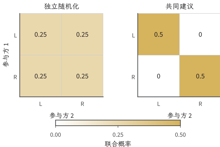
图 16.2 二行动协调博弈的两个教学联合分布，共用 0 至 0.5 的概率色阶。行为参与者 1 的行动，列为参与者 2 的行动。左图为独立均匀策略，四格质量均为 0.25；右图只推荐 (L, L) 与 (R, R) ，各占 0.5。两者边缘概率均为 (0.5, 0.5) ，但每人期望收益分别为 1 和 2；相关分布并非边缘分布的乘积。
