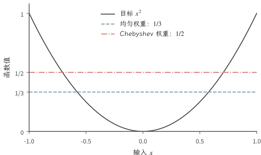
图 5.3 对 x^2 使用同一候选空间 \text{span}\{1, x\} ，均匀权重的最佳常数为 1/3 ，Chebyshev 权重的最佳常数为 1/2 。目标、区间和候选空间保持相同，只改变误差积分的权重。曲线由解析式生成。
