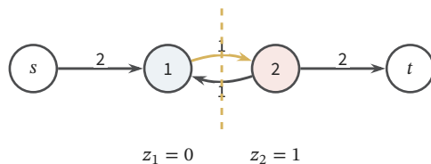
图 9.10 两变量能量的割表示, 零容量弧省略。割把 s, 1 与 2, t 分开, 因而标签为 z_1 = 0, z_2 = 1 。两个容量为 1 的反向弧中, 仅源侧到汇侧的黄弧 1 \rightarrow 2 计费, 成本不是 2。终端弧 s \rightarrow 1 的容量 2 = D_1(1) 只在顶点 1 进入汇侧时支付。
