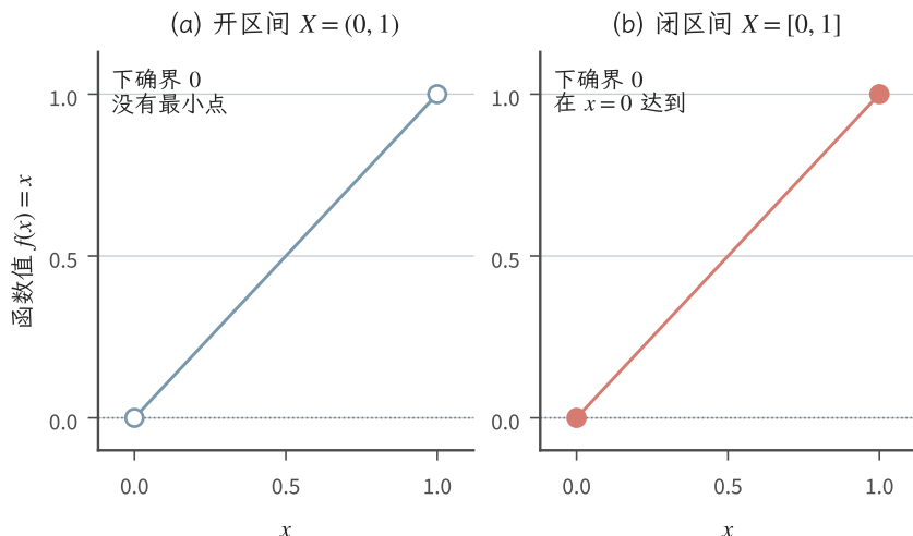
图 1.2 同一函数 f(x) = x 的边界对照。左图定义域为 (0, 1) ，空心端点不属于图像，函数值可任意接近 0，却不能取到；右图定义域为 [0, 1] ，实心端点 (0, 0) 达到下确界。两图的下确界相同，最小点是否存在取决于可行端点是否保留。图为解决教学示例。
