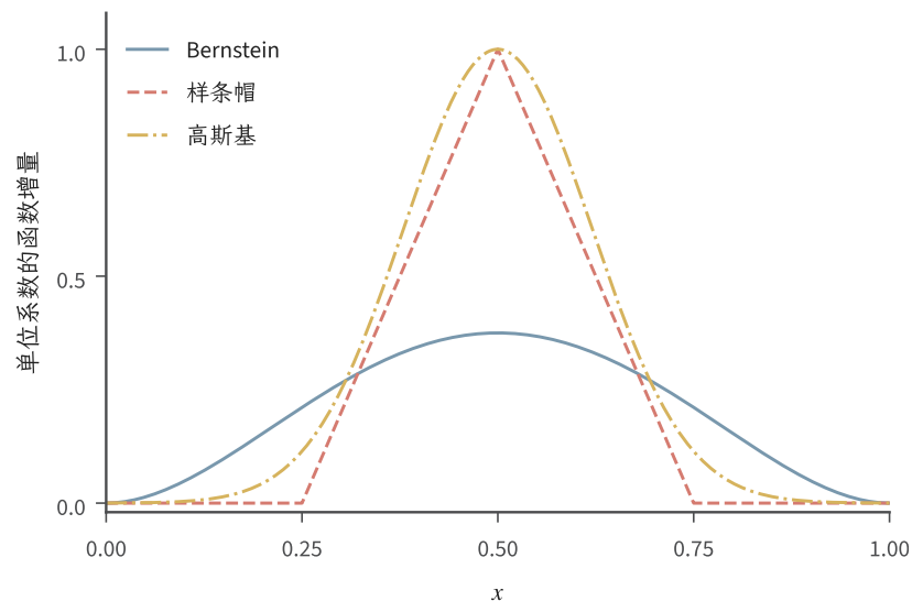
图 5.4 单个系数改变对函数的影响。蓝线为 6x^2(1-x)^2 ，即四阶 Bernstein 多项式的中心基；红线为中心 1/2 、相邻结点 1/4, 3/4 的线性样条帽；黄线为中心 1/2 、宽度 0.12 的高斯基。系数增量均为 1 ，不另行缩放峰高；图比较作用范围，未比较三种方法的最优逼近误差。
