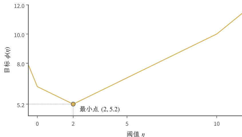
图 15.1 教学分布 P(L=0)=0.6 、 P(L=2)=0.3 、 P(L=10)=0.1 在 \alpha=0.75 下的阈值目标 \phi(\eta) = \eta + 4\mathbb{E}[(L-\eta)_+] 。暖黄色折线的最小点为 (2, 5.2); 阈值 2 与尾部平均 5.2 不能混用。
