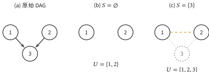
图 9.4 祖先道德图随查询条件改变。端点固定为 1, 2；空条件集时，查询图只有两个孤立顶点。给定 3 时，先扩大的祖先集合使道德化加入黄虚线 1-2，随后删除灰色条件点及灰点线，却不删除这条新增边。不能先道德化整图再取查询顶点。
