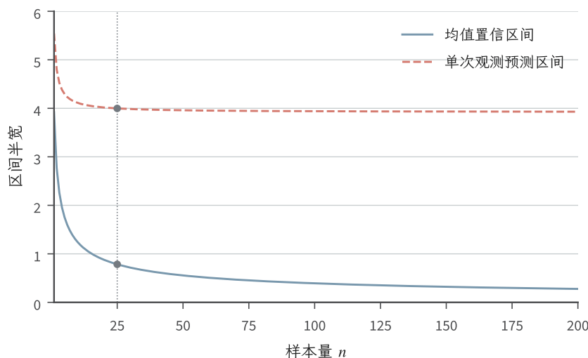
图 10.12 已知 \sigma = 2 的独立高斯位置模型中, 两类区间半宽随样本量变化 (解析式教学图)。使用四舍五入分位数 1.96, 蓝实线为 1.96\sigma/\sqrt{n} , 红虚线为 1.96\sigma\sqrt{1 + 1/n} 。灰竖线标出例 10.96 的 n = 25 , 没有对任何实测数据重复抽样。
