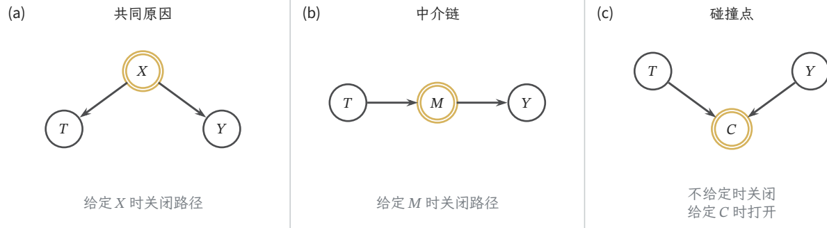
图 12.3 共同原因、中介与碰撞点的局部路径。双边框表示节点已加入条件集。共同原因和中介是非碰撞点，给定后关闭这条路径；给定碰撞点则打开原本关闭的路径。路径打开表示图不再保证相应独立性，并不指定相关的大小或正负。
