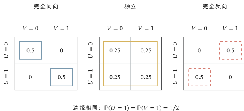
图 10.3 边缘质量相同的三个联合分布。格内数字是联合概率，各行各列的和始终为 1/2 ；质量的位置改变协方差及和的分布。
