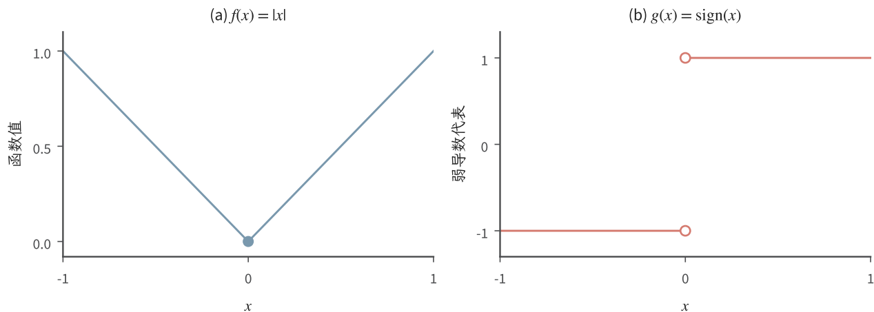
图 5.2 f(x) = |x| 与其一阶弱导数 g(x) = \text{sign}(x) 。左图原点为连续尖点；右图两段分别为 -1 与 1 ，空心端点表示经典导数在原点未定义。
