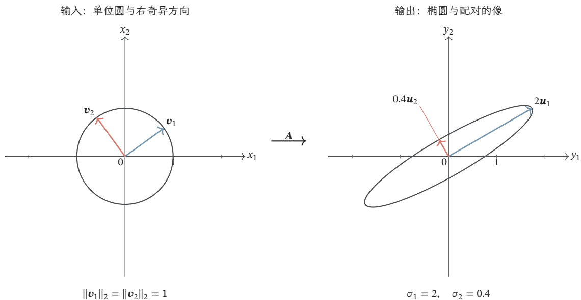
图 6.6 矩阵 \mathbf{A} = \mathbf{R}(\pi/6) \text{diag}(2, 0.4) \mathbf{R}(\pi/5)^T 将单位圆变为椭圆。蓝、红箭头分别标出右奇异方向 \mathbf{v}_i 及其像 \sigma_i \mathbf{u}_i ；两侧坐标比例相同。奇异值决定长度变化，左右方向可以不同，因而这不是沿特征方向的同空间缩放。图为教学构造。
