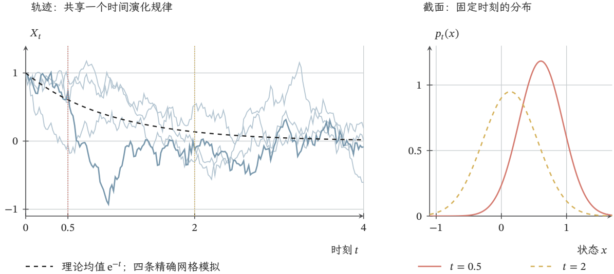
图 13.6 OU 模型的路径与截面。取 \lambda = 1, \sigma = 0.6, X_0 = 1 ，左侧为按精确高斯转移生成的四条网格轨迹与理论均值，右侧为 t = 0.5, 2 的解析边缘密度。折线只连接模拟网格点，不是可微的连续样本路径。截面给出单时刻概率，时间间的相关性还由共同噪声与转移决定。
