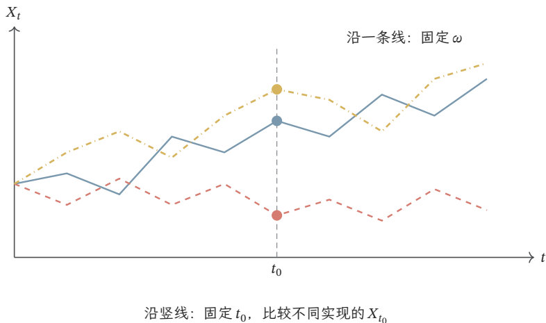
图 10.6 同一过程的路径与时刻截面是不同对象。图为人为给定的三条示意路径，竖虚线固定时刻 t_0 ；交点展示该时刻可能出现的不同值，并非用三条路径估计出的概率密度。
