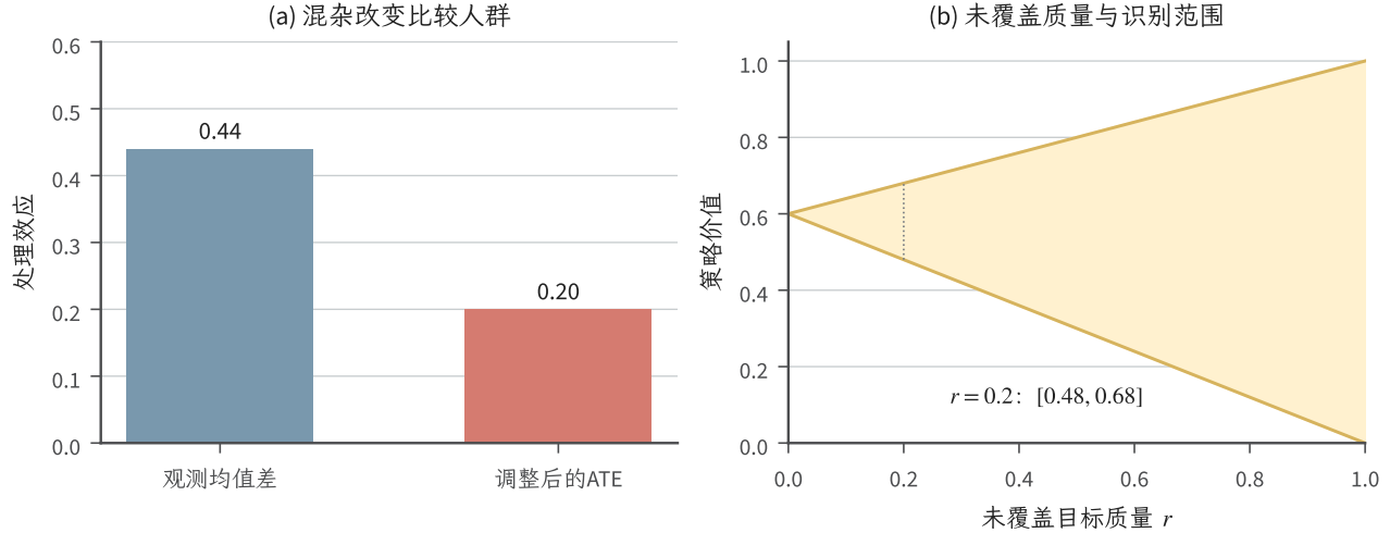
图 12.2 两个独立的教学构造。左图比较风险分层例子的观测均值差 0.44 与调整效应 0.20。右图按式 (12.31) 绘制 [0.6(1 - r), 0.6(1 - r) + r] 。阴影为总体识别范围，不是抽样置信带；两个面板不表示同一数据集。
