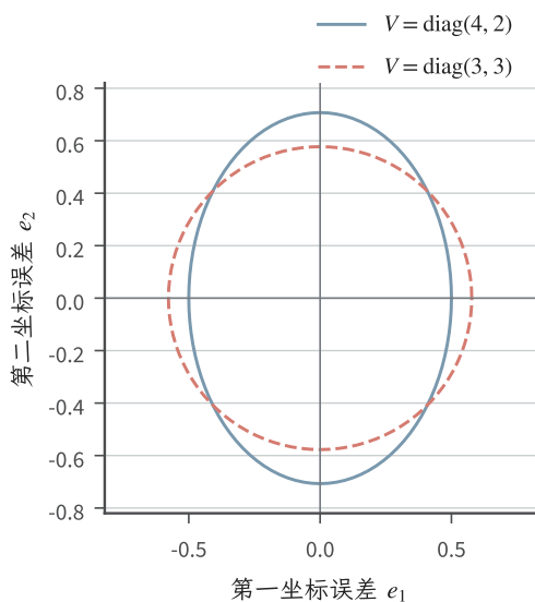
图 10.13 二维设计的归一化误差几何(解析式教学图)。蓝实线为 \mathbf{e}^\top \text{diag}(4, 2)\mathbf{e} = 1 ，红虚线为 \mathbf{e}^\top \text{diag}(3, 3)\mathbf{e} = 1 。它们不是已经具有相同覆盖概率的数值置信区间；真实置信半径由式 (10.62) 另行确定。
