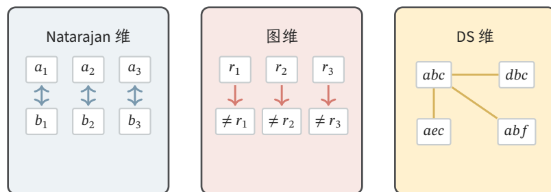
图 2.8 多分类维度关注的三种结构。Natarajan 维固定每个输入处的两个标签，图维固定一个基准标签并区分匹配与不匹配，DS 维考察预测向量之间只改变一个坐标的邻接。右栏只展示局部邻接方式；完整伪立方体还要求每个模式在每个坐标上都有邻居。
