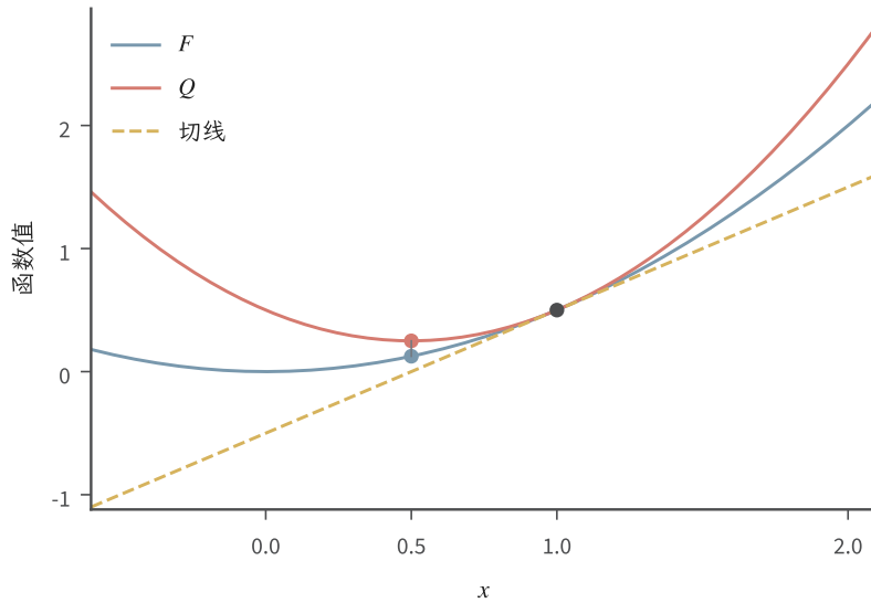
图 4.7 代理上界与切线的区别。蓝线为 F(x) = x^2/2 ，红线为当前点 1 处的主化代理 Q ，黄虚线为同点切线 x - 1/2 。三者在当前点同值同斜率，但切线位于目标下方，最小化它不能使用 MM 的上界链；红点标出代理最小点对应的值。图为解析教学示例。
