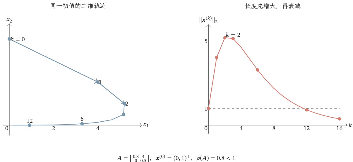
图 6.5 固定二维矩阵的反复作用。初值为 (0, 1)^T , 前两步的长度增加, 此后回到原点; 右图将长度与初始长度 1 比较。特征值 0.8 和 0.5 决定长期衰减, 非正交特征方向间的相消则决定早期放大。两图使用同一个矩阵和同一组迭代点。
