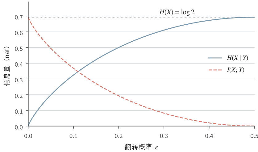
图 11.1 公平二元输入通过独立翻转通道后的信息分配（解析式教学图）。蓝实线为剩余条件熵 H_b(\epsilon) ，红虚线为互信息 \log 2 - H_b(\epsilon) ，均以 nat 计。输入熵保持不变，零噪声与公平翻转分别对应完整信息与零信息。
