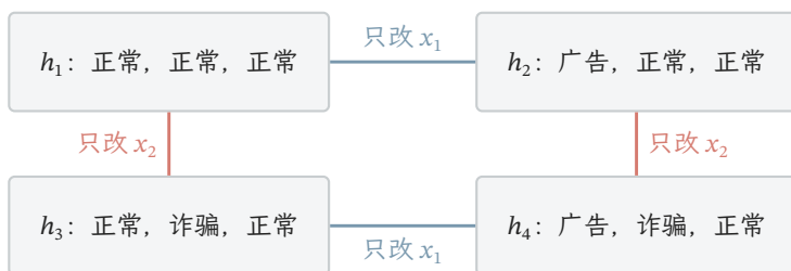
图 2.6 Natarajan 打散的四函数。每个框中的三项依次对应 x_1, x_2, x_3 ; 横向只改变 x_1 , 纵向只改变 x_2 , 而 x_3 始终预测为正常。每个输入处的两个标签预先固定, 四个函数实现全部二选一组合。
