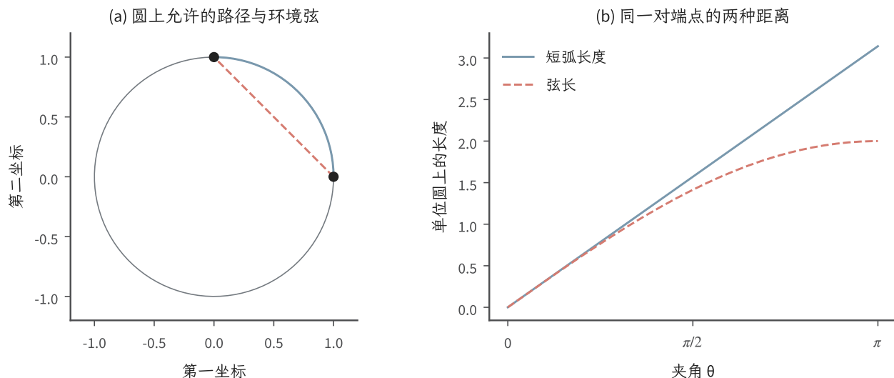
图 7.4 完整单位圆的测地距离与环境弦长。左图夹角为 \pi/2 ，蓝线为圆上的允许短弧，红虚线为穿过圆内的环境线段；右图比较 \theta \in [0, \pi] 时的两种长度。完整圆允许选择两段弧中的较短者，不能与开中心线或二维开带的允许路径混用。图为解决教学示例。
