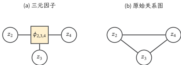
图 9.2 三元因子与原始关系图。左侧方框是同一个依赖 z_2, z_3, z_4 的函数，连线表示作用域归属；右侧只保留变量共同出现的两两关系。右侧三条边不是把三元函数分解成三个二元函数的等价变换，也不能恢复原函数的数值。
