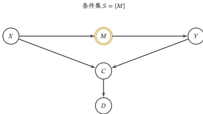
图 12.4 多条路径下的 d-分离。双边框节点 M 属于条件集，上方链式路径关闭；碰撞点 C 及其后代 D 都未给定，下方路径也关闭。若再把 C 或 D 加入条件集，下方路径就会打开，说明增加条件可能破坏原有的分离。
