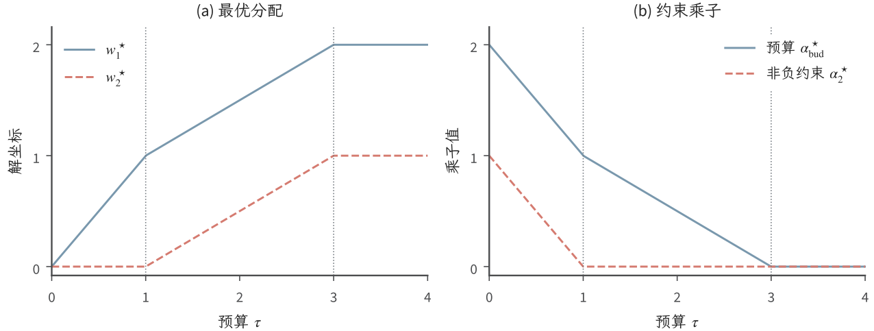
图 4.5 例 4.19 的解析解。左图为两个最优分配坐标，右图为预算乘子与第二个非负约束的乘子。竖参考线标出 \tau = 1, 3 ；在切换点约束可以取等号而乘子为零，说明活跃性与正价格并不等价。
