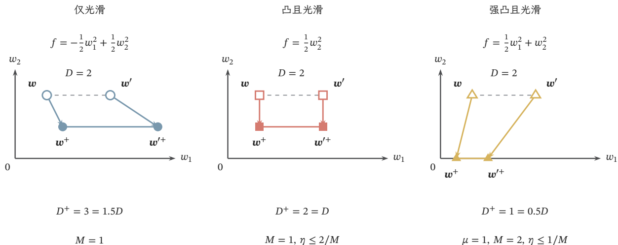
图 7.4 同一梯度更新如何影响参数距离。三个参数平面使用相同尺度，初值均为 w = (1, 2)^T 、 w' = (3, 2)^T ，步长均为 \eta = 1/2 。空心标记表示初值，实心标记表示 w^+ = w - \eta \nabla f(w) 及 w'^+ ；箭头表示各自的梯度步，虚线和实线连接更新前后的两点。图中二次函数的梯度步给出精确距离 D^+ = 3, 2, 1 ，并非一般情形的距离等式。凸且 M -光滑时， \eta \leq 2/M 保证不扩张；满足本章强凸光滑条件时， \eta \leq 1/M 保证至多以 1 - \mu\eta 收缩。仅有光滑性不能排除扩张。
