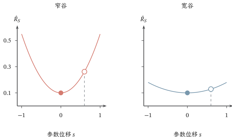
图 8.7 同尺度的窄谷与宽谷损失截面。横轴为同一单位方向上的参数位移 s ，即 \theta = \hat{\theta} + s\mathbf{u} 、 \|\mathbf{u}\|_2 = 1 。构造的窄谷与宽谷分别为 0.1 + 0.45s^2 、 0.1 + 0.08s^2 ；实心点为谷底，空心点对应相同位移 s = 0.6 ，经验风险分别增加 0.162 和 0.0288。两面板共用相同横纵尺度。这是扰动代价的教学示意，不表示宽谷必然具有较小的期望风险。
