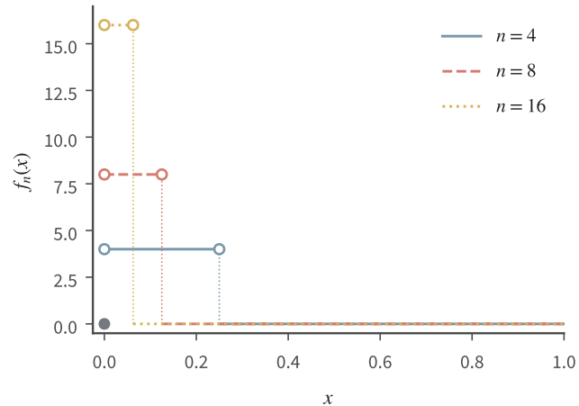
(a) 逐点消失，积分保持为 1
