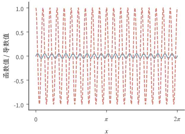
(b) 函数误差小，导数仍振荡
