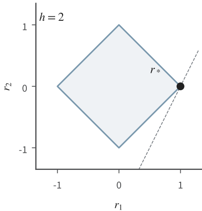
(a) \|r\|_1 \leq 1
