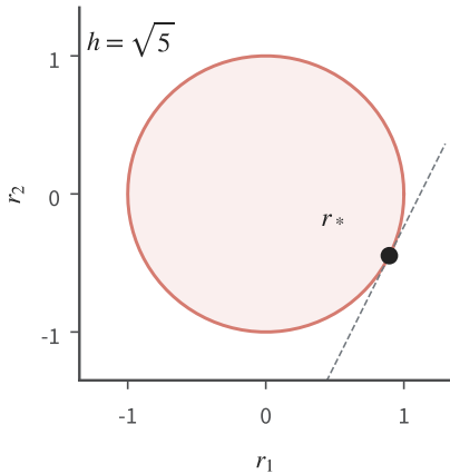
(b) \|r\|_2 \leq 1
