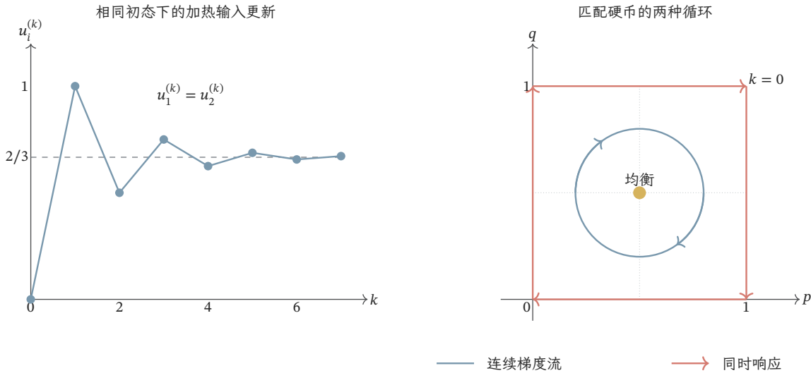
图 16.4 两个已明确更新规则的教学轨迹。左图为相同初态下双加热器的同时最佳响应，从 u_1^{(0)} = u_2^{(0)} = 0 开始，两条输入曲线重合，误差交替减半并趋向 2/3 。右图红色方形箭头是匹配硬币的离散四周期，蓝色圆是内部连续梯度流从 (p, q) = (0.8, 0.5) 出发的闭轨道，中心黄点是 Nash 均衡。圆与方形对应不同更新，均不是最佳响应对应图中的静态集合。
