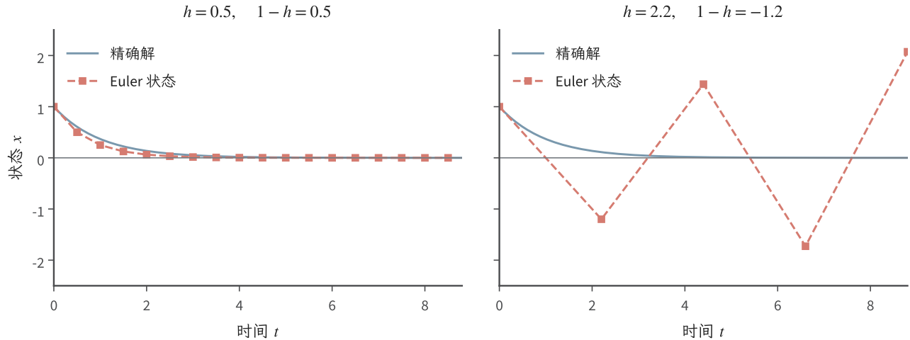
图 13.1 教学方程 \dot{x} = -x 、 x(0) = 1 的精确解与 Euler 近似。蓝色实线为精确解，红色方点为数值状态；左图 h = 0.5 衰减，右图 h = 2.2 交替增长。两图采用相同坐标范围，连线只连接相邻数值状态。右图的发散来自步长，并非原连续系统不稳定。
