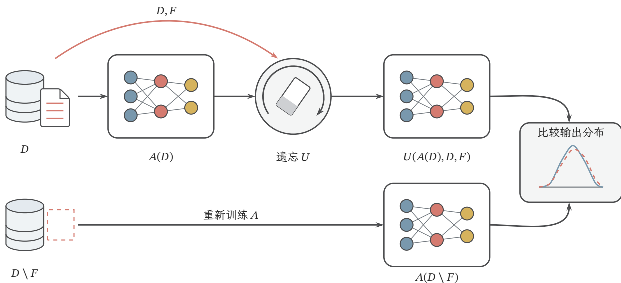
图 16.3 撤回记录与消除训练影响的两条路径。下方从 D 中移除 F ，得到保留数据 D \setminus F ，上方旧模型 A(D) 不会因此自动改变；更新程序 U 另行读取旧模型、原数据和撤回集合。更新结果与从未使用 F 的重训练参照比较所发布模型的分布；精确遗忘要求同分布，近似遗忘须声明距离或可区分性标准。
