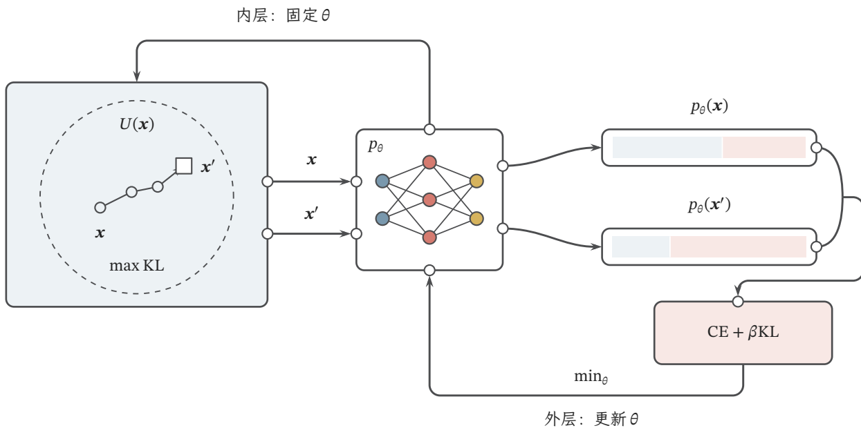
图 12.3 TRADES 中的内层搜索与外层更新。内层在 U(x) 中近似增大原输入与扰动输入预测分布的 KL 散度，外层最小化原输入分类损失与加权 KL 项，再用更新后的参数重新搜索。箭头示意搜索轨迹，概率条只示意分布发生偏离，不来自实验。该训练流程不提供全邻域的形式证书。
