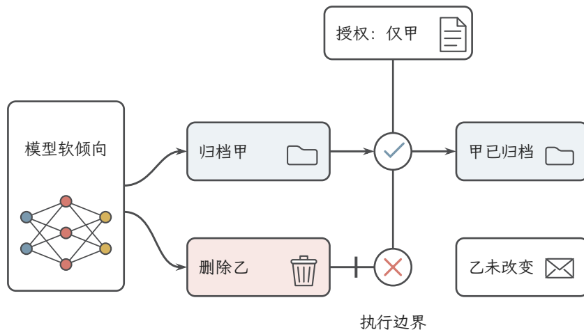
图 14.3 模型内的行为倾向与执行外的权限边界。训练可以改变模型提出何种动作的倾向，却不能作为硬权限的保证。甲、乙表示两封邮件，独立可信记录只允许处理甲；归档甲的提案获准执行，删除乙的提案被拒，乙的状态不变。执行端另行核对授权与当前状态，提案不能扩大许可集合。安全状态的保持仍依赖正文中的转移覆盖与安全动作存在等条件。
