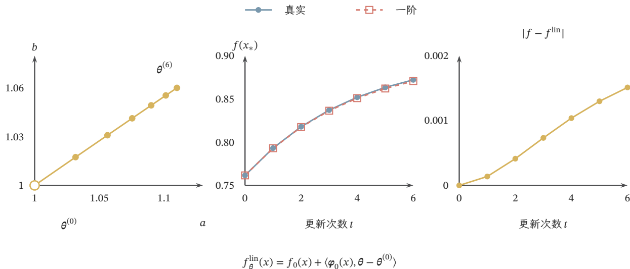
图 8.4 初始化附近的参数轨迹与输出线性化。教学网络为 f_{(a,b)}(x) = a \tanh(bx) , 初值为 (1, 1)^\top ; 用单个样本 (x, y) = (1, 0.9) 的半平方损失、步长 0.3 执行六次梯度下降, 连同初值共七个检查点。中间的真实输出和一阶输出均在左侧同一参数轨迹上计算; 三面板绘图区大小相同, 参数、输出和绝对余项各用所标坐标范围, 不能按纸面高度直接比较数值。右侧余项末次约为 0.00152。近初始化时二者接近, 但余项并非零。参数增量经初始雅可比映射到输出/函数空间的切空间; NTK 是初始梯度在不同输入上的内积。此有限网络示例展示近似对象, 不证明训练中核恒定或新输入上的误差受控。
