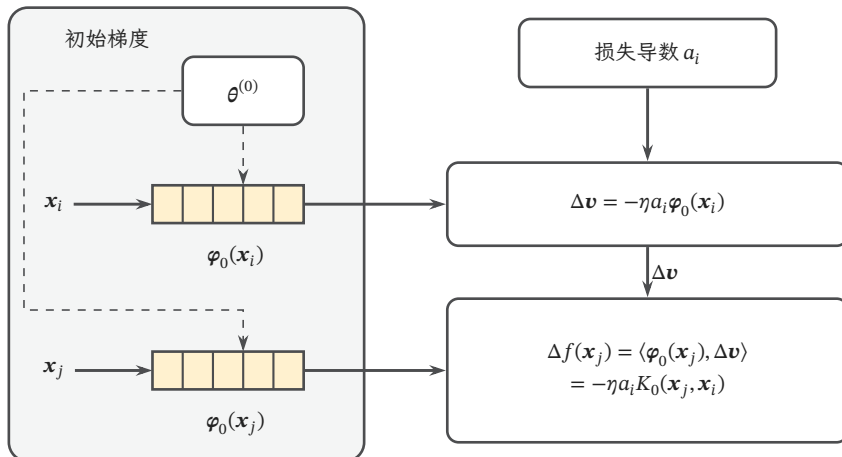
图 8.5 初始梯度特征如何传递一次训练更新。在线性化模型中，样本 i 的梯度特征与损失对预测的导数 a_i 共同确定参数增量 \Delta \mathbf{v} ；将同一增量与样本 j 的梯度特征作内积，得到 \Delta f(\mathbf{x}_j) 。核值 K_0 正是两个初始梯度特征的内积。虚线把两份梯度关联到同一初始化，特征条仅示意梯度坐标，不限定参数维数。对真实有限宽网络使用固定特征，还需控制核变化与线性化误差。
