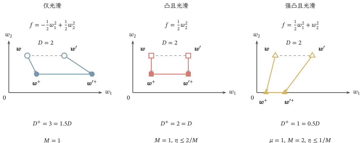
图 7.4 同一梯度更新如何影响参数距离。三个参数平面使用相同尺度，初值均为 w = (1, 2)^\top 、 w' = (3, 2)^\top ，步长均为 \eta = 1/2 。空心标记表示初值，实心标记表示 w^+ = w - \eta \nabla f(w) 及 w'^+ ；箭头表示各自的梯度步，虚线和实线连接更新前后的两点。图中二次函数的梯度步给出精确距离 D^+ = 3, 2, 1 ，并非一般情形的距离等式。凸且 M -光滑时， \eta \leq 2/M 保证不扩张；满足本章强凸光滑条件时， \eta \leq 1/M 保证至多以 1 - \mu\eta 收缩。仅有光滑性不能排除扩张。
