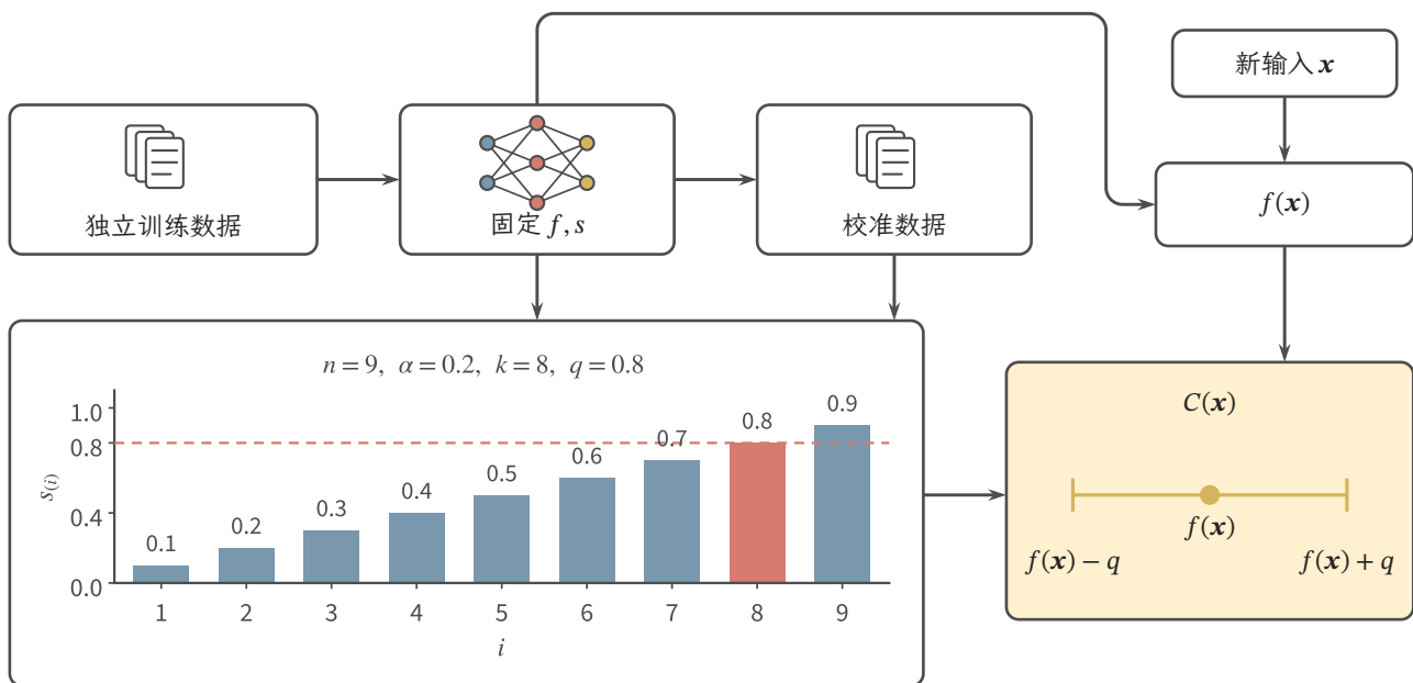
图 11.6 拆分共形预测的构造。评分函数先由独立训练数据确定, 再用校准分数选择阈值。图中采用教学残差 0.1, 0.2, ..., 0.9, 取 n = 9, \alpha = 0.2 , 故 k = 8, q = 0.8 ; 绝对残差评分产生右侧回归区间。数值说明排序与集合构造, 不是覆盖率的实验测量。
