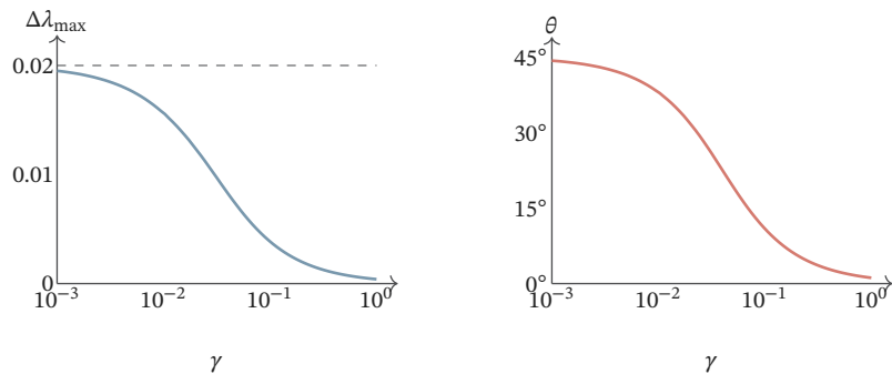
图 6.9 同一对称扰动下, 谱值稳定不等于方向稳定, 固定 \epsilon = 0.02 。左图为最大特征值增量 \Delta\lambda_{\max} = \sqrt{(\gamma/2)^2 + 0.02^2} - \gamma/2 , 灰虚线为扰动范数 0.02; 右图为最大特征方向转角 \theta = \frac{1}{2} \arctan(0.04/\gamma) , 角度用度表示。两图横轴均为原始谱隙 \gamma , 采用相同的对数刻度。所有数值均来自二阶特征方程的解析解。
