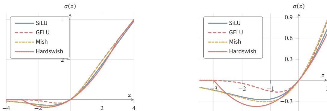
图 8.7 SiLU、GELU、Mish 与 Hardswish。左图展示整体响应，右图放大原点附近的负值和过渡区域；GELU 按标准正态累积分布函数采样。它们在正端接近线性，但负区间的形状和拐点不同。SiLU、GELU 与 Mish 平滑，Hardswish 含有分段边界；两图使用不同坐标范围以显示细节。
