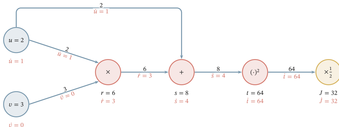
图 8.11 具体算子图上的前向模式。圆形节点表示乘法、加法、平方和缩放; 实线上方的黑色数字是传入算子的值, 下方红色数字是同一路径上的方向导数。每个算子下方再用两行列出其输出值和输出方向导数。输入方向 (1, 0) 给出 \partial J / \partial u = 32 ; 加法处的 \dot{s} = 3 + 1 包含了 u 的两条路径。
