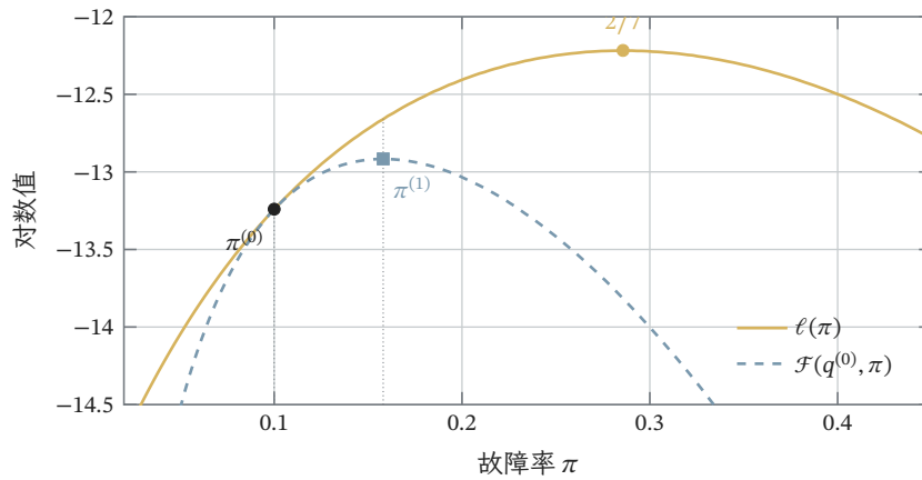
图 24.1 故障率例子的第一轮 EM。实线是观测对数似然，虚线是固定 \pi^{(0)} = 0.1 后验所得的下界。两者在旧参数处相等；下界在 \pi^{(1)} \approx 0.158044 处最大，而观测对数似然在 2/7 处最大。图中纵轴为自然对数，曲线可由正文公式直接复算。
