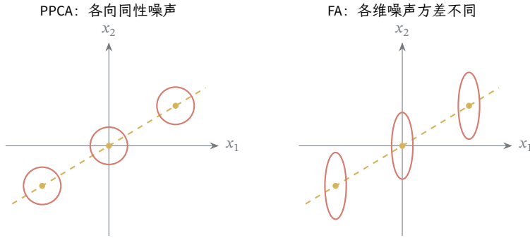
图 5.11 PPCA 与 FA 的条件噪声示意。设 d = 2 、 k = 1 、 \mu = \mathbf{0} 、 \mathbf{W} = (1, 0.6)^\top ，三个实心点对应 z = -1, 0, 1 的条件均值。左图取 \sigma = 0.28 ，右图取 \Psi = \text{diag}(0.16^2, 0.50^2) ；每条轮廓到其中心的平方 Mahalanobis 距离均为 1。坐标为无量纲构造值，轮廓是条件等密度线，不是总体数据云或置信区域。
