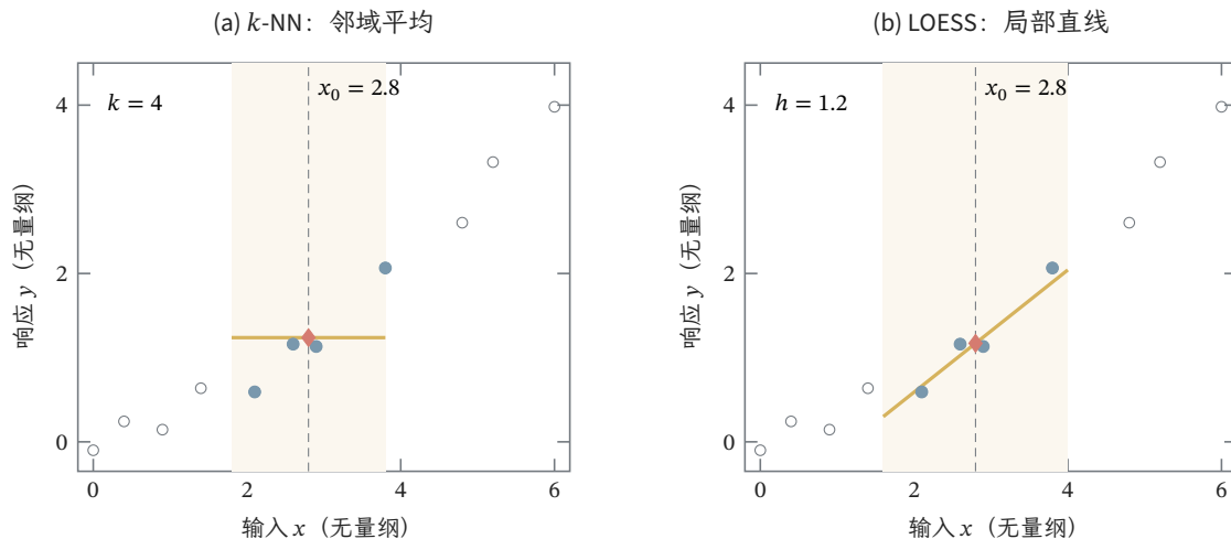
图 2.4 同一查询点上的邻域平均与局部线性拟合。横、纵轴均无量纲，所有点均为构造样本；空心点为未使用样本，蓝色实心点为本次使用的四个样本，菱形为 x_0 = 2.8 处的预测。左图取 k = 4 、等权平均，预测约为 1.238；右图取 h = 1.2 与三立方距离权重，不做残差重加权，局部线性预测约为 1.171。浅色带标出各自的邻域，两图同时改变了局部函数形式和权重，不据此断言某种方法总是更准。
