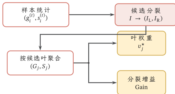
(b) XGBoost：二阶统计进入树评分
