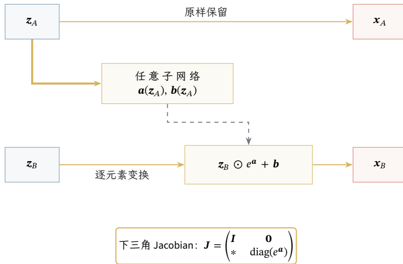
图 29.2 仿射耦合层的计算依赖。粗线把 \mathbf{z}_A 送入任意子网络, 该子网络只产生缩放和平移参数; 下方逐元素仿射变换才真正改变 \mathbf{z}_B 。Jacobian 为下三角结构, 因此子网络不必可逆, 整层的对数行列式只需对缩放对数求和。逆向计算先恢复原样保留的 \mathbf{z}_A , 再撤销缩放和平移。
