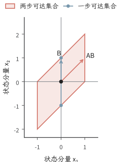
图 14.1 教学系统 \mathbf{A} = \begin{bmatrix} 1 & 1 \\ 0 & 1 \end{bmatrix} 、 \mathbf{B} = (0, 1)^\top 从零出发。蓝色线段为 |u_0| \leq 1 的一步可达集合，红色区域为 |u_0|, |u_1| \leq 1 的两步可达集合；箭头为 \mathbf{B} 与 \mathbf{A}\mathbf{B} 。幅值限制用于显示可达区域，不属于无约束可控性秩判据的假设。
