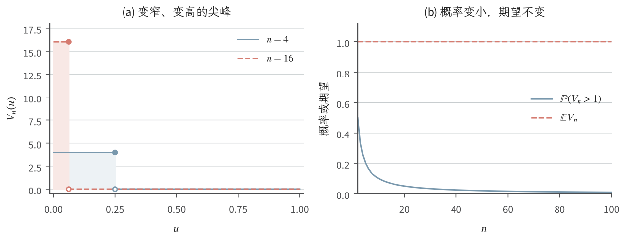
图 8.5 小概率尖峰与期望质量 (解析式教学图)。左图为 V_n(u) = n\mathbb{I}\{u \leq 1/n\} 在 n=4, 16 时的取值, 均以面积 1 贡献期望; 右图对 n \geq 2 显示 P(V_n > 1) = 1/n 趋于零, 而 EV_n = 1 不变。基础变量为 U \sim \text{Unif}(0, 1) 。
