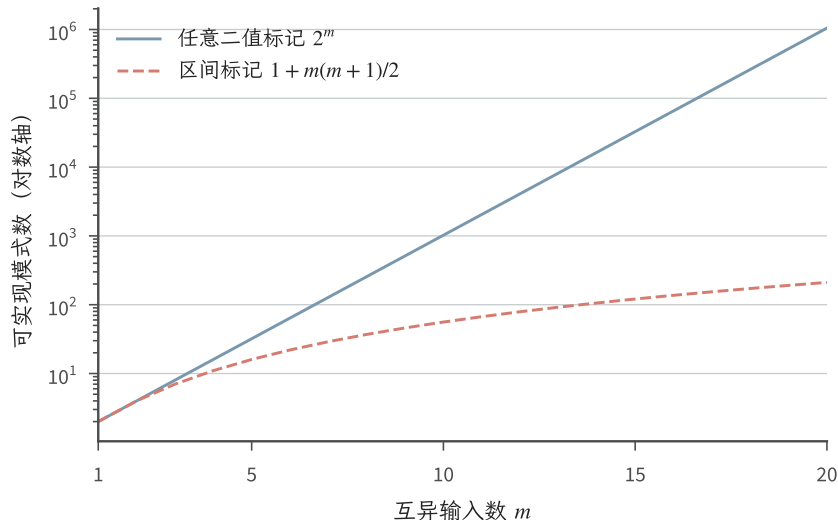
图 2.3 有限输入上的二值模式数（精确计数教学图）。蓝实线为不受限制的 2^m ，红虚线为实数轴区间分类器的 1 + m(m+1)/2 。纵轴使用对数刻度，红线是该具体类的精确计数；它也恰等于至多两个正类点的集合族计数，但两类实现的模式可以不同。
