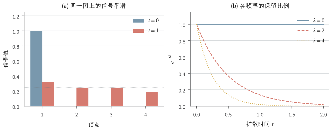
图 11.13 贯穿四顶点图的解析式扩散。左图比较 f(0) = (1, 0, 0, 0)^T 与 f(1) = e^{-L}f(0) , 灰虚线是最终均值 1/4 ; 右图绘制特征值 0, 2, 4 的保留比例, 4 的重数为 2 。柱和曲线直接由该图的拉普拉斯计算, 不表示实验均值或误差条。
