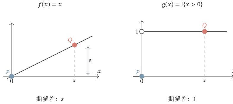
图 9.4 同一小位移对两种固定评价的影响。取 P = \delta_0 、 Q = \delta_\varepsilon 、 \varepsilon > 0 ，底层距离为绝对值。左图的 1-Lipschitz 函数 f(x) = x 变化 \varepsilon ；右图的事件函数 1\{x > 0\} 变化 1。横向位置仅作示意，结论对任意正的 \varepsilon 成立。
