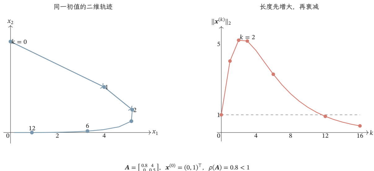
图 6.5 固定二维矩阵的反复作用。初值为 (0, 1)^\top ，前两步的长度增加，此后回到原点；右图将长度与初始长度 1 比较。特征值 0.8 和 0.5 决定长期衰减，非正交特征方向间的相消则决定早期放大。两图使用同一个矩阵和同一组迭代点。
