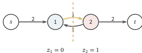
图 11.10 两变量能量的割表示，零容量弧省略。割把 s, 1 与 2, t 分开，因而标签为 z_1 = 0, z_2 = 1 。两个容量为 1 的反向弧中，仅源侧到汇侧的黄弧 1 \rightarrow 2 计费，成本不是 2。终端弧 s \rightarrow 1 的容量 2 = D_1(1) 只在顶点 1 进入汇侧时支付。
