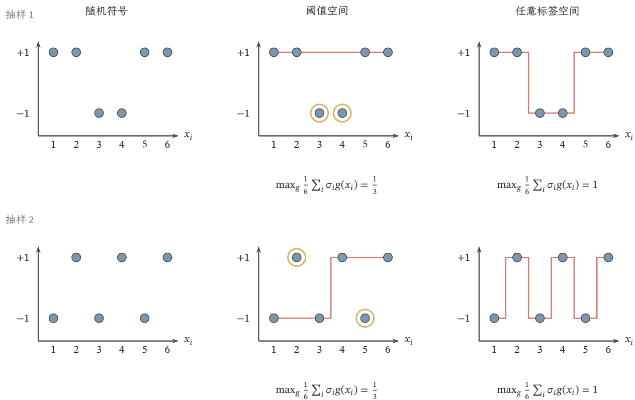
图 5.2 固定六个输入上的两次随机符号抽样。圆点表示 \sigma_i \in \{-1, 1\} ，其水平位置不变；中列曲线是取值为 \{-1, 1\} 的递增阈值函数，右列可在这六个点上任意赋值。暖色圈标出符号与中列函数不一致的点。两组示意符号下，阈值空间的最大相关得分均为 1/3 ，任意标签空间均为 1 。两个实现只展示逐组选择，经验 Rademacher 复杂度还要对全部 2^6 组等概率符号取平均；随机符号不是被改写的任务标签。
