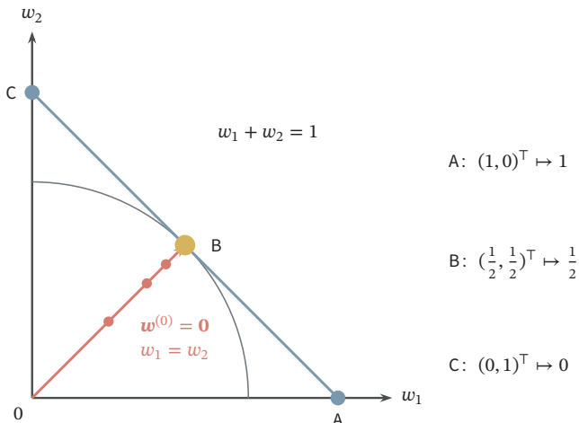
图 8.6 一个训练观测对应多个插值参数。直线上的 A、B、C 都使输入 (1, 1)^\top 的预测为 1，右侧列出它们对同一新输入 \mathbf{x}_{\text{new}} = (1, 0)^\top 的预测。对半平方损失从零初始化，图中以步长 1/4 画出前三次更新，轨迹趋向 B；细弧表示经过 B 的欧氏范数等值线，说明 B 是插值直线上距离原点最近的点。这个教学例子解释选解规则，不给出新输入的真实标签或泛化保证。
