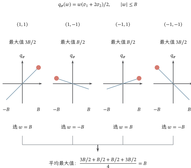
图 5.3 先最大化、再平均的经验 Rademacher 复杂度。固定教学输入 x_1 = 1, x_2 = 2 ，四幅小图分别对应等概率的四组随机符号；横轴为参数 w ，纵轴为得分 q_{\sigma}(w) ，各图共用尺度。圆点标出每组符号下的最大值，所选参数允许随符号改变；四个最大值的平均为 B 。这些符号独立于数据的真实标签，图中直线由得分公式计算得到。
