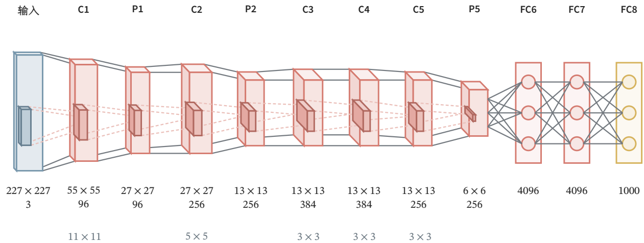
图 9.15 AlexNet 的五个卷积层与三个全连接层。全部主路径在一行展开，卷积层、最大池化层与全连接层分别绘出；最后一次池化的输出展平为 9216 维。各层下方给出空间尺寸和通道数，C 表示卷积，P 表示池化。此图采用 227 输入及正文给定的填充约定，省略局部响应归一化、Dropout 和原始双 GPU 的分组细节。
