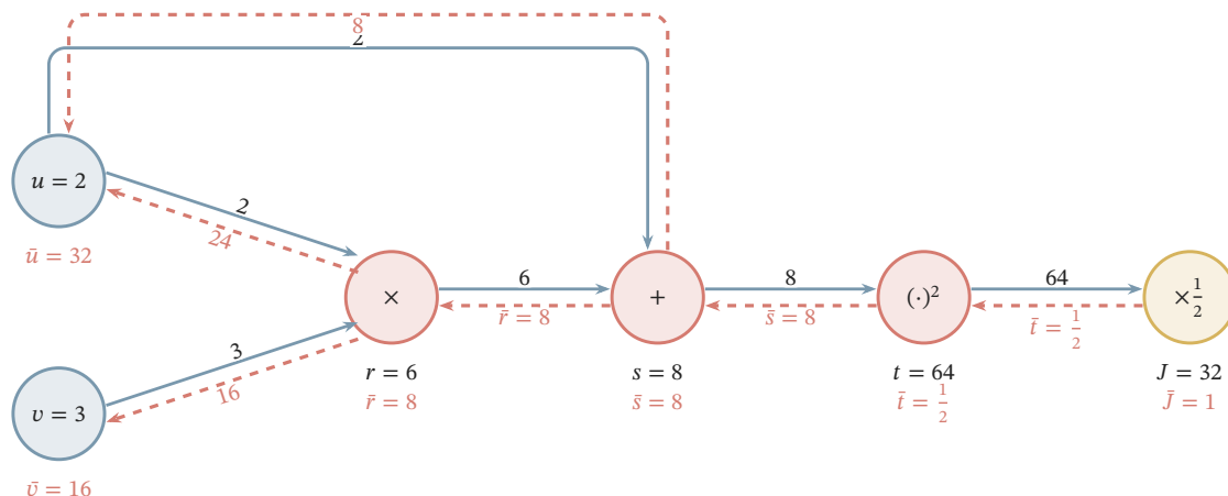
图 8.12 同一算子图上的后向模式。节点位置与前向模式相同，实线及其黑色标注保留前向传递值，红色虚线及其标注从 \bar{J} = 1 开始回传导数贡献；每个算子下方两行分别给出输出值和伴随值。输入 u 收到经乘法传来的 24 和直接经加法传来的 8，累加为 32；输入 v 得到 16。一次后向遍历同时得到两个偏导。
