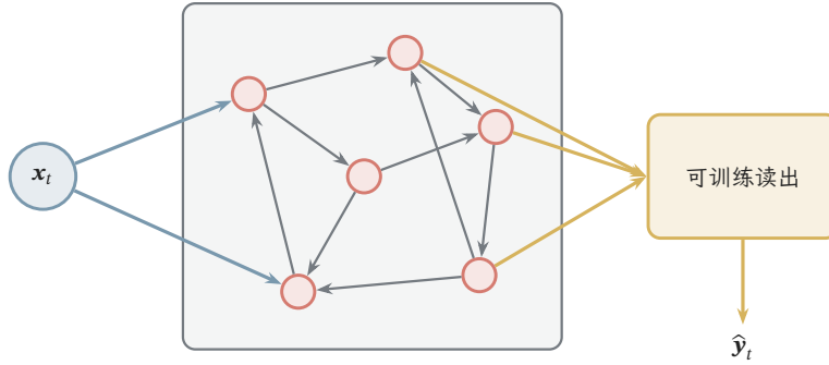
图 10.6 储备池计算的参数分工。输入进入固定的循环动态，多个内部单元共同形成随历史变化的状态，可训练读出将状态映射到目标。灰色连线表示固定连接，黄色箭头表示参与拟合的读出；内部连接只示意结构，不表示某个随机生成样本。ESN 使用连续值激活，LSM 可由脉冲活动及其滤波响应形成读出特征。
