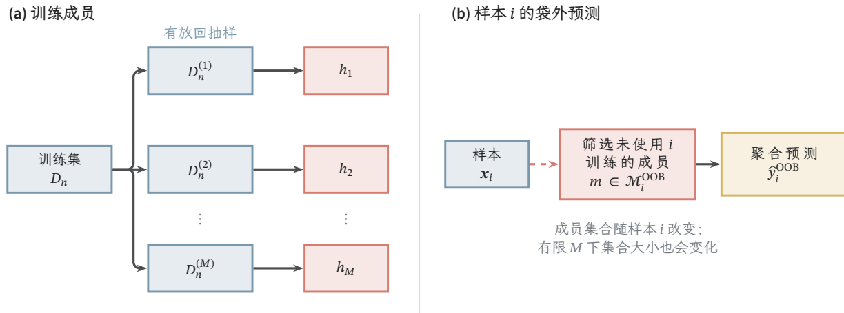
图 6.3 Bagging 训练与袋外预测。每个成员只使用其自助样本训练；对训练样本 x_i ，袋外预测只聚合未抽中 i 的成员。图中索引和成员集合仅用于说明数据流；有限成员下，各样本可用的袋外成员数并不相同。
