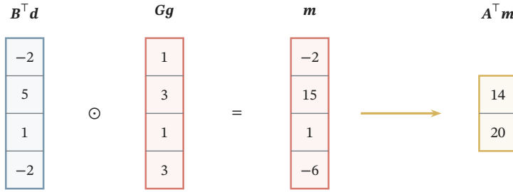
图 9.9 一维 F(2, 3) 的完整数值路径。输入 \mathbf{d} = (1, 2, 3, 4)^\top 与核 \mathbf{g} = (1, 2, 3)^\top 分别变为四个组合值，按位置相乘得到 \mathbf{m} = (-2, 15, 1, -6)^\top ，再用输出变换恢复两个互相关结果。四次核心乘法替代直接算法的六次乘法，加减与固定系数变换仍有成本。
