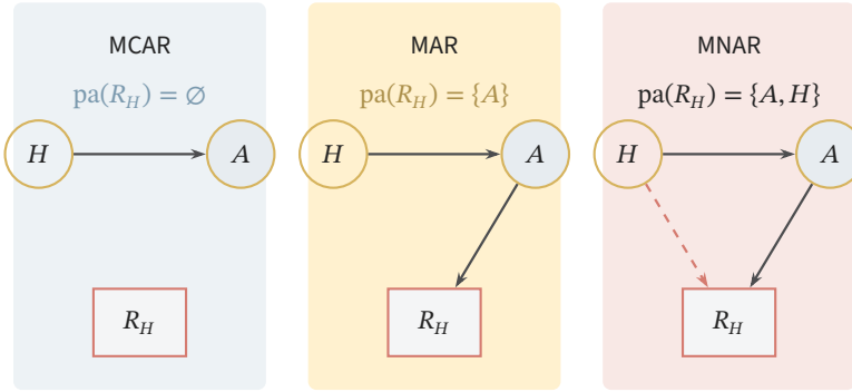
图 24.3 固定已观测的 F, S 后，温度记录指示量 R_H 的三种示意机制。三栏顶部直接给出 R_H 的父集，底部分别配独立日志故障、报警后安排检查、过热改变漏报概率的日常例子。 A 总是观测， H 在 R_H = 0 时不可见；右图需有实际的剩余依赖才属于 MNAR，单凭箭头存在不能排除参数抵消。
