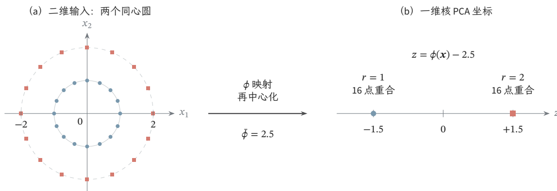
图 5.5 由核选择保留量的构造例子。左图在半径为 1, 2 的圆上各取 16 个等角度样本, 圆点与方点区分两圈。所示特制核对应标量特征 \phi(\mathbf{x}) = \|\mathbf{x}\|_2^2 , 中心化核矩阵秩为 1; 选择图示主轴方向, 核 PCA 坐标为 \pm 1.5 。右侧每个标记表示 16 点重合, 坐标无量纲。此结果依赖所选核, 不能推广为任意高斯核或多项式核的输出。
