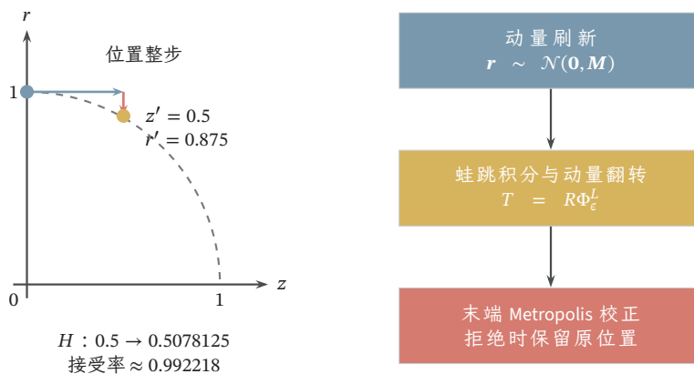
图 23.2 标准正态目标的一步 HMC 计算。左图中虚线圆弧属于 H = 1/2 的精确轨迹，折线表示 \epsilon = 0.5 的蛙跳位置整步与末端动量半步；初始动量半步因 z = 0 而不动。右图区分保持扩展分布的动量刷新与校正更新；末端动量翻转未画在相图上。
