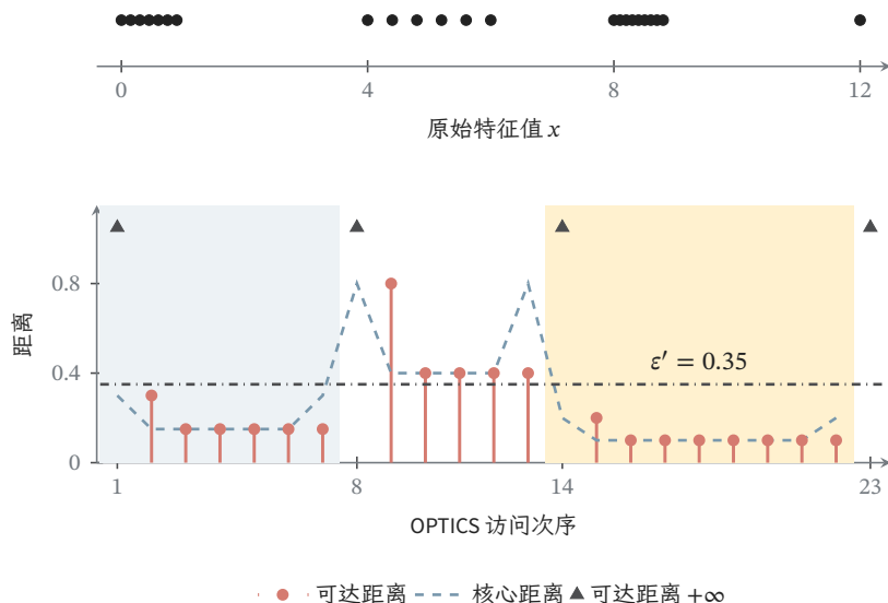
图 4.4 固定一维教学数据上的 OPTICS 排序，取 \text{MinPts} = 3 (含自身)、 \epsilon_{\max} = 1.1 。三组样本的间距分别为 0.15、0.4、0.1，另有 x = 12 的孤立点。红色竖棒为可达距离，蓝色虚线为核心距离；蓝、黄底色标出两个低谷。无穷可达距离用顶部三角形表示，不能按其显示高度作数值比较；水平点划线展示阈值切割在本例中提取哪些低谷。
