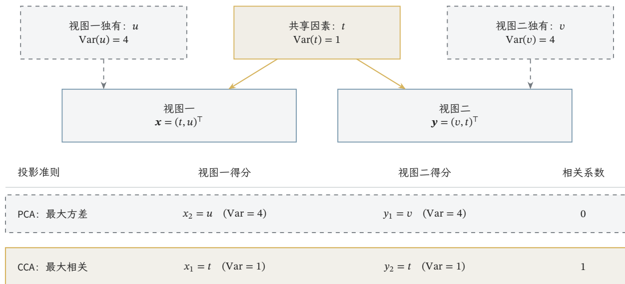
图 5.2 CCA 提取共有变化的构造例子。设 t, u, v 相互独立且均值为零, 方差依次为 1, 4, 4; 两视图为 \mathbf{x} = (t, u)^\top 和 \mathbf{y} = (v, t)^\top 。实线连接共享因素, 虚线连接各视图独有因素。各保留一维时, PCA 选择 u, v , CCA 选择 t, t , 对应相关系数分别为 0 和 1。箭头表示坐标构造关系, 图中结论针对给定总体, 不是样本拟合结果。
