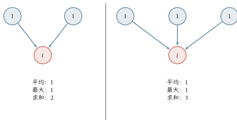
图 11.6 聚合如何保留或丢掉重复次数。两个邻域分别含两个和三个数值为 1 的邻居。平均与最大值都产生 1，求和分别产生 2 和 3。图只比较固定标量消息；求和本身也不能区分所有不同多重集，还需要合适的特征映射。
