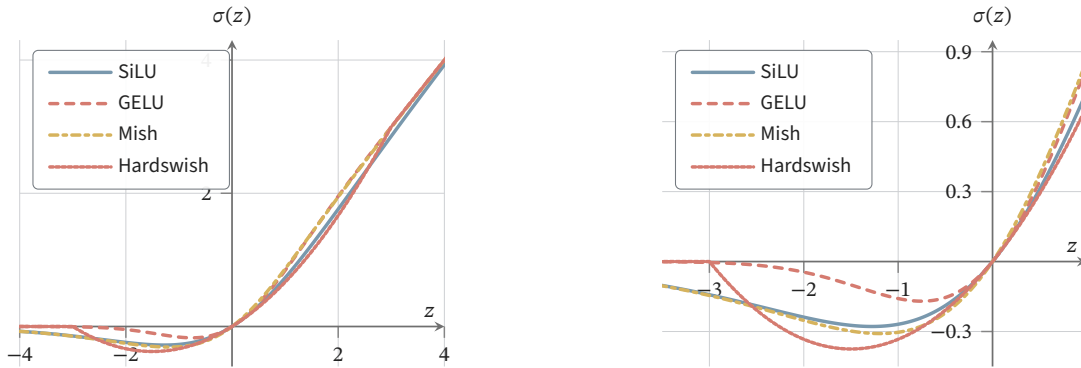
图 8.7 SiLU、GELU、Mish 与 Hardswish。左图展示整体响应，右图放大原点附近的负值和过渡区域；GELU 按标准正态累积分布函数采样。它们在正端接近线性，但负区间的形状和拐点不同。SiLU、GELU 与 Mish 平滑，Hardswish 含有分段边界；两图使用不同坐标标范围以显示细节。
