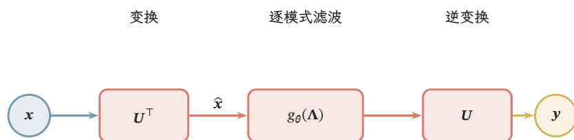
图 11.5 谱滤波的计算路径。节点信号 x 经 U^T 分解为图傅里叶系数，每个模式由 g_\theta(\lambda_k) 调整，再经 U 还原为节点信号。左、右两端使用同一张图和同一节点顺序；中间向量的下标表示频率模式。
