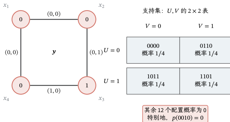
图 18.6 零概率破坏逆向分解的反例。左侧节点给出被禁止配置 \mathbf{y} = (0, 0, 1, 0) ，边旁的每个局部取值对都曾在正概率配置中出现。右侧 2 \times 2 支持表按 (U, V) 列出四个正概率配置，并直接标出其余 12 个配置概率为 0。若存在非负边势分解， \mathbf{y} 对应的四个边势值就必须都为正，其乘积也为正，与 p(\mathbf{y}) = 0 矛盾。
