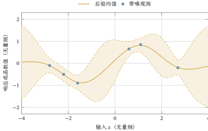
图 2.7 高斯过程的后验均值与函数不确定性。六个点为构造观测；先验均值为零，平方指数核取 \ell = 0.9 、 \sigma_f = 1 ，观测噪声标准差为 \sigma = 0.18 。实线为 \mu_* ，浅色带及虚线边界为 \mu_* \pm 1.96\sqrt{v_*} ，表示潜在函数值的逐点约 95% 后验可信区间。它不是整条函数的同时可信带；预测未来带噪响应时，方差还须加 \sigma^2 。
