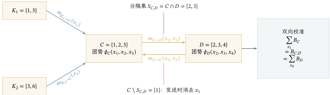
图 21.4 团间消息的组成与双向校准。蓝色箭头是 C 收到的入站消息, 团势与这些消息相乘后, 对 C \setminus S_{C,D} = \{1\} 中的 x_1 求和, 得到定义在分隔集 \{2, 3\} 上的 m_{C \rightarrow D} ; 发送时排除接收方 D 的入站消息。黄色双向箭头分别汇总树边两侧的贡献, 收集与分发都完成后, 两个团消去非共享变量所得的表均等于分隔集势 B_{C,D} 。
