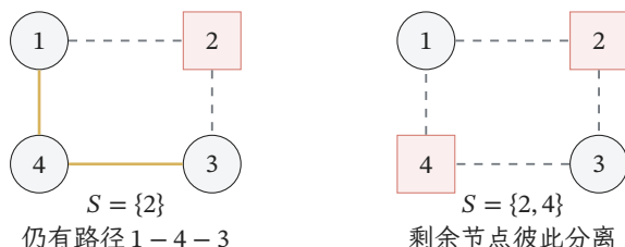
图18.4 删除条件节点以检测分离。方形节点属于 S ，虚线边随节点一同删除，实线边保留。左侧删除2后仍有路径 1-4-3 ；右侧同时删除2,4后，1与3处于不同连通分量。
