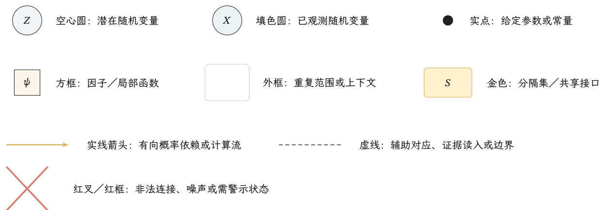
图 16.2 概率图模型部分的视觉约定。空心、填充和实点区分潜变量、观测变量与给定量；方框表示局部因子，金色强调团树分隔集或共享接口，红色表示非法或需警示的对象。实线箭头的概率语义与计算流语义由所在图决定；虚线只作辅助表达，不应在没有图注时自动解释为概率依赖。具体图内标注优先于本总图。
