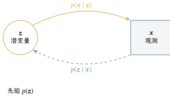
图 5.10 概率生成与后验推断的结构示意。实线表示 \mathbf{z} \rightarrow \mathbf{x} 的生成方向; 虚线表示 \mathbf{x} \rightarrow \mathbf{z} 的后验推断, 不是额外的生成依赖。图中节点与箭头只说明变量角色和条件关系, 不表示实测数据、网络层数或计算流程; 噪声描述观测对信号的偏离, 不是新增的潜变量维数。
