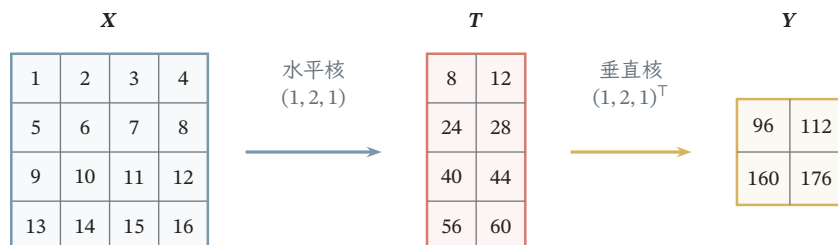
图 9.12 秩一空间核的两阶段计算。水平核与垂直核均为 (1, 2, 1) ，组成 3 \times 3 核 \mathbf{u}\mathbf{v}^\top 。在步长一、无填充条件下，原 4 \times 4 输入先变为 4 \times 2 中间结果，再变为 2 \times 2 输出。该小例子的两阶段核心乘法量仍为三十六次，图示验证的是结果等价，而非每种输入尺寸都能节省计算。
