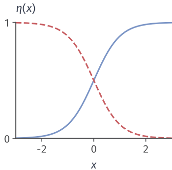
概念偏移
