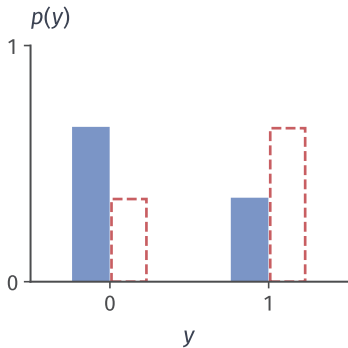
标签偏移
