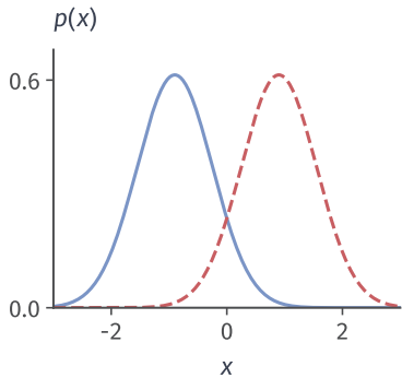
协变量偏移
