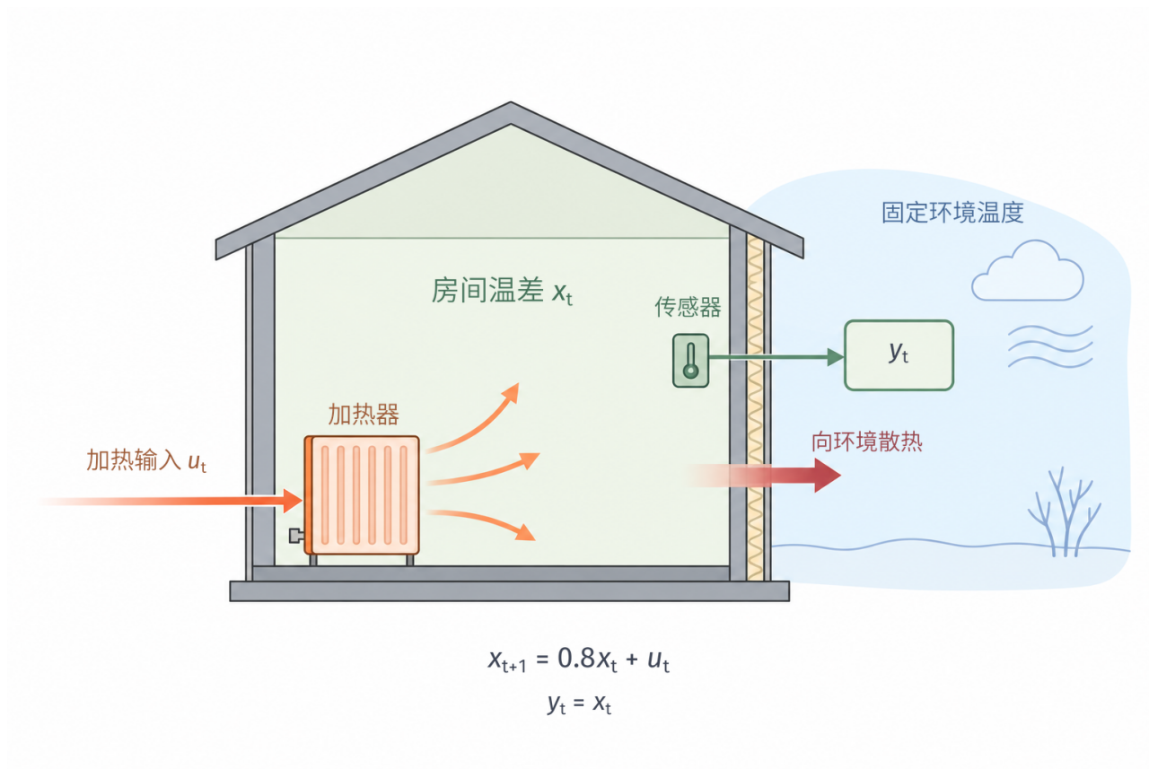
图 13.1 温度模型中的状态、输入与输出。环境温度固定时， x_t 表示房间相对环境的温差， u_t 表示给定加热输入，传感器在时刻 t 读取 y_t = x_t 。随后按 x_{t+1} = 0.8x_t + u_t 形成下一时刻温差；系数 0.8 表示未加热时保留下来的温差比例。图中没有根据读数选择输入的控制器的。
