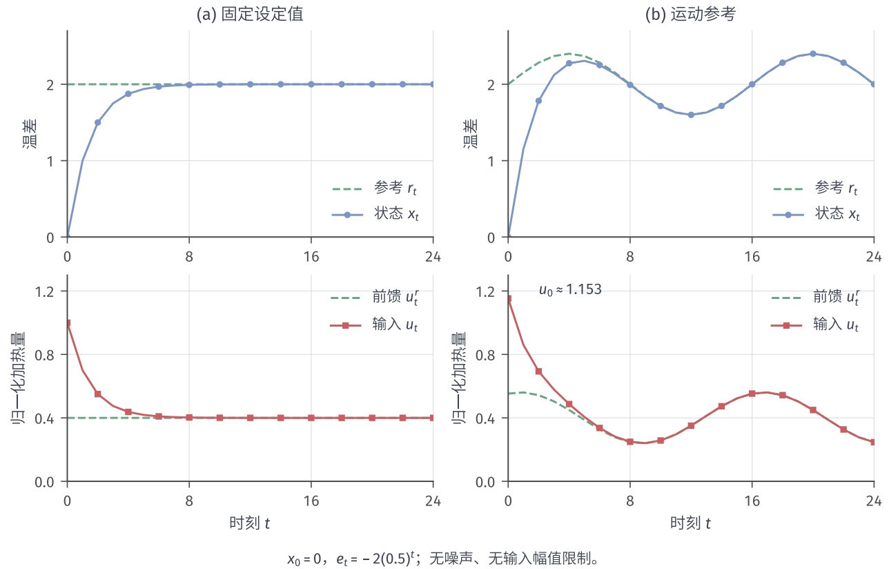
图 14.3 同一无噪声温度模型、初态 x_0 = 0 与误差增益 0.3 下的调节和跟踪。左列固定 r_t = 2 ，右列取 r_t = 2 + 0.4 \sin(\pi t/8) ；上排比较参考与实际状态，下排比较维持参考的前馈与完整输入。两种任务的误差均为 e_t = -2(0.5)^t ，但运动参考需要持续变化的前馈。图中输入无幅值限制，右下首个动作超过 1，因而此图不是受限执行器的安全证明。离散点之间连线仅便于阅读。
