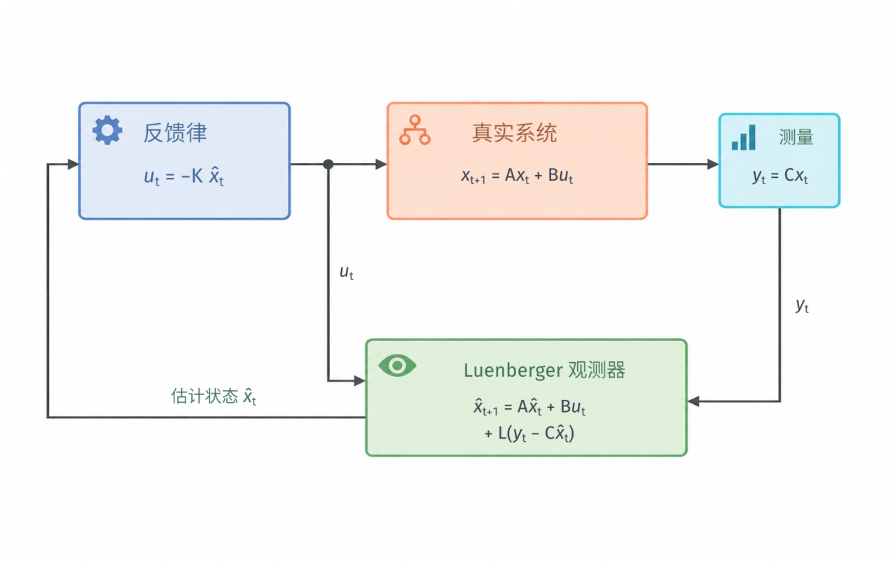
图 14.2 离散确定性 Luenberger 观测器的输出反馈。观测器同时接收 u_t 与 y_t ，用残差 y_t - C\hat{x}_t 修正估计，再由 u_t = -K\hat{x}_t 形成闭环。真实状态进入测量映射，不直接供给反馈律。 K 与 L 分别决定 A - BK 与 A - LC 的特征模态；这里没有随机 Kalman 增益更新。
