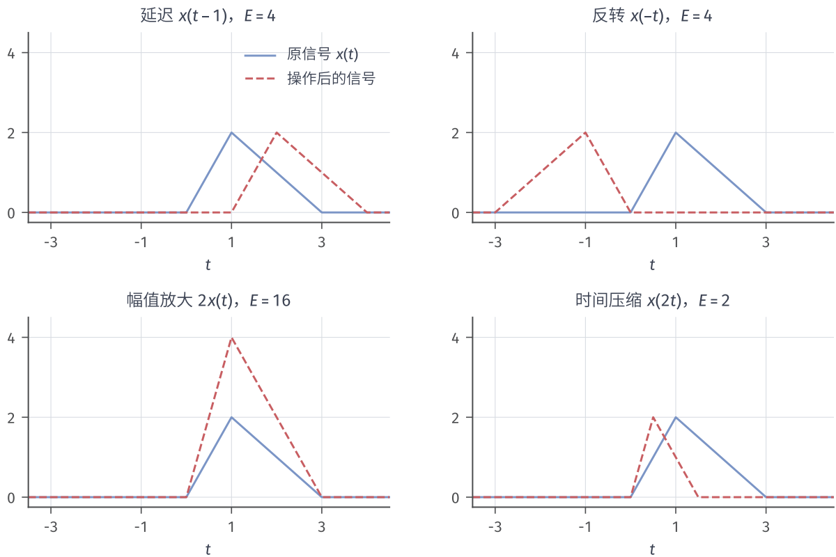
图 8.2 对同一非对称三角脉冲分别延迟、反转、放大幅值和压缩时间。每幅图的蓝线均为式 (8.14) 的原信号，红线为指定操作结果，横轴为时间、纵轴为幅值，坐标尺度一致。平移和反转保持整轴能量 4，幅值乘 2 使能量变为 16，时间压缩为一半使能量变为 2；各图均在整轴零值背景下观察，不作窗口裁剪。
