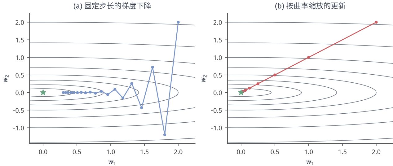
图 4.2 例 4.11 中的精确更新路径。灰线是同一二次目标的等值线，蓝、红圆点分别表示普通更新与预条件更新，星号是最小点。预条件使用了已知曲率，获得和应用这一矩阵的成本仍属于算法代价。
