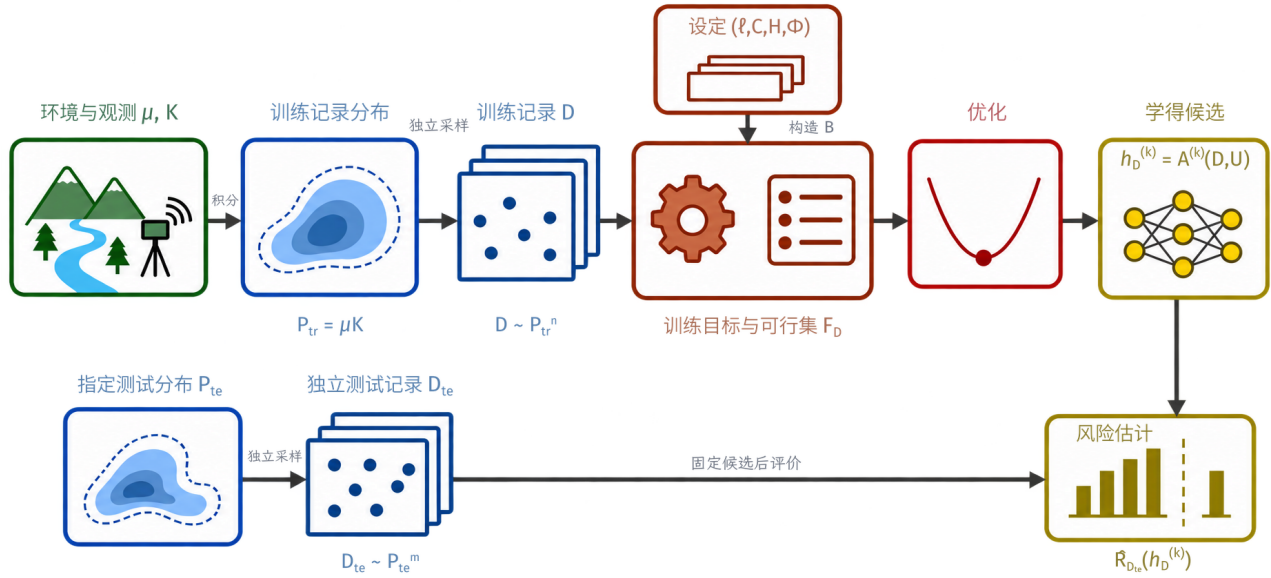
图 17.1 静态学习中的数据、目标与方法。图中取独立采样 Q_n = P_{tr}^n ； P_{tr} = \mu K 是分布运算， D \sim Q_n 是采样。目标构造 B 与优化规则共同组成学习映射 A 。固定学得候选后，独立测试记录用于估计指定测试分布下的评价风险。
