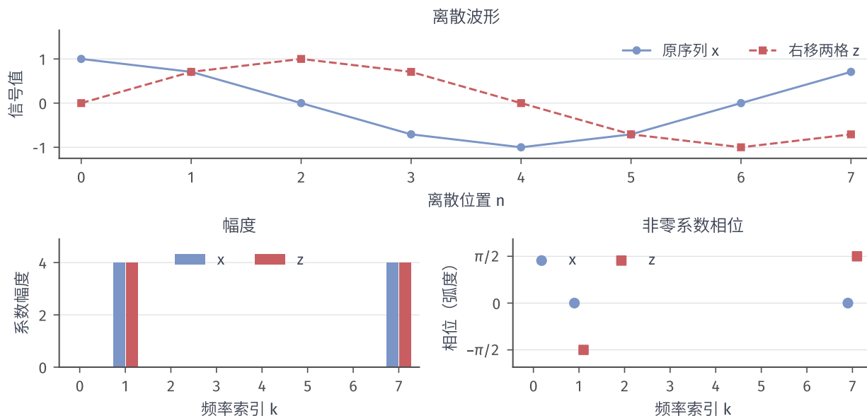
图 8.1 长度 8 的教学信号 x[n] = \cos(2\pi n/8) 及其循环延迟两格的结果。上方波形的峰值位置不同，下方在 k=1,7 的幅度均为 4，相位却改变。相位图只画非零系数；波形连线只帮助观察顺序，不表示已选择连续时间插值。
