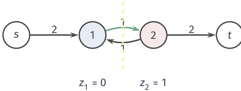
图 9.10 两变量能量的割表示，零容量弧省略。割把 s, 1 与 2, t 分开，因而标签为 z_1 = 0, z_2 = 1 。两个容量为 1 的反向弧中，仅源侧到汇侧的绿弧 1 \rightarrow 2 计费，成本不是 2。终端弧 s \rightarrow 1 的容量 2 = D_1(1) 只在顶点 1 进入汇侧时支付。
