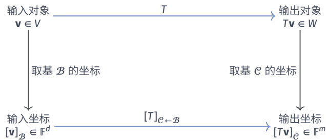
图 6.3 先作用于对象再取坐标，与先取输入坐标再乘矩阵，得到相同输出坐标。横向箭头改变对象或数值，竖向箭头只改变记录方式。
