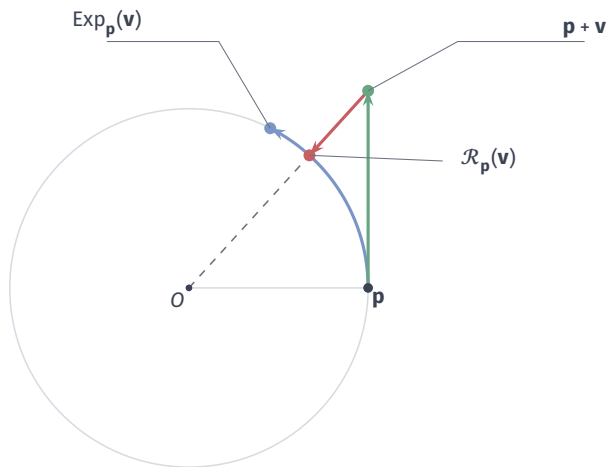
图 7.6 单位圆截面中的切向步、指数映射与归一化回缩。取 \mathbf{p} = (1, 0)^\top 、 \mathbf{v} = (0, 1.1)^\top 。箭头为切向步，终点 \mathbf{p} + \mathbf{v} 位于圆外；红色径向箭头将该点归一化为 \mathcal{R}_p(\mathbf{v}) 。从起点方向计，蓝色指数更新转过 1.1 弧度，归一化回缩转过 \arctan(1.1) \approx 0.833 弧度。两种更新关于步长的曲线在零步长处有相同初速度，但有限步位置不同。图为解析教学示例。
