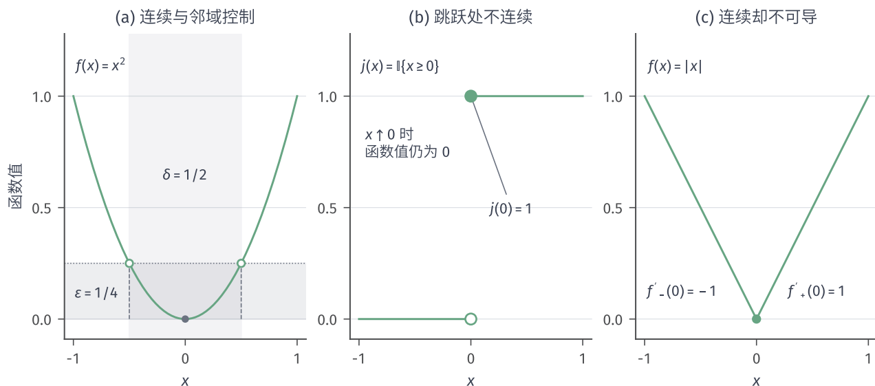
图 3.3 三个不同的局部性质。(a) f(x) = x^2 在 0 处可用 \delta = 1/2 控制 \varepsilon = 1/4 : 严格位于输入邻域内的点, 其函数值严格落在输出邻域内。(b) 阶跃函数在 0 的左极限为 0, 取值却为 1, 空心点和实心点区分两者。(c) |x| 在 0 处连续, 但左右导数分别为 -1 和 1 , 不存在共同的双侧导数。图中曲线均为解析教学示例。
