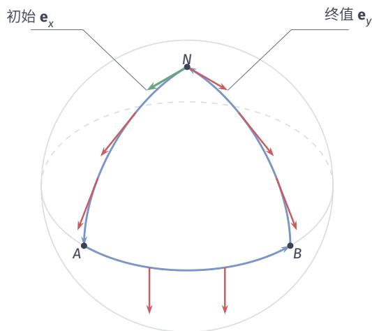
图 7.5 单位球面上沿 N \rightarrow A \rightarrow B \rightarrow N 的平行移动。蓝色为给定的三条大圆弧，红箭头为例 7.24 中逐段计算的切向量。沿路协变导数为零，返回 N 后的方向却由初始箭头 e_x 变为红色终值箭头 e_y 。箭头在三维中等长，投影到纸面后的长度可以不同。图为解析教学示例。
