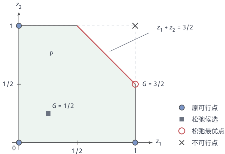
图 2.11 式 (2.27) 的精确可行域。浅色多边形为松弛范围 P ，蓝色实心圆点为原零一可行点，灰色方点的目标值仅为 1/2 ，红色空心圆点达到松弛最优值 3/2 ；右上角叉号为取整后不可行的 (1, 1) 。红色线段满足 z_1 + z_2 = 3/2 ，整个 P 都在该线的低值一侧。
