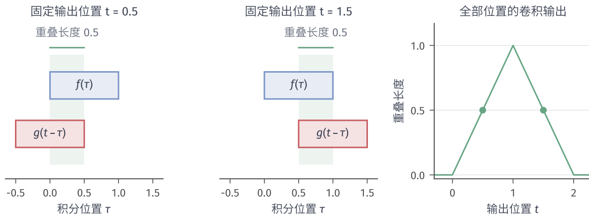
图 8.3 教学函数 f = g = \mathbb{I}_{[0,1]} 的连续卷积。左两图分别固定 t = 0.5 与 t = 1.5 , 蓝色为 f(\tau) 的支撑, 红色为 g(t-\tau) 的支撑, 绿色重叠区间的长度均为 0.5。右图汇总全部 t 处的重叠长度, 在 t = 1 时达到 1。左图横轴 \tau 用于积分, 右图横轴 t 标记输出位置。
