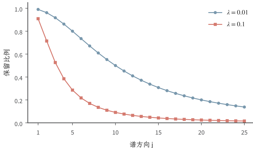
图 5.9 教学谱 \mu_j = j^{-2} 上的收缩比例 \mu_j/(\mu_j + \lambda) 。蓝、红线使用 \lambda = 0.01 和 0.1 ，点标出前 25 个方向；增大正则化后更多方向被抑制。有效维度的定义仍对全部谱方向求和。
