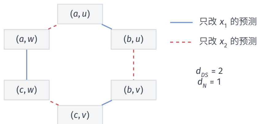
图 2.7 六模式族 \mathcal{V} 的逐坐标邻接。每个顶点是一种两输入预测；蓝实线只改变第一坐标，红虚线只改变第二坐标。每个顶点在两个方向上都有邻居，所以它构成二维伪立方体；图中没有固定两标签对形成的四角矩形，故其 DS 维为 2 而 Natarajan 维为 1。
