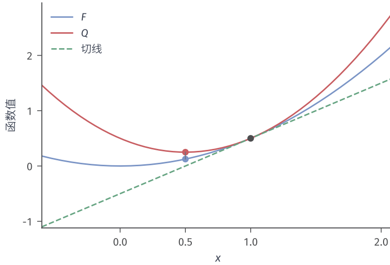
图 4.7 代理上界与切线的区别。蓝线为 F(x) = x^2/2 ，红线为当前点 1 处的主化代理 Q ，绿虚线为同点切线 x - 1/2 。三者在当前点同值同斜率，但切线位于目标下方，最小化它不能使用 MM 的上界链；红点标出代理最小点对应的值。图为解析教学示例。
