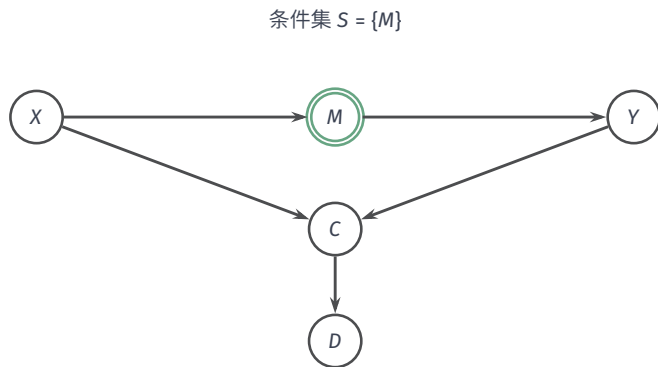
图 12.5 多条路径下的 d-分离。双边框节点 M 属于条件集，上方链式路径关闭；碰撞点 C 及其后代 D 都未给定，下方路径也关闭。若再把 C 或 D 加入条件集，下方路径就会打开，说明增加条件可能破坏原有的分离。
