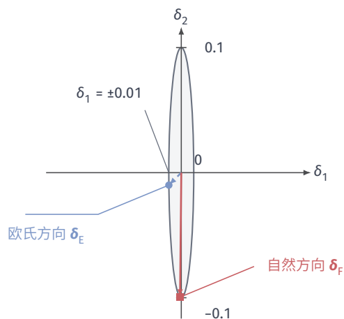
图 11.7 局部 KL 预算下的下降方向（解析式教学图）。灰色椭圆满足 100\delta_1^2 + \delta_2^2 = 0.01 ，对应 \varepsilon = 0.005 。蓝色虚线与圆点是缩放后的欧氏方向 \delta_E ，红色实线与方点是自然方向 \delta_F ；两个终点消耗相同的二次预算。椭圆表达分布变化代价，不是目标函数的等高线。
