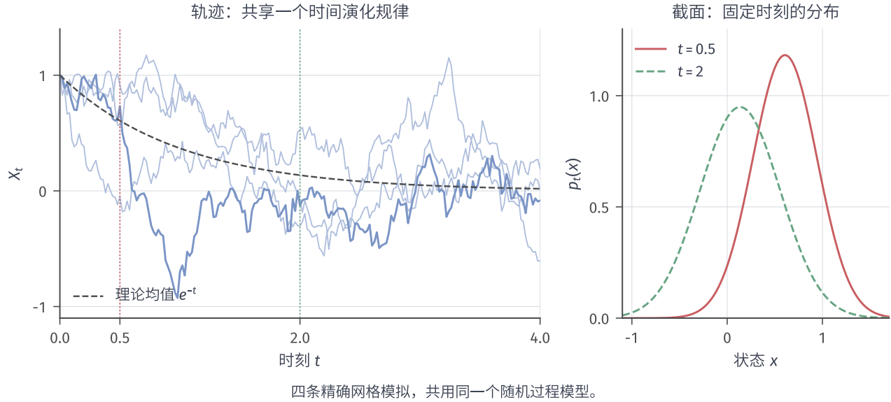
图 13.7 OU 模型的路径与截面。取 \lambda = 1, \sigma = 0.6, X_0 = 1 ，左侧为按精确高斯转移生成的四条网格轨迹与理论均值，右侧为 t = 0.5, 2 的解析边缘密度。折线只连接模拟网格点，不是可微的连续样本路径。截面给出单时刻概率，时间间的相关性还由共同噪声与转移决定。
