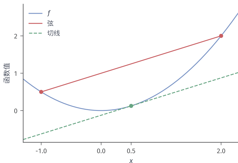
图 4.1 f(x) = x^2/2 的弦与切线。蓝线为函数，红线连接 u = -1 与 v = 2 的函数值，在这两个输入之间给出弦上界；绿虚线是在 x_0 = 1/2 处的一阶仿射下界，适用于整个实线。红线的上界只在其端点之间使用，切线下界来自凸性。图为解析教学示例。
