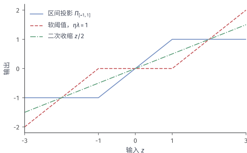
图 4.3 同一输入 z 的三种邻近映射。投影采用 C = [-1, 1] ；软阈值与二次收缩均取 \eta\lambda = 1 ，分别输出 \text{sign}(z)(|z| - 1)_+ 和 z/2 。横轴刻度标出阈值位置，曲线由完整分段解析式生成。
