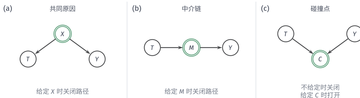
图 12.4 共同原因、中介与碰撞点的局部路径。双边框表示节点已加入条件集。共同原因和中介是非碰撞点, 给定后关闭这条路径; 给定碰撞点则打开原本关闭的路径。路径打开表示图不再保证相应独立性, 并不指定相关的大小或正负。
