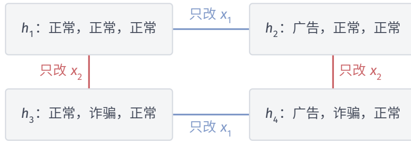
图 2.6 Natarajan 打散的四种预测。每个框中的三项依次对应 x_1, x_2, x_3 ；横向只改变 x_1 ，纵向只改变 x_2 ，而 x_3 始终预测为正常。每个输入处的两个标签预先固定，四个函数实现全部二选一组合。
