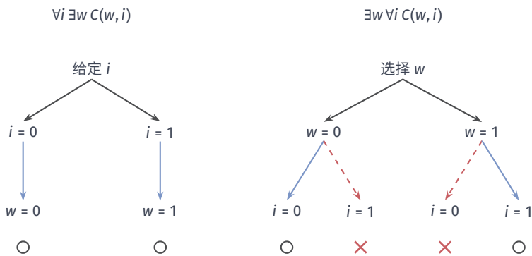
图 1.3 固定 S = W = \{0, 1\} 和条件 C(w, i) \Leftrightarrow (w = i) ，只改变量词次序。左侧每个 i 分支分别选到合格的 w ，故 \forall i \exists w C(w, i) 成立。右侧无论先选哪个 w ，其下两个 i 分支总有一个失败，故 \exists w \forall i C(w, i) 不成立。圆形标记表示条件成立，叉形标记表示条件不成立；右侧的虚线标出失败分支。
