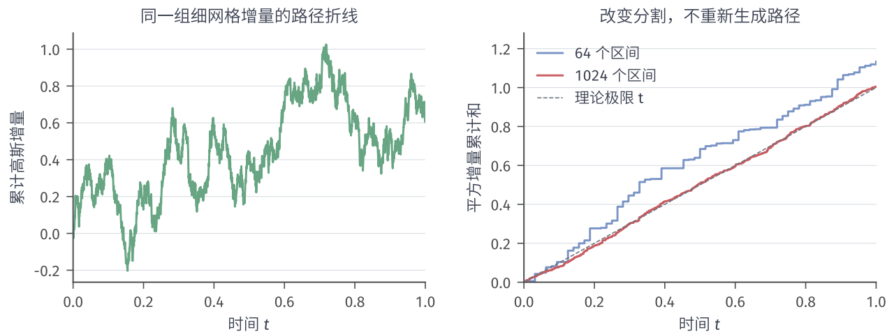
图 10.9 以固定随机种子构造的高斯增量教学例。左图由 4096 个独立增量 \Delta W_i \sim \mathcal{N}(0, 1/4096) 累计成路径折线；右图将同一组增量分别合并为 64 和 1024 个时间区间，再累计各区间增量的平方。蓝、红阶梯线使用不同分割，灰色参考线为理论二次变差 t 。这里只绘制有限网格，不把某一条折线作为连续布朗路径或收敛证明。
