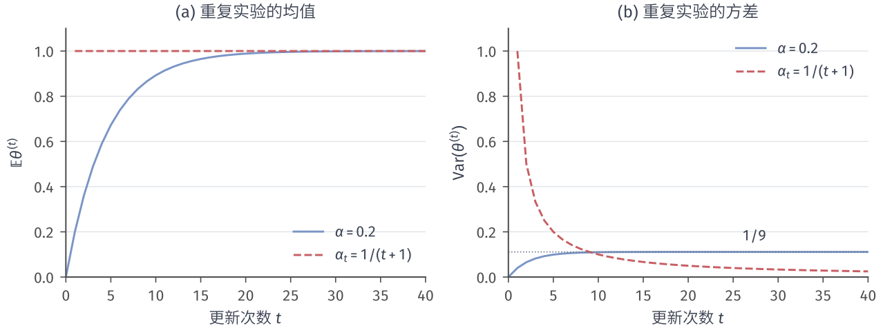
图 13.6 同一均值问题的重复实验均值与方差。取 \theta^{(0)} = 0, \mu = 1, \sigma^2 = 1 , 观测独立同分布; 蓝实线为固定 \alpha = 0.2 , 红虚线为 \alpha_t = 1/(t+1) 。固定步长方差趋于 1/9 , 样本平均方差为 1/t 。曲线由解析式得到, 不是一条样本轨迹。
