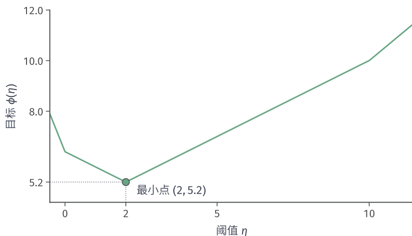
图 15.1 教学分布 P(L=0)=0.6 、 P(L=2)=0.3 、 P(L=10)=0.1 在 \alpha=0.75 下的阈值目标 \phi(\eta) = \eta + 4\mathbb{E}[(L-\eta)_+] 。绿色折线的最小点为 (2, 5.2) ; 阈值 2 与尾部平均 5.2 不能混用。
