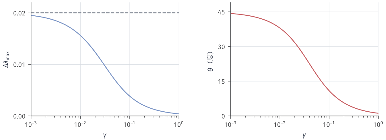
图 6.9 同一对称扰动下，谱值稳定不等于方向稳定，固定 \epsilon = 0.02 。左图为最大特征值增量 \Delta\lambda_{\max} = \sqrt{(\gamma/2)^2 + 0.02^2} - \gamma/2 ，灰虚线为扰动范数 0.02；右图为最大特征方向转角 \theta = \frac{1}{2} \arctan(0.04/\gamma) ，角度用度表示。两图横轴均为原始谱隙 \gamma ，采用相同的对数刻度。所有数值均来自二阶特征方程的解析解。
