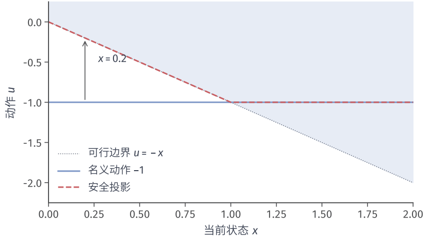
图 14.5 教学积分器 \dot{x}_t = u_t 、安全集合 x \geq 0 及 \alpha(h) = h 。灰色虚线 u = -x 上方为允许动作；蓝色实线为名义动作 u = -1 ，红色虚线为投影 u^* = \max\{-1, -x\} 。 x \geq 1 处无需修正， x = 0.2 处修正为 -0.2 。图中没有额外执行器限制，不能据此判断有限输入范围下的联合可行性。
