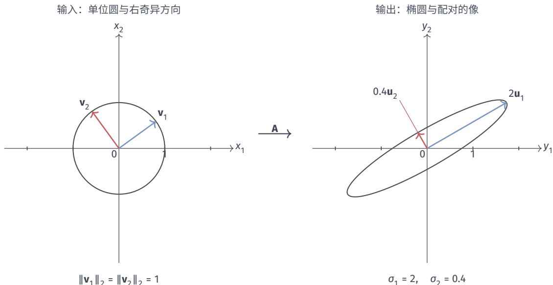
图 6.6 矩阵 \mathbf{A} = \mathbf{R}(\pi/6) \text{diag}(2, 0.4) \mathbf{R}(\pi/5)^\top 将单位圆变为椭圆。蓝、红箭头分别标出右奇异方向 \mathbf{v}_i 及其像 \sigma_i \mathbf{u}_i ；两侧坐标比例相同。奇异值决定长度变化，左右方向可以不同，因而这不是沿特征方向的空间缩放。图为教学构造。
