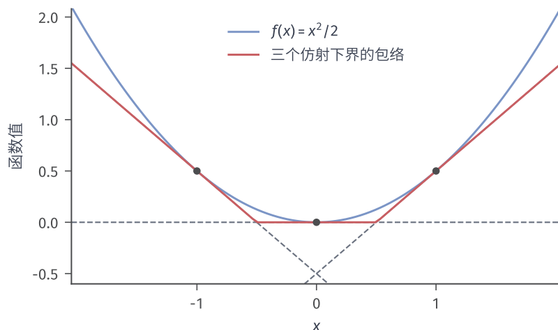
图 4.4 f(x) = x^2/2 与斜率 y = -1, 0, 1 对应的仿射下界 \ell_y(x) = yx - y^2/2 。蓝实线为抛物线，三条灰虚线为下界，红实线为这三条下界的逐点最大值。三个实心点标出相切位置；有限个斜率留下的间隙，在取全部斜率的上确界时消失。图为解析教学示例。
