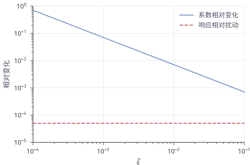
图 6.8 近共线矩阵的精确敏感性。固定 \mathbf{y}_0 = (2, 0)^\top ，扰动为 (0, 10^{-4})^\top ；红线是响应相对扰动 5 \times 10^{-5} ，蓝线是系数相对变化 10^{-4}/(\sqrt{2}\varepsilon) 。双对数坐标显示列越接近，反求系数越敏感；图中没有数值求解误差。
