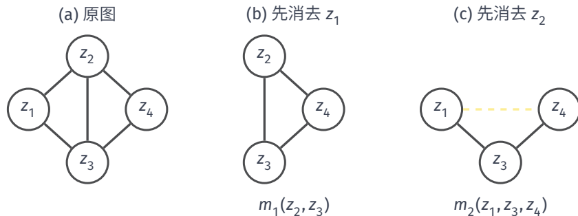
图 9.6 两个首步消元产生不同接口。删去 z_1 后，新表索引 (z_2, z_3) ；删去 z_2 后，通常须索引 (z_1, z_3, z_4) ，黄虚线为填充边 1—4。二值稠密接口表分别有 4 和 8 项，虽然两张余图都只剩三个顶点。特殊函数可能还能分解；图给出的是通用作用域范围。
