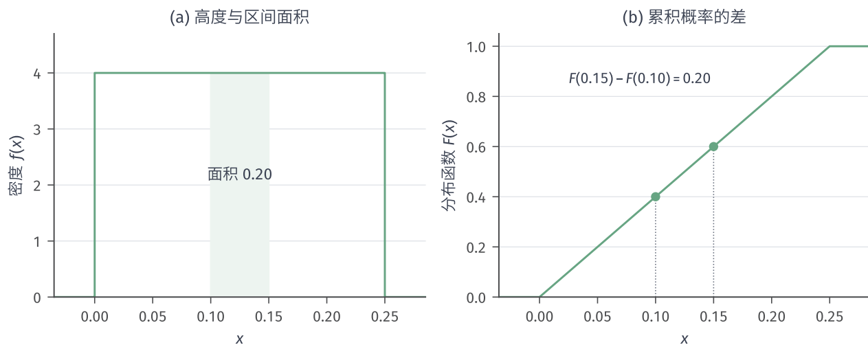
图 10.2 区间 [0, 1/4] 上的均匀分布（解析式教学图）。左图阴影为 [0.10, 0.15] 的概率 0.20，密度高度为 4；右图的概率是 F(0.15) - F(0.10) ，两个端点本身均没有正概率质量。
