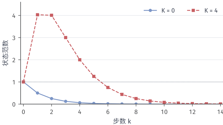
图 13.3 同谱系统的不同瞬态. 初值均为 (0, 1)^\top , 蓝色圆点取 K = 0 , 红色方点取 K = 4 , 谱半径均为 1/2 . 后者前两步范数约为 4.03、4.01, 随后才趋零; 灰线为初始范数 1. 长期衰减不等于每一步都收缩.
