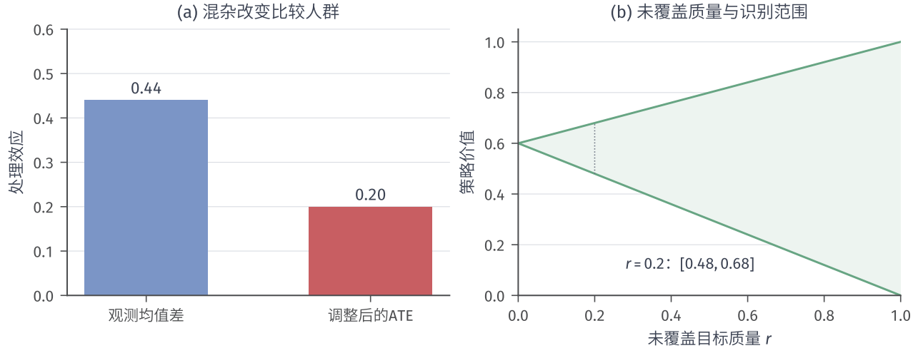
图 12.3 两个独立的教学构造。左图比较风险分层例子的观测均值差 0.44 与调整效应 0.20。右图按式 (12.31) 绘制 [0.6(1-r), 0.6(1-r)+r] 。阴影为总体识别范围，不是抽样置信带；两个面板不表示同一数据集。
