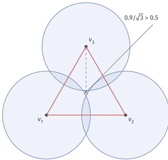
图 7.1 固定同组三点比较共同交集与成对条件。正三角形边长 0.9, \varepsilon = 1 , 蓝色开球半径 0.5; 红色边满足两种构造的连边条件。三球无共同交点, Čech 不含二维面, Rips 含二维面。中心到各顶点的距离为 0.9/\sqrt{3} > 0.5 。圆周只标开球边界, 图为解析教学构造。
