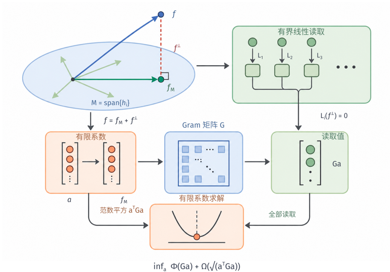
图 5.8 有限读取下的表示与求解。有界线性泛函 L_i 在 Hilbert 空间中有 Riesz 表示元 h_i 。所有读取只依赖 M = \text{span}\{h_i\} 中的分量 f_M ，单调不减的范数惩罚允许删去 f^\perp 而不增大目标。写 f_M = \sum_j a_j h_j 后，读数与范数平方分别为 Ga 与 a^T Ga 。有限表示不单独保证最优解存在或系数唯一；下方曲线只示意求解操作，不规定目标形状。
