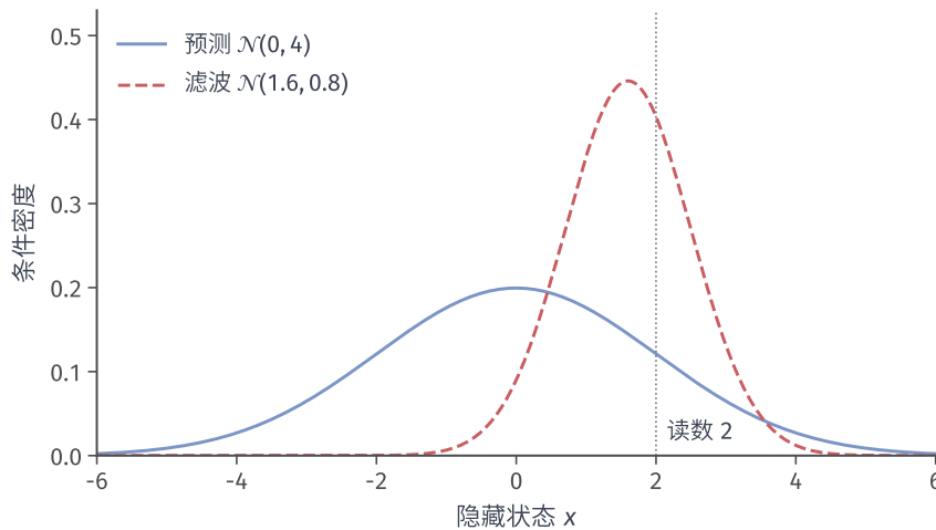
图 13.8 独立标量教学例的预测 \mathcal{N}(0, 4) 与后验 \mathcal{N}(1.6, 0.8) ，实际读数 y = 2 、观测噪声方差 1。第二个高斯参数是方差；本图不是贯穿温度模型的参数设定。
