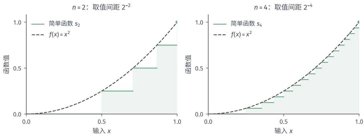
图 3.6 按取值分层的简单函数逼近。两图都使用式 (3.33) 的构造，分别取 n = 2 和 n = 4 ；本例中高度截断不起作用。绿色阶梯下的面积是有限加权和，目标曲线下的面积为 1/3 。两图共用坐标尺度。
