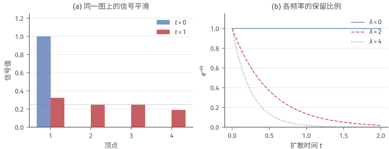
图 9.13 贯穿四顶点图的解析式扩散。左图比较 \mathbf{f}(0) = (1, 0, 0, 0)^T 与 \mathbf{f}(1) = e^{-L}\mathbf{f}(0) ，灰虚线是最终均值 1/4 ；右图绘制特征值 0, 2, 4 的保留比例，4 的重数为 2。柱和曲线直接由该图的拉普拉斯计算，不表示实验均值或误差条。
