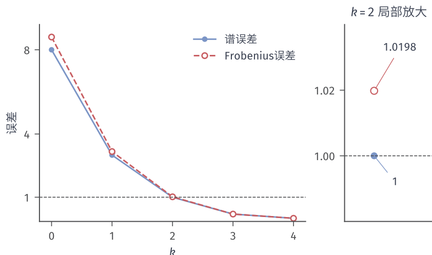
图 6.7 固定奇异值 (8, 3, 1, 0.2) 的最优误差曲线。给定横轴的秩可读出最低误差；给定水平误差阈值则寻找第一个满足要求的整数秩。 \tau = 1 时，蓝色谱误差在 k = 2 达标，红色 Frobenius 误差要到 k = 3 才达标。连线只辅助阅读，可行秩为整数。
