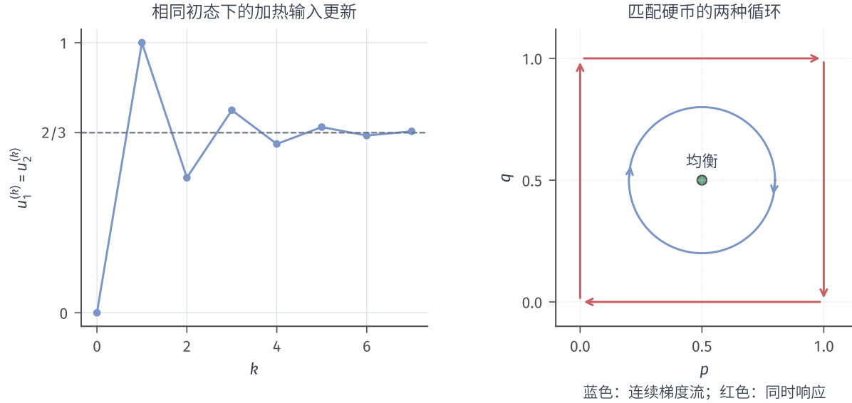
图 16.4 两个已明确更新规则的教学轨迹。左图为相同初态下双加热器的同时最佳响应，从 u_1^{(0)} = u_2^{(0)} = 0 开始，两条输入曲线重合，误差交替减半并趋向 2/3 。右图红色方形箭头是匹配硬币的离散四周期，蓝色圆是内部连续梯度流从 (p, q) = (0.8, 0.5) 出发的闭轨道，中心标记是 Nash 均衡。圆与方形对应不同更新，均不是最佳响应对应图中的静态集合。
