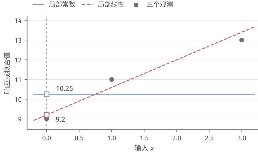
图 10.11 边界处的局部常数与局部线性拟合（教学数据图）。观测为 (0, 9), (1, 11), (3, 13) ，权重为 1, 0.75, 0.25 。蓝实线为加权常数 10.25 ，红虚线为 9.2 + 1.4x ，边界 x_0 = 0 处分别预测 10.25 和 9.2 。
