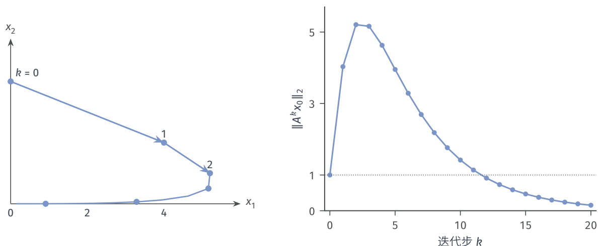
图 6.5 固定二维矩阵的反复作用。初值为 (0,1)^\top ，前两步的长度增加，此后回到原点；右图将长度与初始长度 1 比较。特征值 0.8 和 0.5 决定长期衰减，非正交特征方向间的相消则决定早期放大。两图使用同一个矩阵和同一组迭代点。
