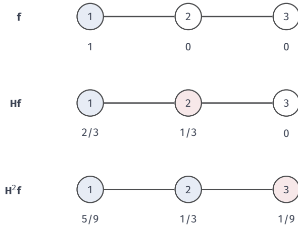
图 9.12 三顶点路径上的一次与二次局部滤波。顶点下方为精确值，白色表示零值，浅蓝表示此前已非零的顶点，浅红表示本步新到达的顶点；初始非零点也用浅蓝标出。颜色不编码连续色标。图的边均为单位权无向边，没有时间箭头；从上行到下行表示反复作用 H = I - L/3 。两步结果的算子是二次多项式，能到达两跳邻居。
