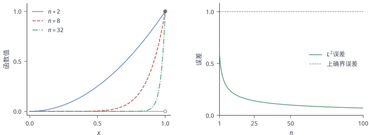
图 3.7 x^n 在 [0, 1] 上的两种整体尺度。左图蓝、红、绿线分别取 n = 2, 8, 32 ；灰线与端点标记表示逐点极限，它在 x < 1 处为零、在 x = 1 处为 1。右图绿色曲线为精确的 L^2 误差 (2n+1)^{-1/2} ，灰虚线为始终等于 1 的普通上确界误差；单点 x = 1 的修改不影响积分。图为解析教学示例。
