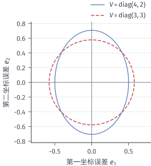
图 10.13 二维设计的归一化误差几何(解析式教学图)。蓝实线为 \mathbf{e}^T \text{diag}(4, 2)\mathbf{e} = 1 ，红虚线为 \mathbf{e}^T \text{diag}(3, 3)\mathbf{e} = 1 。它们不是已经具有相同覆盖概率的数值置信区间；真实置信半径由式(10.62)另行确定。
