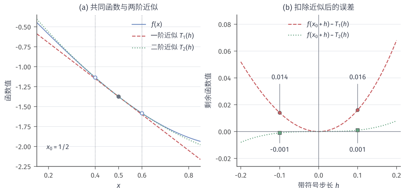
图 3.4 统一函数 f(x) = x^3 - 3x 在 x_0 = 1/2 处的两阶近似，记 h = x - x_0 。(a) 蓝线为真函数，红虚线为切线近似 T_1 = f(x_0) + f'(x_0)h ，绿点线加入二次项 f''(x_0)h^2/2 ，得到 T_2 。(b) 扣除各近似后的带符号余项分别为 3h^2/2 + h^3 与 h^3 ，标出 h = \pm 0.1 的精确结果。一阶导数确定切线，二阶导数补充局部曲率；余项的正负表示真值位于近似值的哪一侧。图为解析教学示例。
