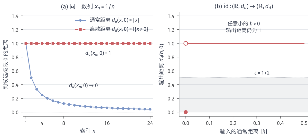
图 3.2 数值相同，距离不同。图中 d_u, d_d 分别对应正文的通常距离 d_1 与离散距离 d_2 。(a) 数列 x_n = 1/n 到 0 的通常距离趋于零，离散距离却恒为 1，所以收敛要连同度量说明。(b) 恒等映射从通常度量空间映入离散度量空间时，任意非零且很小的输入位移仍对应输出距离 1，不能进入 \varepsilon = 1/2 的输出邻域，故它在 0 处不连续。图为解析教学示例。
