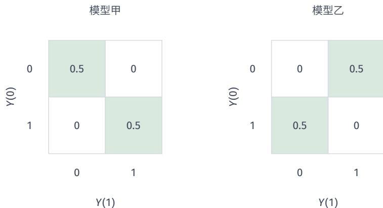
图 12.2 相同干预边缘的两种跨世界配对。行对应 Y(0) ，列对应 Y(1) ，格内数字为联合概率；每张表的行和、列和均为 1/2 。甲的个体效应恒为零，乙的个体效应等概率取 1, -1 ，两者 ATE 均为零。这是相容机制的教学构造，不是随机试验直接观察到的潜在结果联合表。
