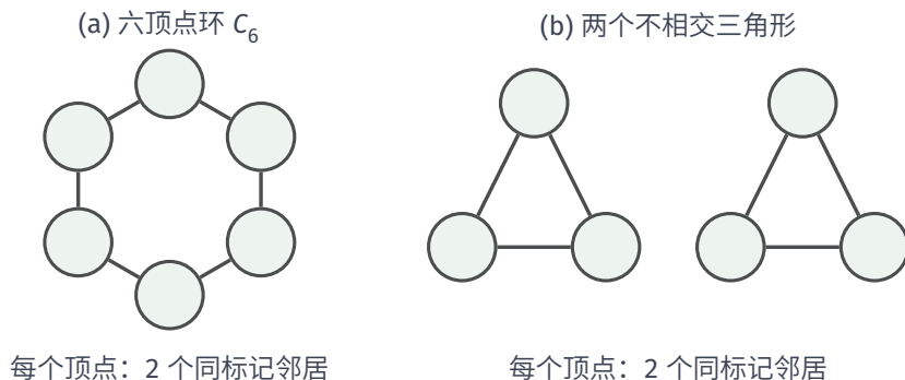
图 9.14 同样的邻居标记计数可以来自不同全局结构。两张六顶点图初始同标记，每轮每点仍见到两个同标记邻居，故 1-WL 计数无法区分一条六环与两个三角形。这不表示连通性难计算，而是说明该细化遗漏了这一差异。浅绿只表示共同标记，不加入唯一编号，以保持无标记图的比较设定。
