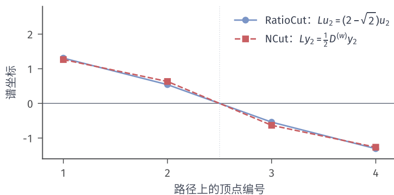
图 9.11 单位权四顶点路径的两种谱方向。蓝实线为组合拉普拉斯第二特征向量, 红虚线为度加权广义特征向量, 点形也作区分。显示时均按欧氏范数 2 缩放, 不替代 NCut 的度加权范数。横轴为四个离散顶点, 连线仅引导阅读; 竖虚线标出零阈值分割, 两种方向虽同号分组, 相对幅度并不相同。
