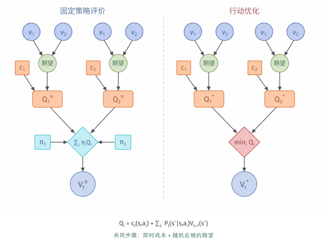
图 15.5 成本口径下的两种 Bellman 递推。两边都先将即时成本与随机后继价值的期望相加；固定策略评价再按 \pi_t(a | s) 平均，最优递推则在允许行动之间取最小值，不能把行动最小化移到随机后继状态上。图中 c_i = c_t(s, a_i) 、 \pi_i = \pi_t(a_i | s) ； v_1, v_2 是下一时刻两个后继状态的价值，左侧使用 V_{t+1}^\pi ，右侧使用 V_{t+1}^* ，不暗示两边数值相同。有限时域边界为 V_H = c_H ，此处没有折扣系数。
