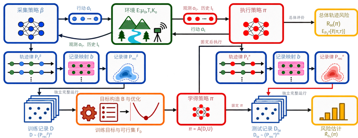
图 17.2 同一环境中的交互学习及其分布、记录与评价。采集策略 \beta 与执行策略 \pi 分阶段接入同一个环境, 行动返回环境, 观测 o_t 进入历史 I_t 。记录分布由轨迹律经记录映射 b 推前得到。图示取完整运行之间独立, 固定学得策略后重新采集测试轨迹, 且轨迹损失可由可见记录计算。总体轨迹风险由期望定义, 独立测试记录给出相应的样本风险估计。
