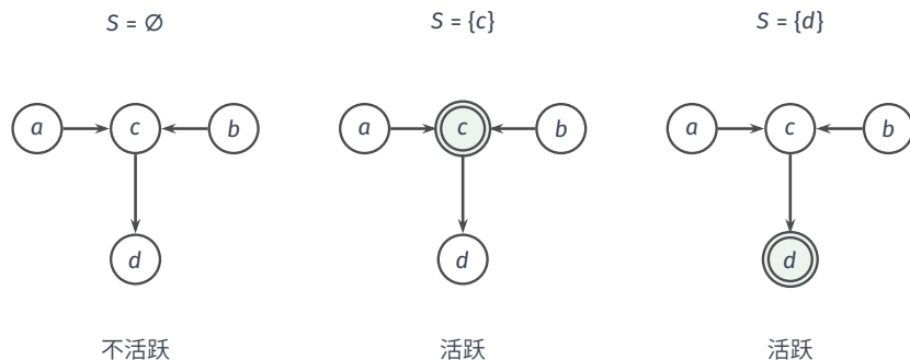
图 9.3 同一底层路径 a-c-b 在三个条件集下的活跃性。箭头及顶点没有改变；空条件集未打开碰撞点，给定碰撞点 c 或其后代 d 都会打开它。双圈表示被给定的顶点，底部文字给出判定。活跃性不是沿箭头从 a 走到 b 的可达性，也不是简单删除条件顶点后的连通性。
