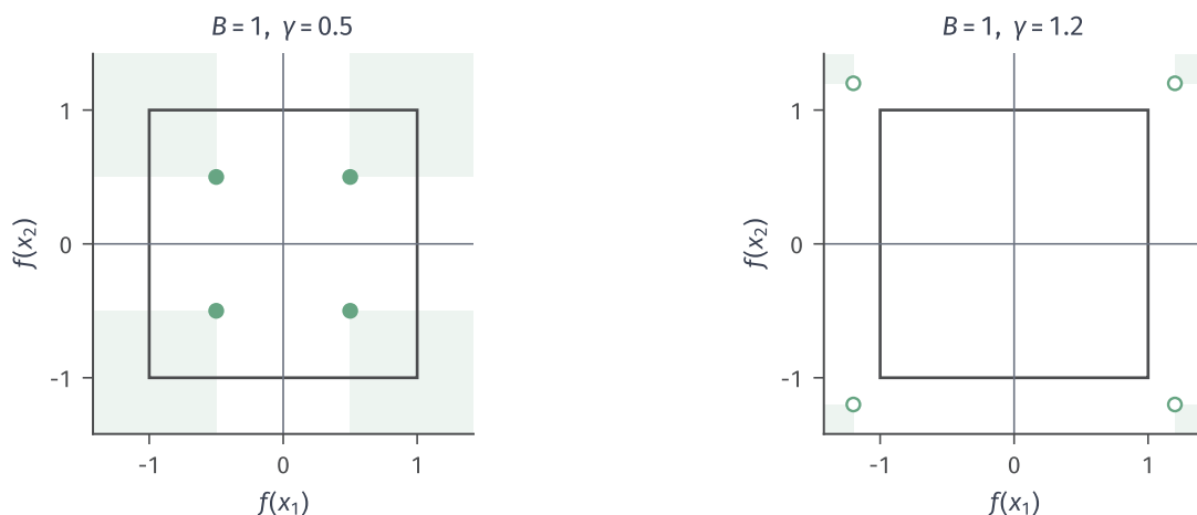
图 2.9 两个分块、 B=1 与固定阈值 r_1=r_2=0 的输出几何。灰框是函数类允许的 (f(x_1), f(x_2)) \in [-1, 1]^2 ; 浅绿区域要求两坐标分别离阈值至少 \gamma 。左图 \gamma=0.5 的四种符号可由实心点实现; 右图 \gamma=1.2 的空心点只标出要求的边界, 全部落在允许框之外, 因而不是类中的函数输出。图为解析教学构造。
