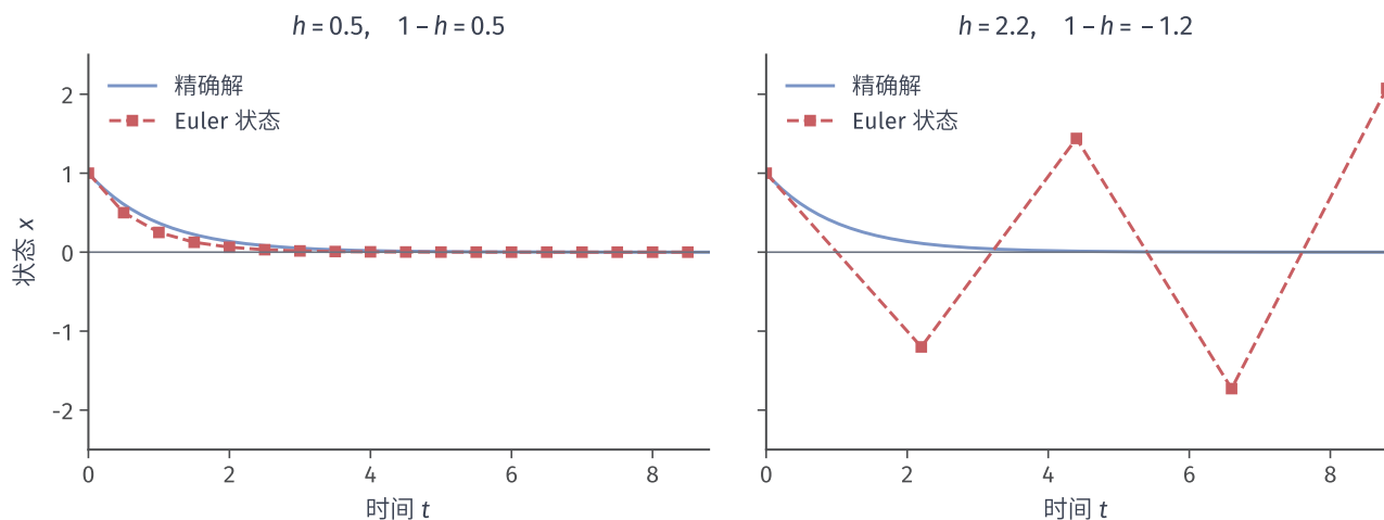
图 13.2 教学方程 \dot{x} = -x 、 x(0) = 1 的精确解与 Euler 近似。蓝色实线为精确解, 红色方点为数值状态; 左图 h = 0.5 衰减, 右图 h = 2.2 交替增长。两图采用相同坐标范围, 连线只连接相邻数值状态。右图的发散来自步长, 并非原连续系统不稳定。
