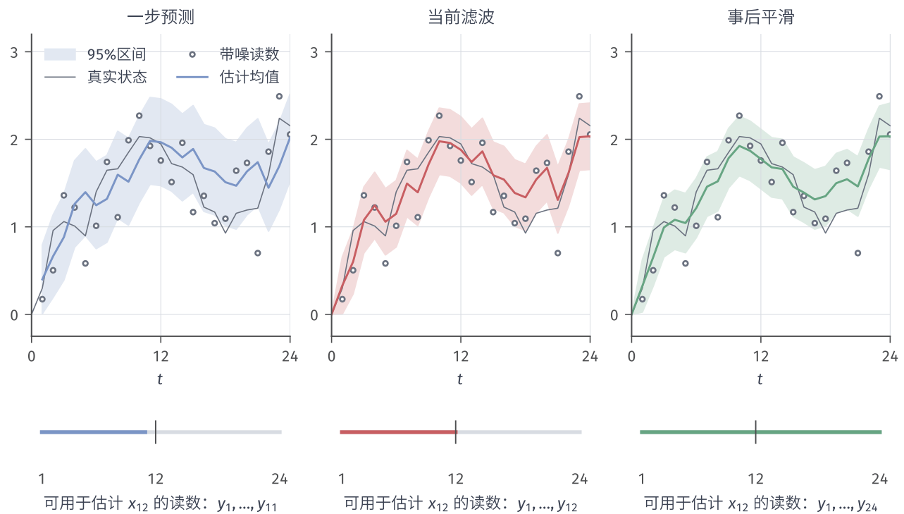
图 13.9 与图 13.5 完全相同的温度轨迹及读数。三栏分别画一步预测、滤波与固定终点 T = 24 的平滑均值和逐时刻 95% 高斯区间，灰线为实际状态，圆点为读数；区间不是整条路径同时覆盖的置信带。下方以 t = 12 为例标出可用观测范围。已知 x_0 = 0 ，给定 u_t = 0.4 ，过程、观测方差仍为 0.04, 0.09。平滑的信息优势不是额外的在线能力。
