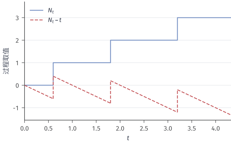
图 10.8 给定三次到达时刻的教学路径, 取 \lambda = 1 。蓝线为计数 N_t , 红虚线为 \tilde{N}_t = N_t - t ; 两条路径在同一时刻跳跃且跳跃量相同。减去的是平均趋势, 不是实现中的跳跃。
