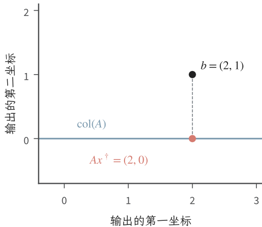
输出空间：最小残差已固定
