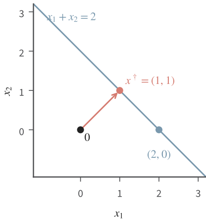
参数空间：选择最小范数
