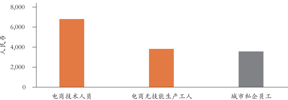
图 5.27. 员工的月平均工资
