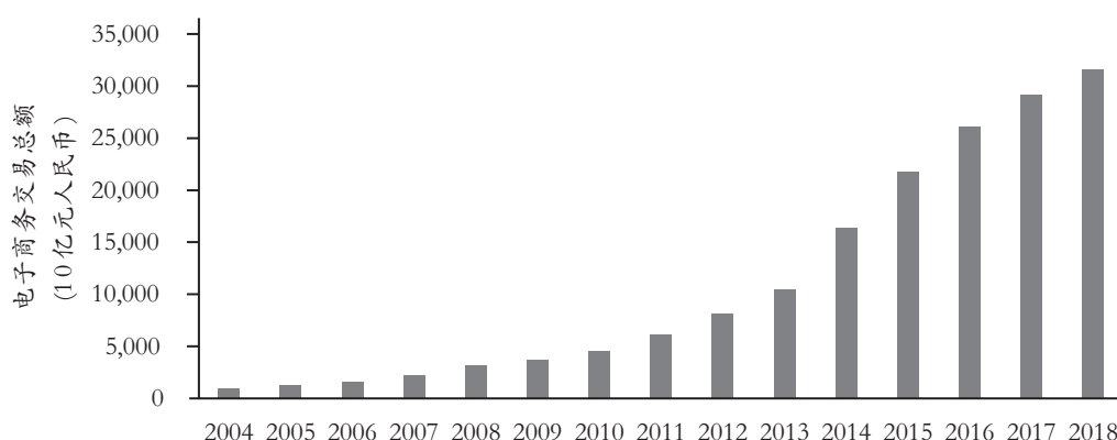
图 1.3. 中国电子商务交易总额
