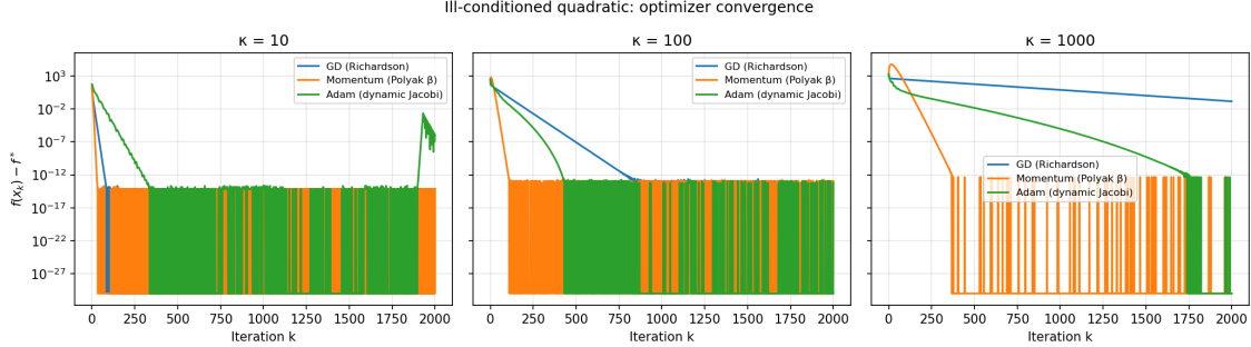
图 4: \kappa \in \{10, 100, 1000\} 下 GD / Heavy-ball / Adam 收敛曲线（实验 1）
