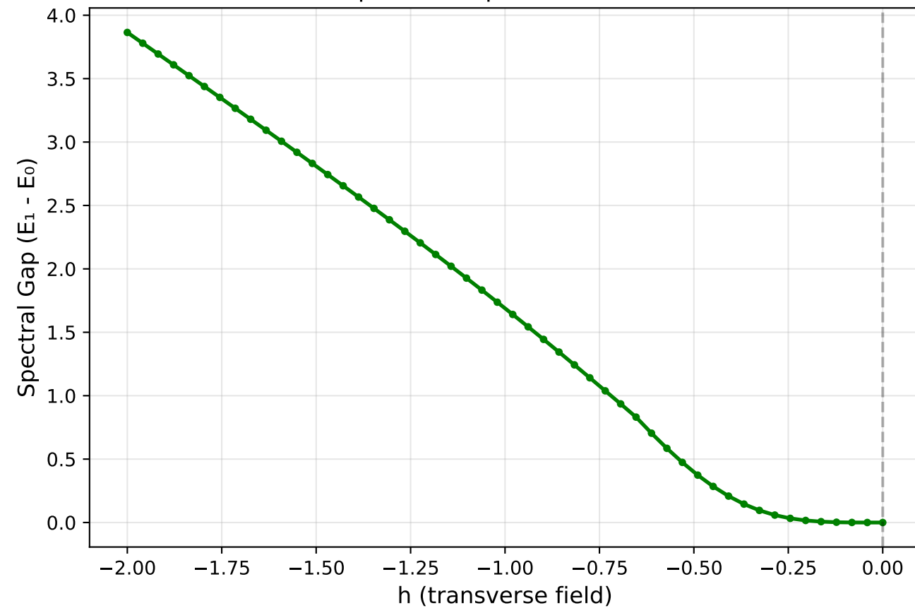
Spectral Gap (linear scale)
