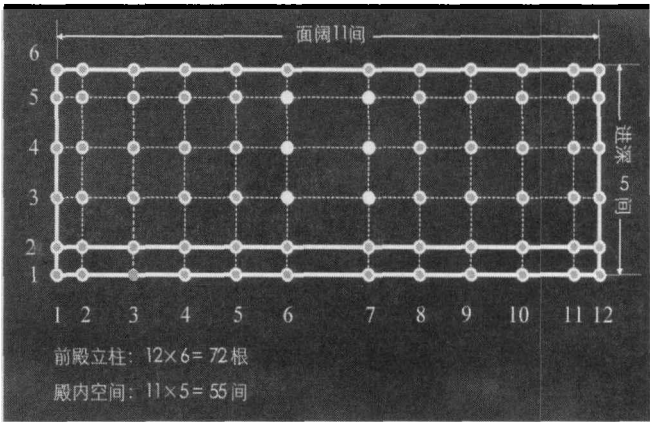
(图4) 北京故宫太和殿的建筑平面结构示意图
