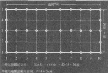
（图7）乾隆年间北京太庙建筑结构改制後中殿与後殿的建筑平面结构示意图
