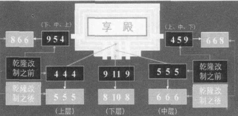
（图8）清代乾隆年间北京太庙前殿台阶改制前後 的比较示意图
