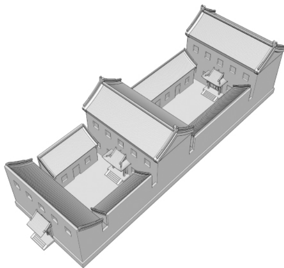
图九 “里五外三穿心楼”的布局形态示意图
