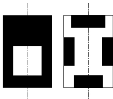
图六 江南毗连型 天井布局庭院与北方分离型庭院比较
