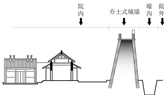
图一四 夯土砖砌城墙剖面示意图
