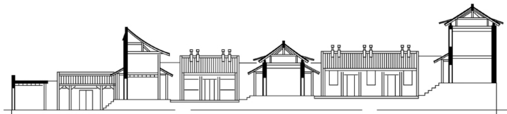
图一〇 乔家大院2号院剖面图
