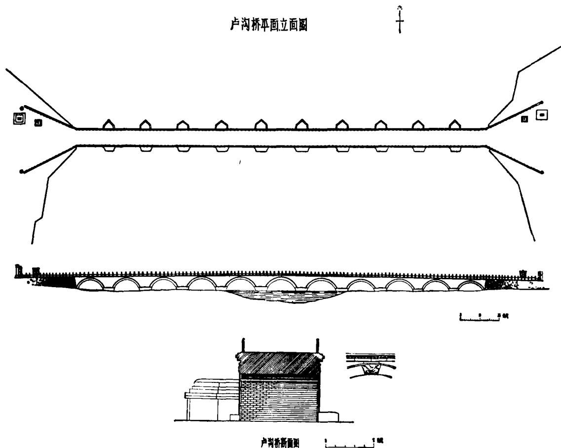
图一 卢沟桥平面、立面、断面图
