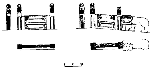
图五 石栏干细部图
