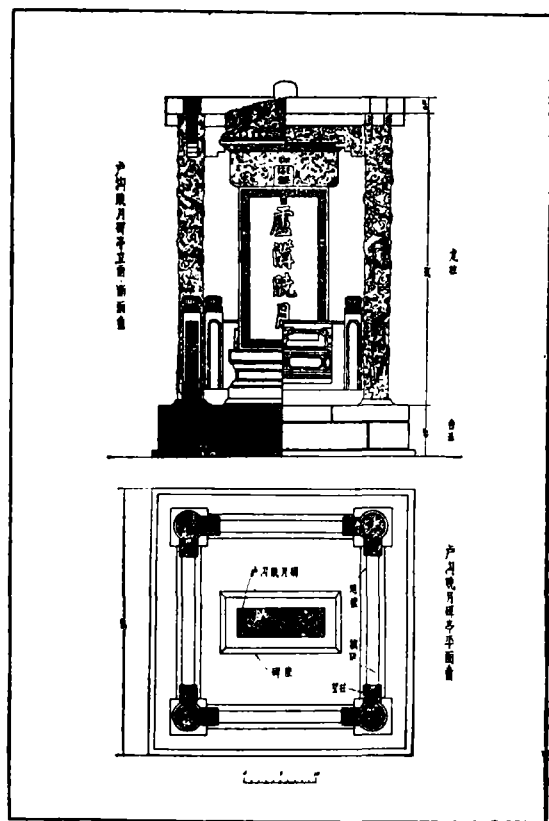
图七 “卢沟晓月”碑亭立面、断面、平面图
