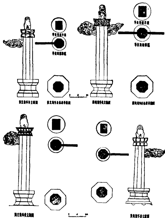
图六 华表立面、平面图
