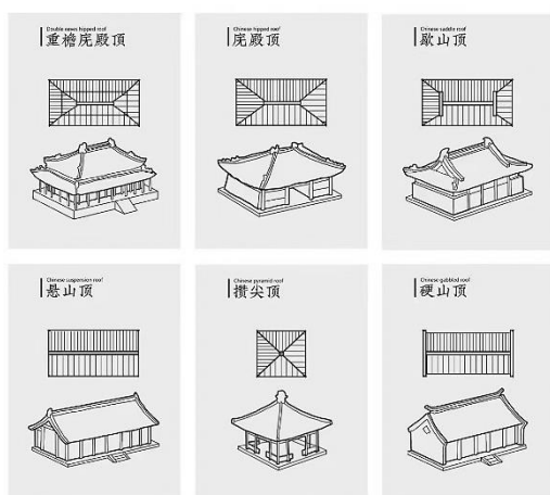
图1-6 常见屋顶样式(图源于网络)
