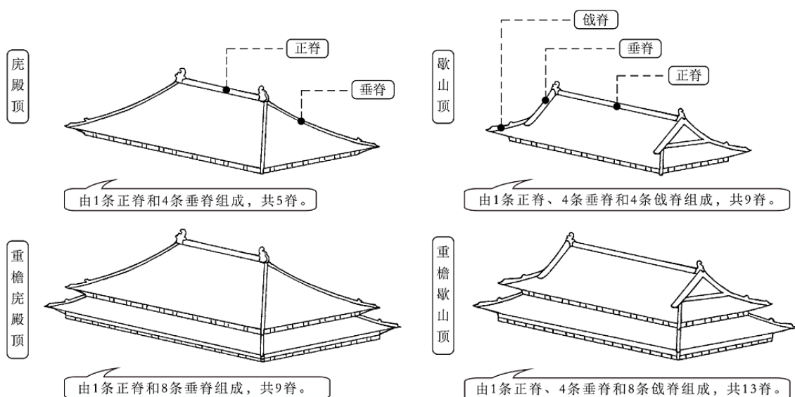
图 4-10 屋顶结构及屋脊（笔者绘制）
