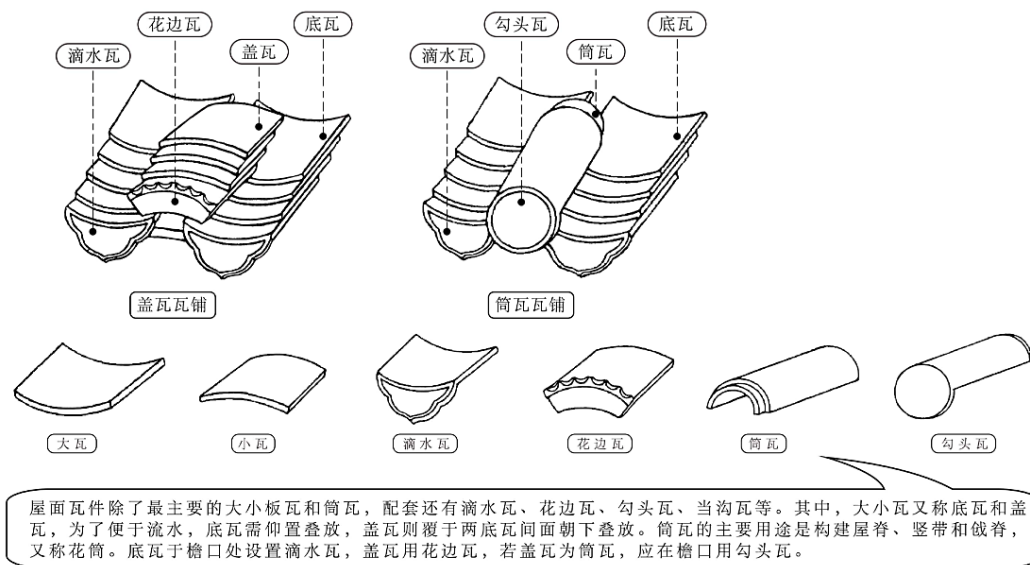
图 4-12 瓦铺结构图（笔者绘制）
