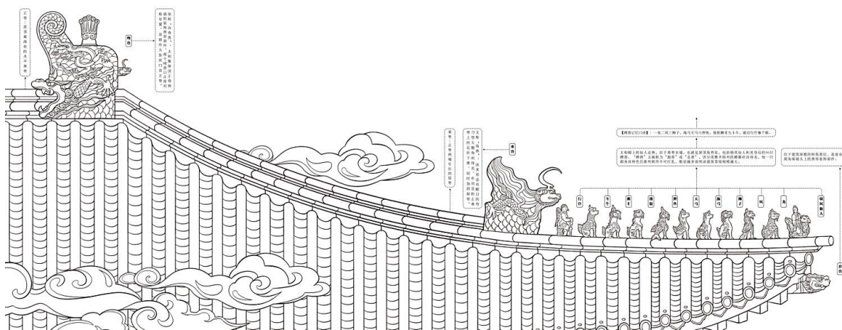
图4-22 太和殿屋脊局部提炼（笔者绘制）
