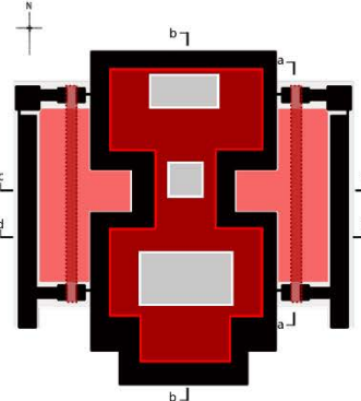
(e) 洞口空间平面
