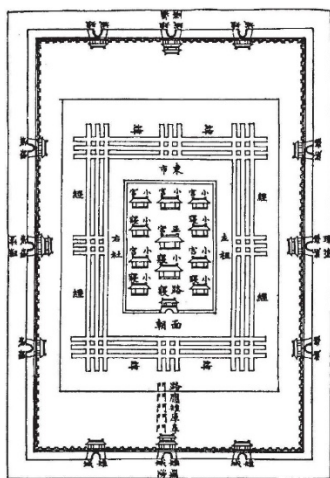
图 3.3 《考工记》中理想周王都平面图 (图片来源:《周礼·考工记》)
