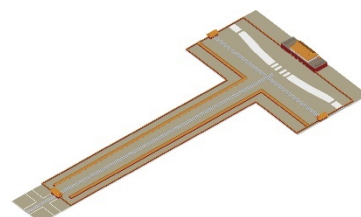
(c) 材质模型空间轴测
