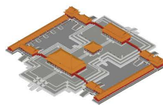
(c) 材质模型空间轴测
