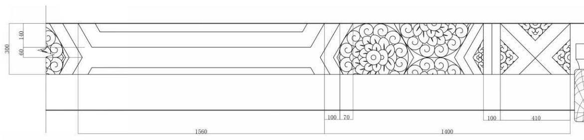
图 4-29 燕喜堂东次间西缝四架梁线图（图片来源：作者绘制）
