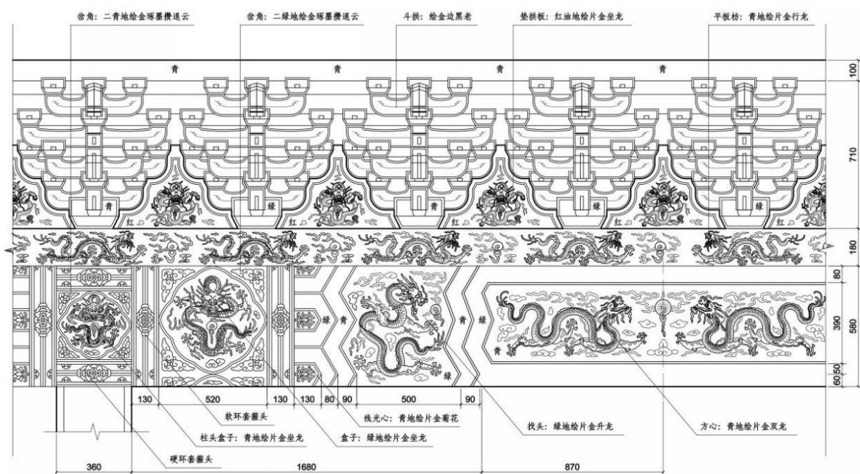
图 4-22 养心殿正殿前檐明间后檐中开间彩画线图 (图片来源: 高业京绘制)
