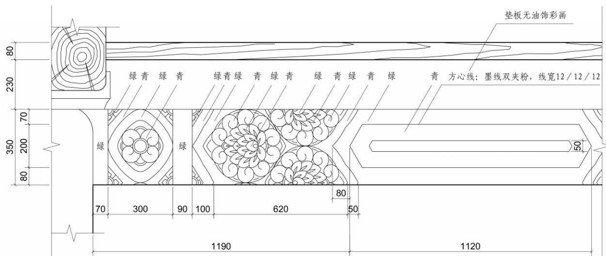
图 4-27 养心殿西配殿明间后檐额枋彩画线图（图片来源：高业京绘制）
