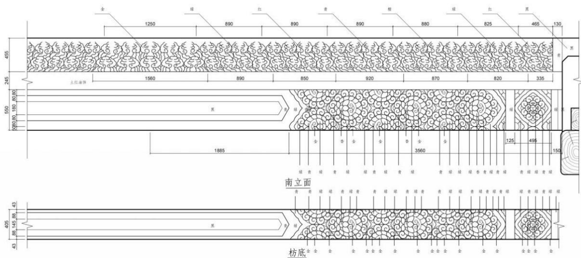
图 4-23 养心殿正殿明间脊檩枋南立面彩画线图（图片来源：高业京绘制）
