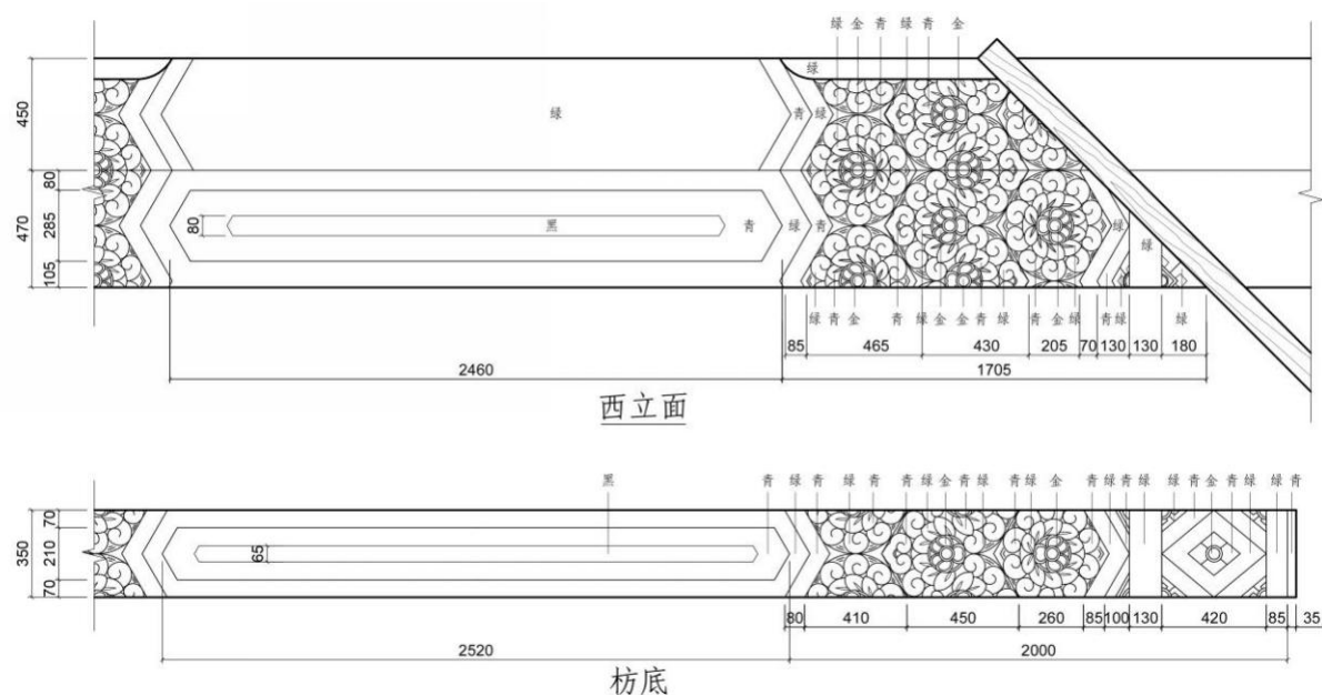
图 4-24 养心殿东暖阁东缝彩画线图（图片来源：高业京绘制）
