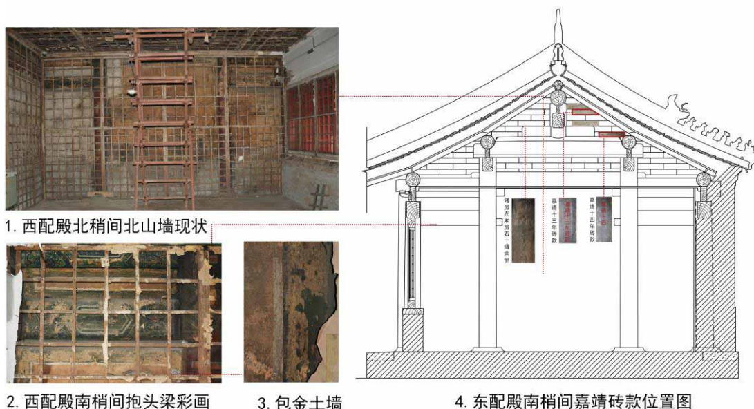
图 3-25 东西配殿内檐彩画（图片来源：作者拍摄、绘制）
