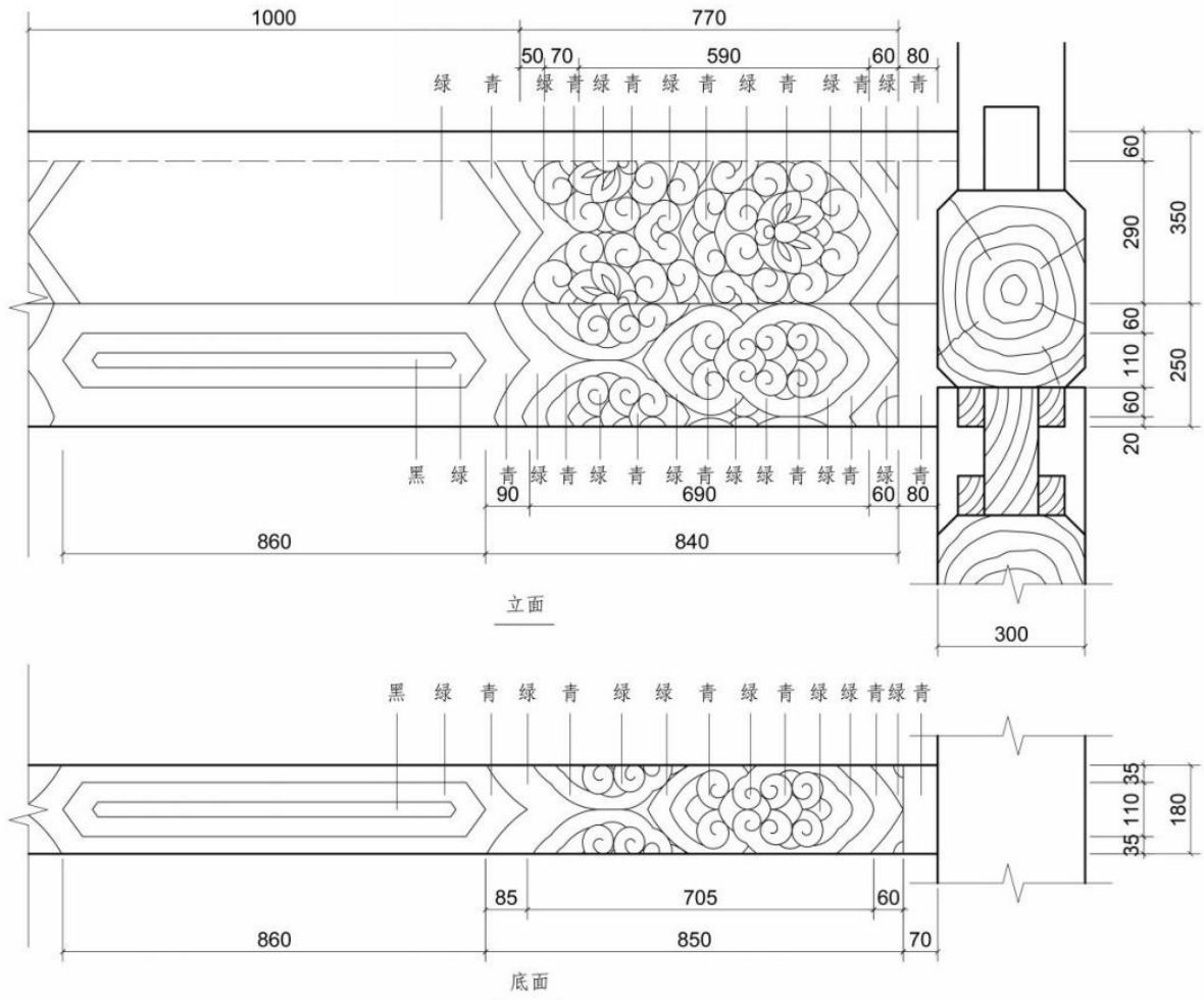
图 4-37 燕喜堂西围房南数第六间前檐上金步内侧彩画线图（图片来源：高业京绘制）
