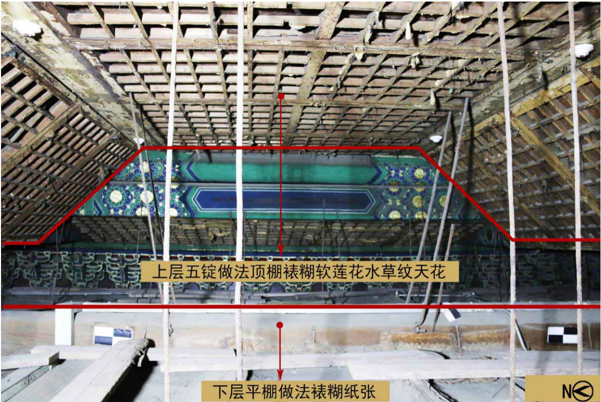
图 3-2 东暖阁五锭做法顶棚（图片来源：作者拍摄、绘制）
