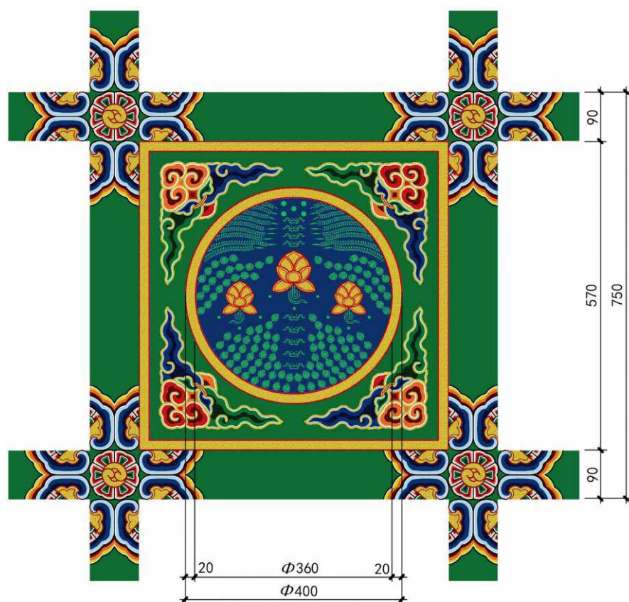
图 4-55 养心殿东西暖阁莲花水草纹天花复原图（图片来源：高业京绘制）
