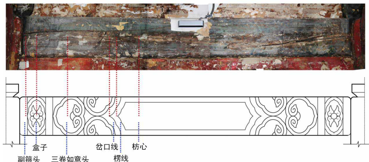
图 3-13 燕喜堂东次间前檐额枋彩画（图片来源：作者拍摄、绘制）
