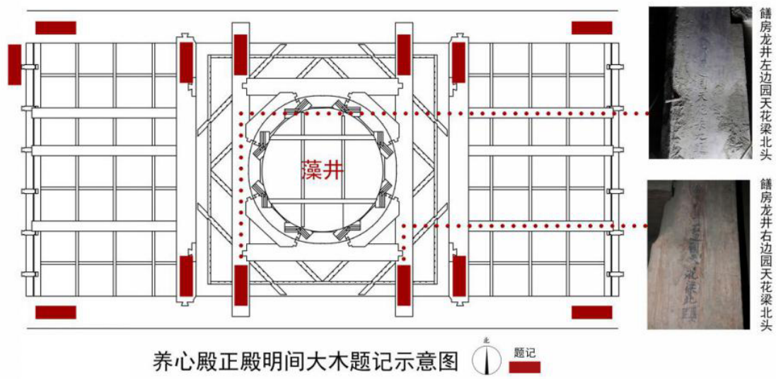
图 3-15 养心殿正殿井口天花以上大木题记（图片来源：作者拍摄、绘制，底图天津大学绘制）
