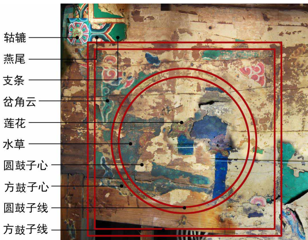
图 4-52 养心殿东西暖阁莲花水草纹天花彩画纹饰图案 (图片来源: 作者拍摄、绘制)
