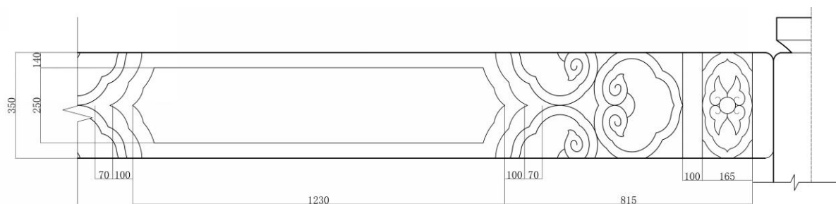
图 4-28 燕喜堂东次间前檐额枋线图（图片来源：作者绘制）
