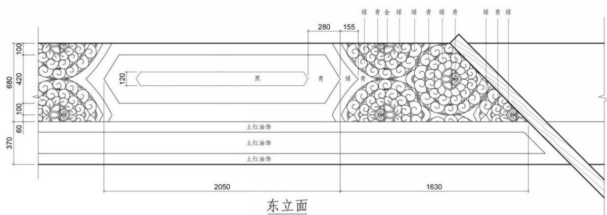
图 4-25 养心殿西暖阁东缝彩画线图（图片来源：高业京绘制）
