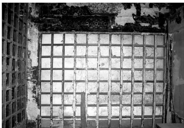
图8 寿康宫北围房后接小房西墙的白槿算子
