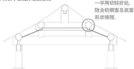
图2 真枋子三锭作法剖面图
