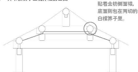
图3 一捧书假枋子三锭作法剖面图
