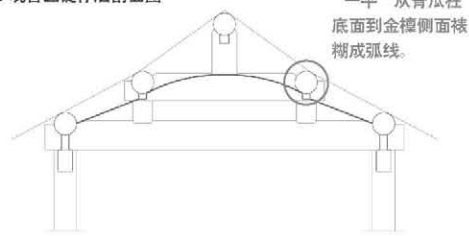
图6 观音三锭作法剖面图
