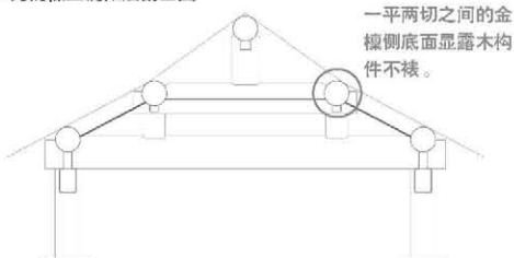
图7 光棍檩三锭做法剖面图
