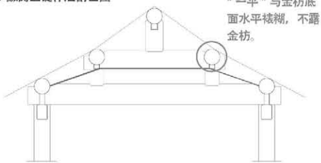
图5 搬窝三锭作法剖面图
