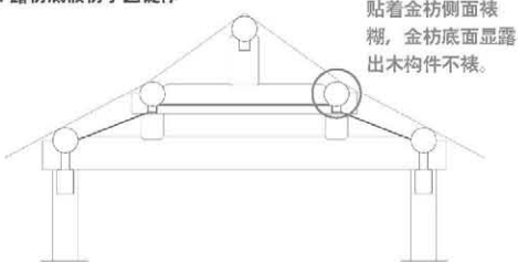
图4 露枋底假枋子三锭作
