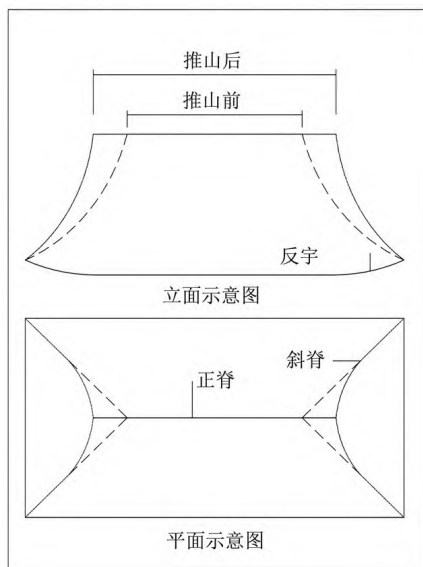
图2 乾清宫庀殿屋顶
