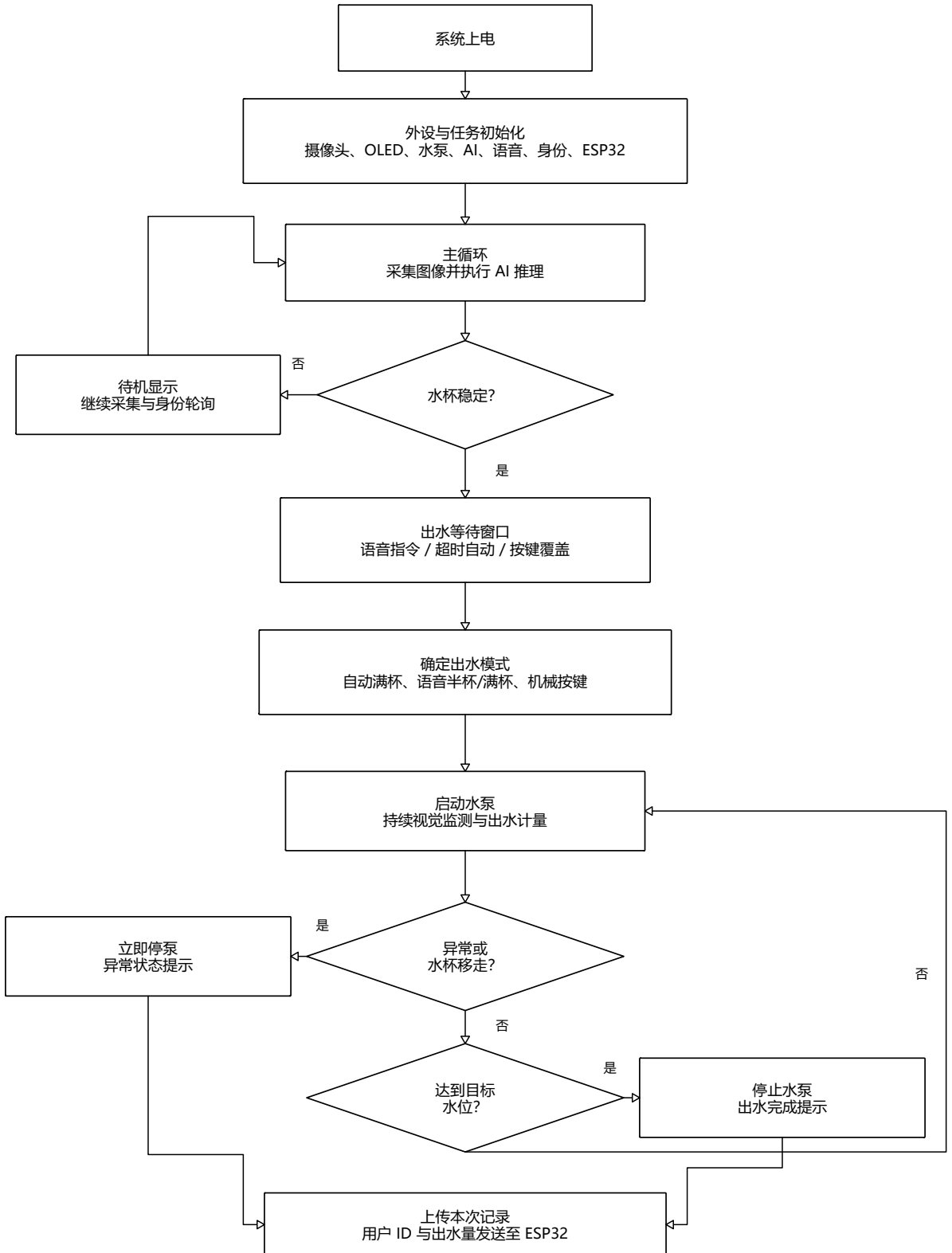
图 X 主控软件流程。身份识别仅作为用户信息补充，不阻塞出水控制；异常保护与目标水位判断由 STM32H7 本地闭环完成。
