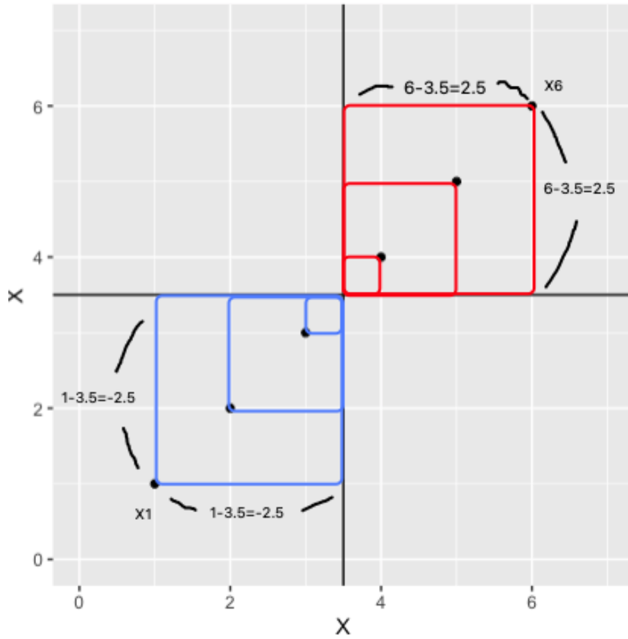
그림 7.1: X의 분산
