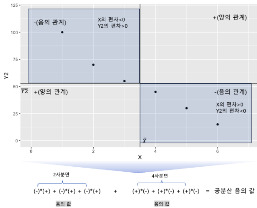
그림 7.3: 음의 공분산
