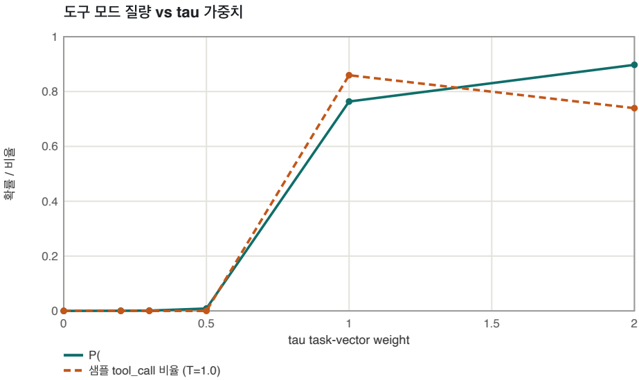
그림 5. tau task-vector 가중치 vs 도구 모드 질량· \tau^2 (학습 전 merge init)
