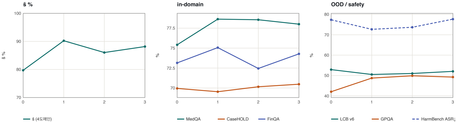
그림 4. 늦은 재-merge ablation — ck200 → +0.3· \tau_{med} → MOPD 25 → 50
