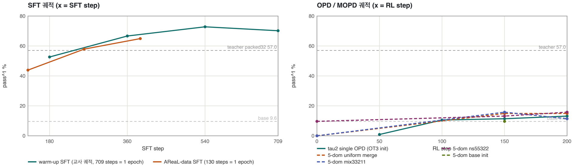
그림 3. \tau^2 telecom — warm-up SFT vs OPD vs 5-dom MOPD
