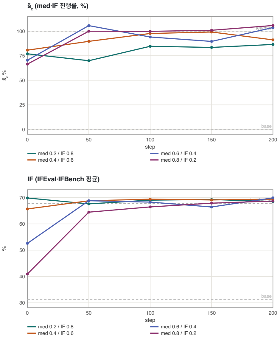
그림 1. 2-dom med+IF grid — merge init(step 0)부터 ck200까지
