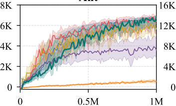
Ant
