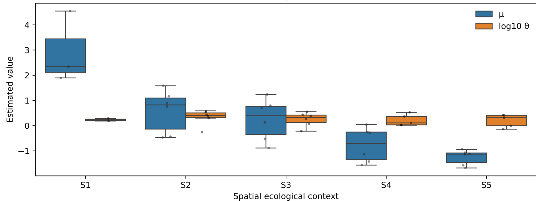
Context-level OU-like parameter summaries
