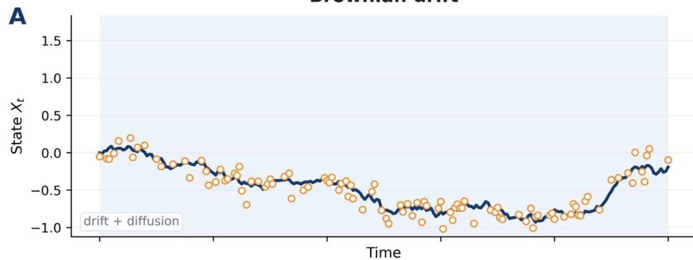
Brownian drift
