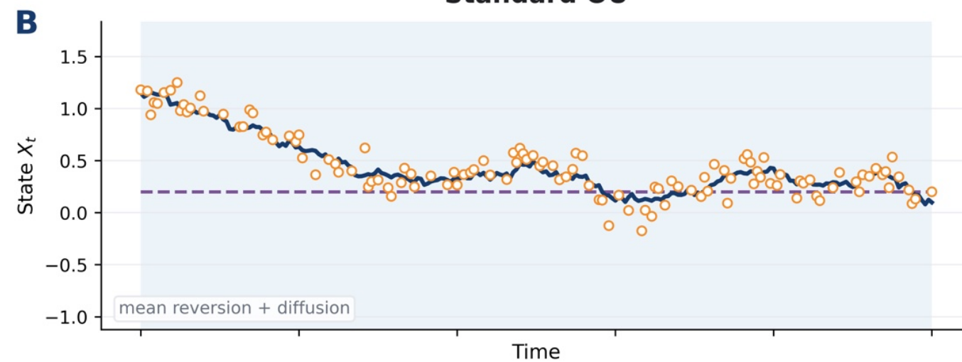
Standard OU
