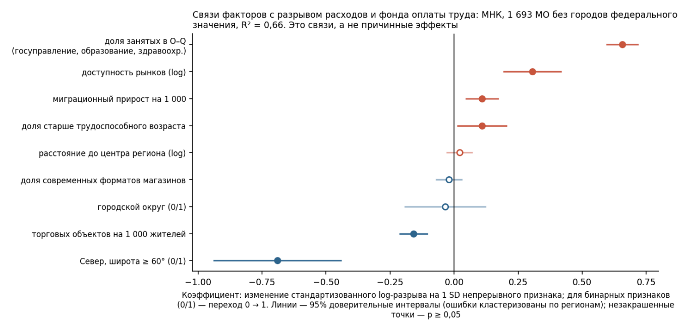
Рис. 2. Модель разрыва: коэффициенты и 95%-ные доверительные интервалы
