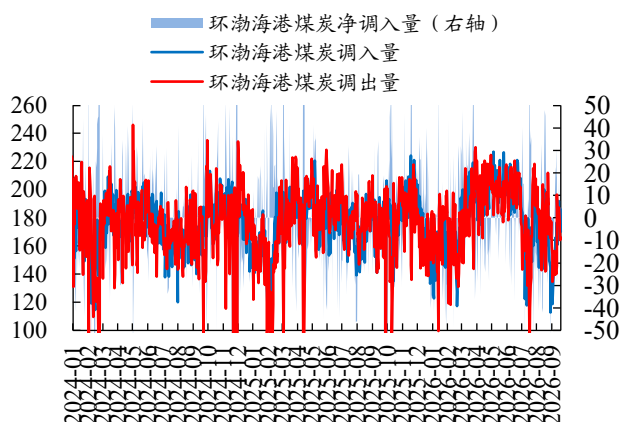
图30: 本周环渤海港口煤炭净调入(万吨)
