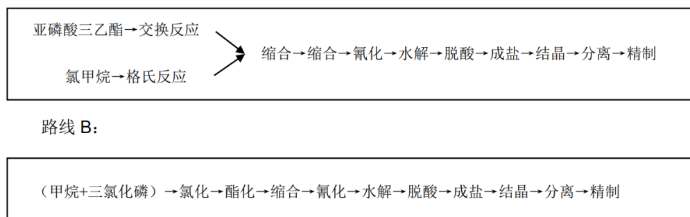
图3：草铵膦生产工艺：主要涉及亚磷酸三乙酯、三氯化磷等重要原材料
