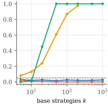
(d) DSR certifies, \rho = 0.6
