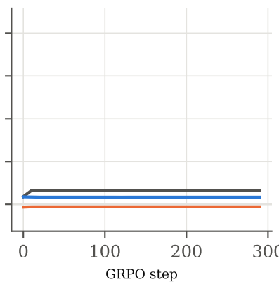
actual, train
