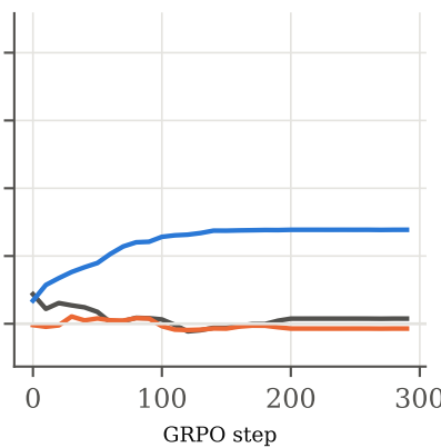
actual, val
