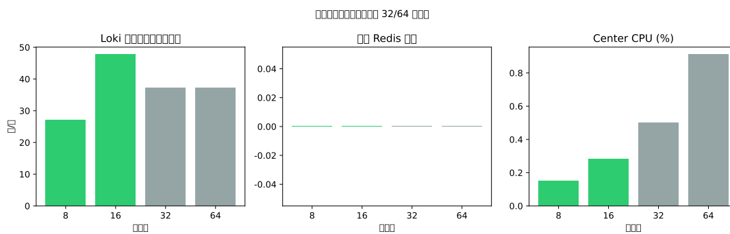
图 7: 多规模扩展实验 (绿: 实测 8/16 节点; 灰: 32/64 外推)
