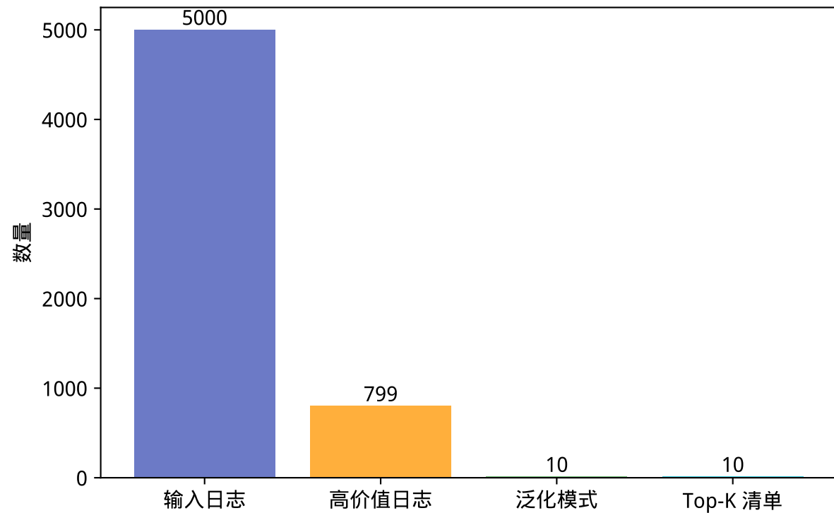
图6 关注清单生成算法微基准 (耗时 0.5 ms)
