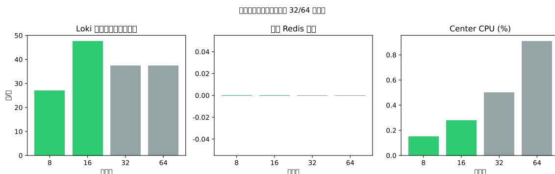
图 7: 多规模扩展实验（绿色/实线：8/16 节点集群实测；灰色/虚线：32/64 节点线性外推，非实测）
