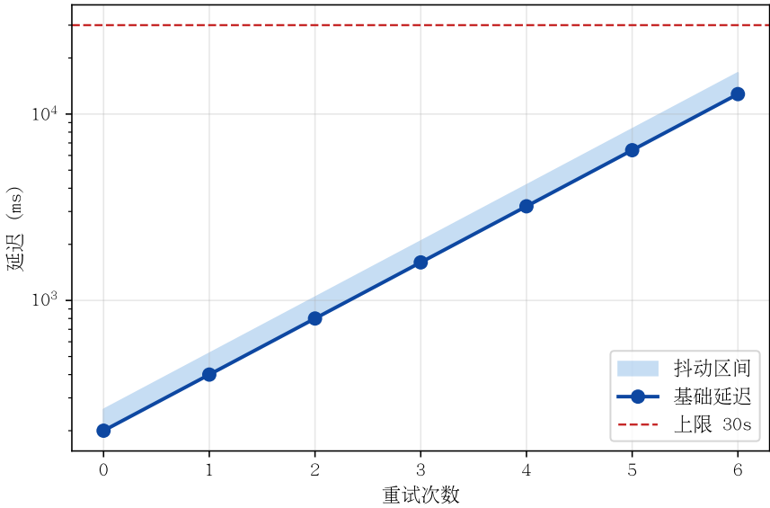
图 3 指数退避重试延迟分布
