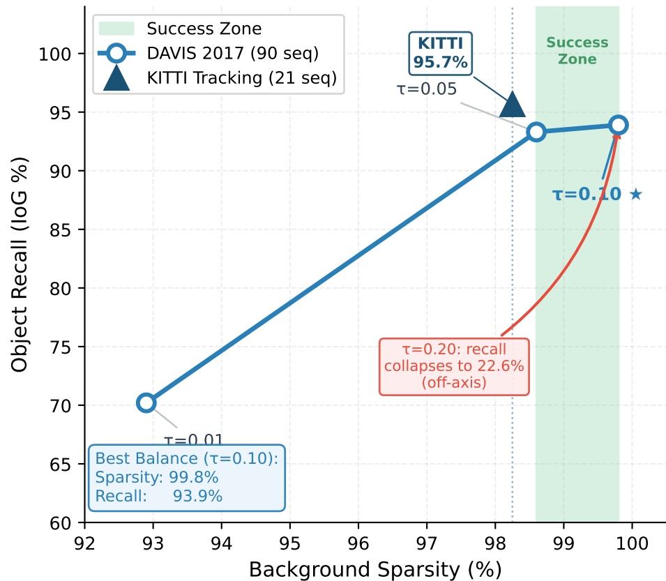
Sparsity-Recall Pareto Frontier
