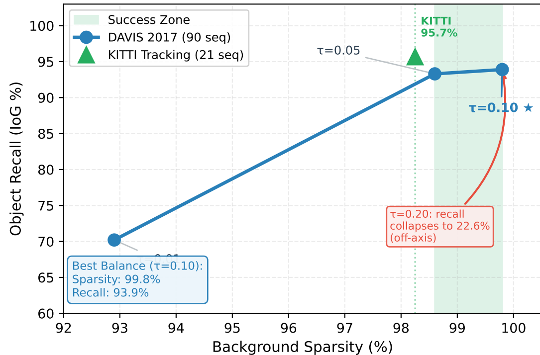
Sparsity-Recall Pareto Frontier
