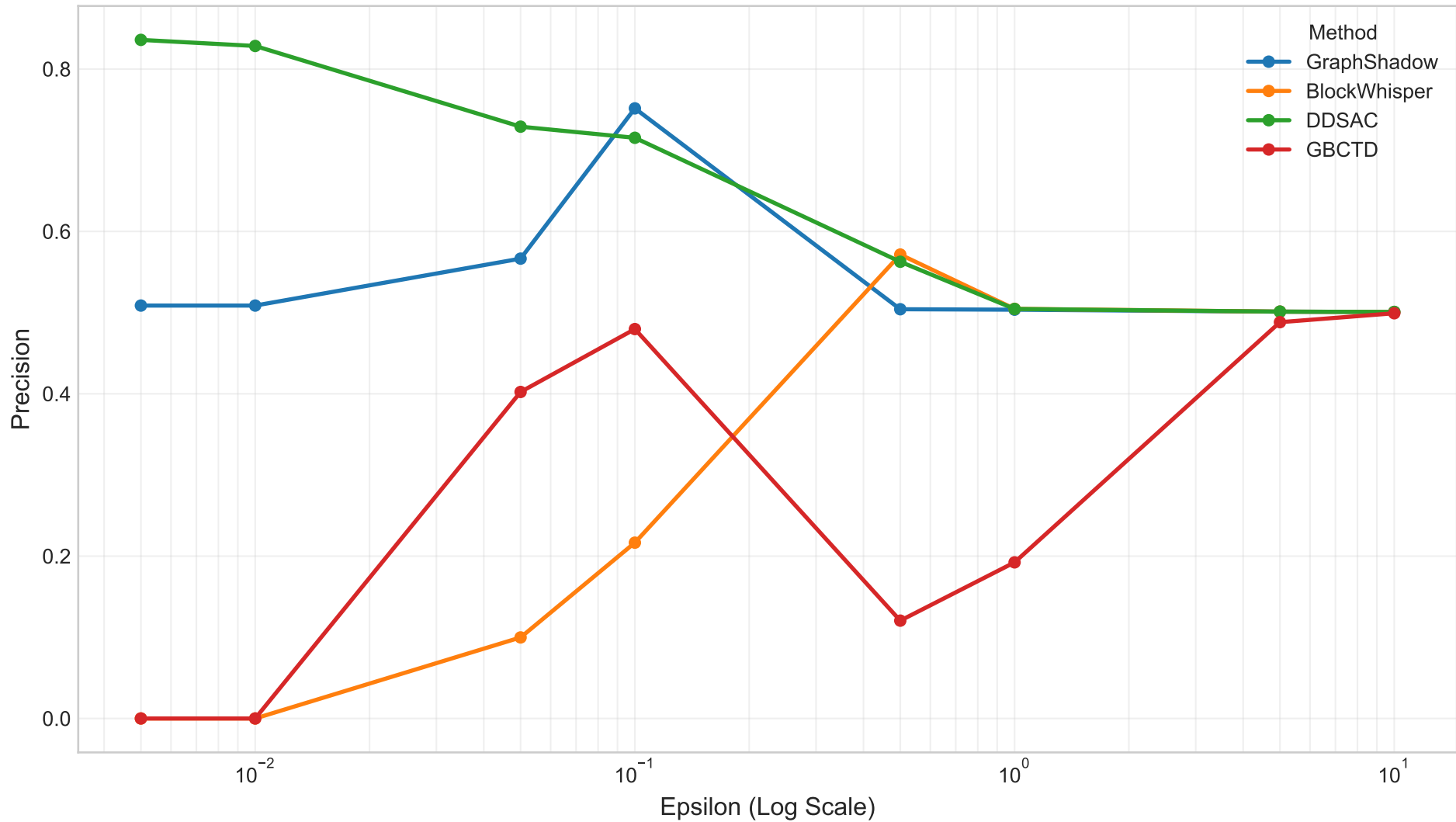
Precision vs Epsilon (Fixed Quota)
